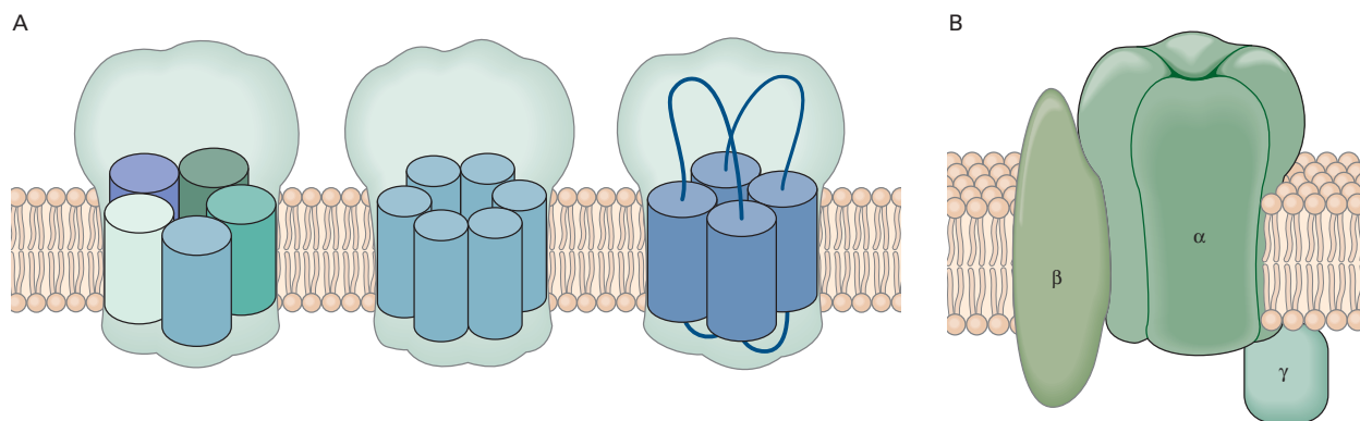
图 8.3.1: 离子通道是由多个亚基组成的完整膜蛋白。A. 离子通道可以构建为来自不同亚基的异源寡聚体（左），作为来自单一类型亚基的同源寡聚体（中间），或者来自组织成重复基序的单个多肽链，其中每个基序的功能相当于一个亚基（右）。B. 除了形成中心孔的一个或多个 \alpha 亚基外，一些通道还包含调节孔门控、通道表达和膜定位的辅助亚基（ \beta 或 \gamma ）。
