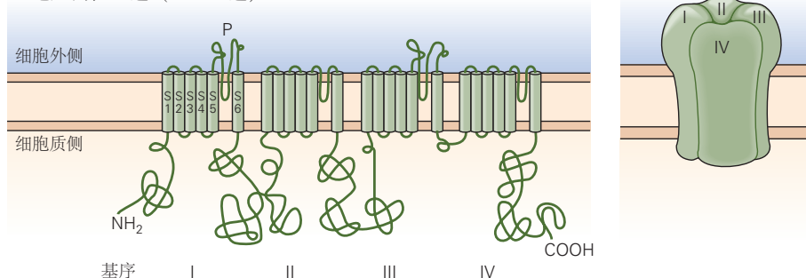
图 8.3.3: 离子通道的 3 个超家族。A. 配体门控通道大家族的成员，例如乙酰胆碱受体通道，由 5 个相同或密切相关的亚基组成，每个亚基包含 4 个跨膜 \alpha -螺旋（M1-M4）。图中的每个圆柱体代表一个跨膜 \alpha -螺旋。B. 间隙连接通道由一对半通道形成，突触前和突触后细胞膜各有一个，连接在 2 个细胞之间的空间中。每个半通道由 6 个相同的亚基组成，每个亚基包含 4 个跨膜 \alpha -螺旋。间隙连接通道充当电突触中突触前和突触后细胞的细胞质之间的管道（第 11 章）。C. 电压门控 Na + 通道由一条多肽链形成，该多肽链包含 4 个同源结构域或重复序列（基序 I-IV），每个具有 6 个跨膜 \alpha -螺旋（S1-S6）。S5 和 S6 区段由一条延伸的氨基酸链连接（即 P 区），它浸入和浸出膜的外表面，形成孔的选择性过滤器。电压门控 Ca 2+ 通道具有相同的一般结构模式，尽管氨基酸序列不同。
