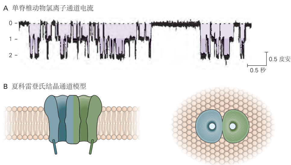
图 8.3.8: Cl^- 通道和转运蛋白的脊椎动物夏科雷登氏结晶家族是具有 2 个相同孔的双桶通道。A. 通过单个脊椎动物 Cl^- 通道的电流记录显示 3 个级别的电流: 2 个孔都关闭 (0)、1 个孔打开 (1), 2 个孔都打开 (2)。B. 从侧面 (左) 显示通道并从细胞外向下看膜 (右)。每个亚基都包含自己的离子传输通路和门。此外, 二聚体有 1 个由 2 个亚基共享的门 (未显示)。
