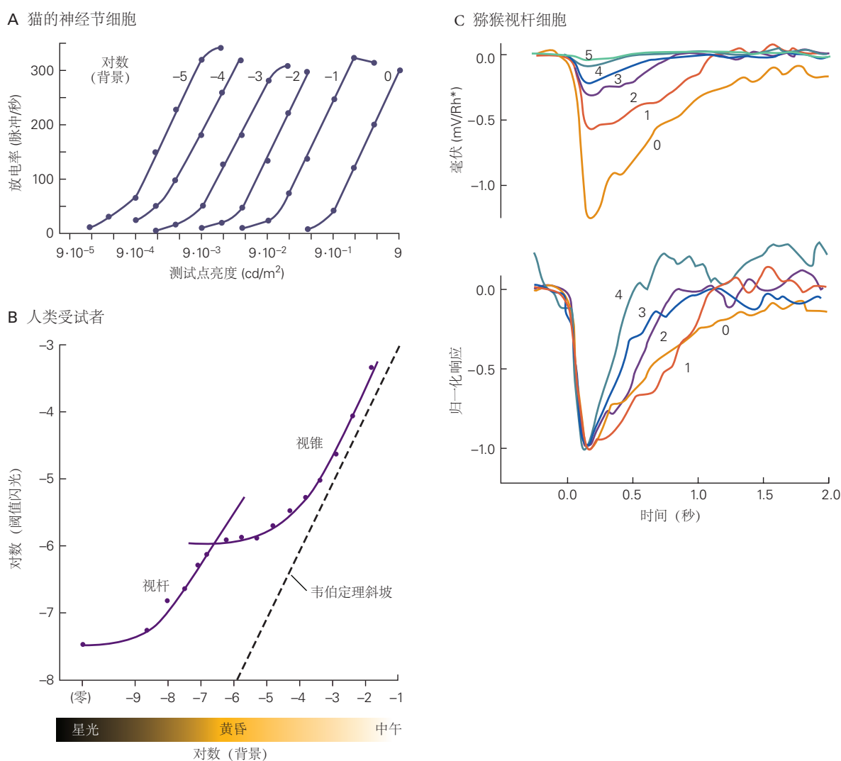
图 22.5.2: 光照适应。 A. 猫视网膜神经节细胞的感受野在稳定的背景强度下均匀照明, 并在感受野中心短暂闪烁一个测试点。测量闪光后的峰值激活率并根据闪光强度的对数绘制。每条曲线对应不同的背景强度, 从左到右增加 10 倍 [199] 。 B. 一个小的测试点在稳定照明的背景上短暂闪光, 闪光强度逐渐增加到人类受试者刚好可以检测到的程度。在不同的背景强度下重复该过程。这里, 阈值闪光强度根据背景强度绘制。该曲线有 2 个分支, 由一个明显的扭结相连: 它们对应于视杆视觉和视锥视觉的状态。当阈值强度与背景强度成正比时, 韦伯定律的斜率表示理想化 [200] 。 C. 上图显示了猕猴视杆细胞对不同背景强度下出现闪光的响应。细胞的单光子响应根据记录的膜电位除以闪光激活的视紫红质的数量计算得出。单光子响应的增益随着背景强度的增加而显著降低。背景强度 (以光子/平方微米/秒为单位) 对于迹线 0 为 0, 对于迹线 1 为 3.1, 对于迹线 2 为 12, 对于迹线 3 为 41, 对于迹线 4 为 84, 对于迹线 5 为 162。在底部图中, 相同数据 (最小响应除外) 被归一化为相同的振幅, 表明单光子响应的时间进程在高强度下加速 [201] 。
