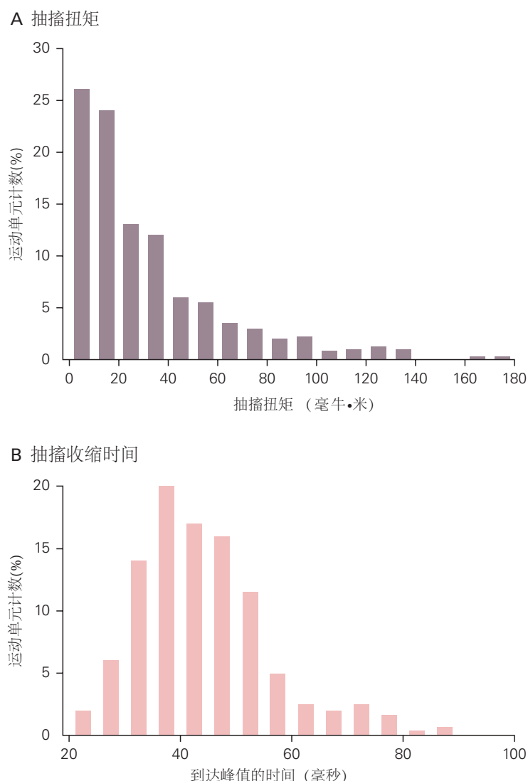
图 31.1.3: 大多数人体运动单元产生的力小，收缩时间中等 [281] 。A. 从 10 名受试者获得的胫骨前肌中 528 个运动单元的抽搐扭矩分布。B. 胫骨前肌 528 个运动单元的抽搐收缩时间分布。
