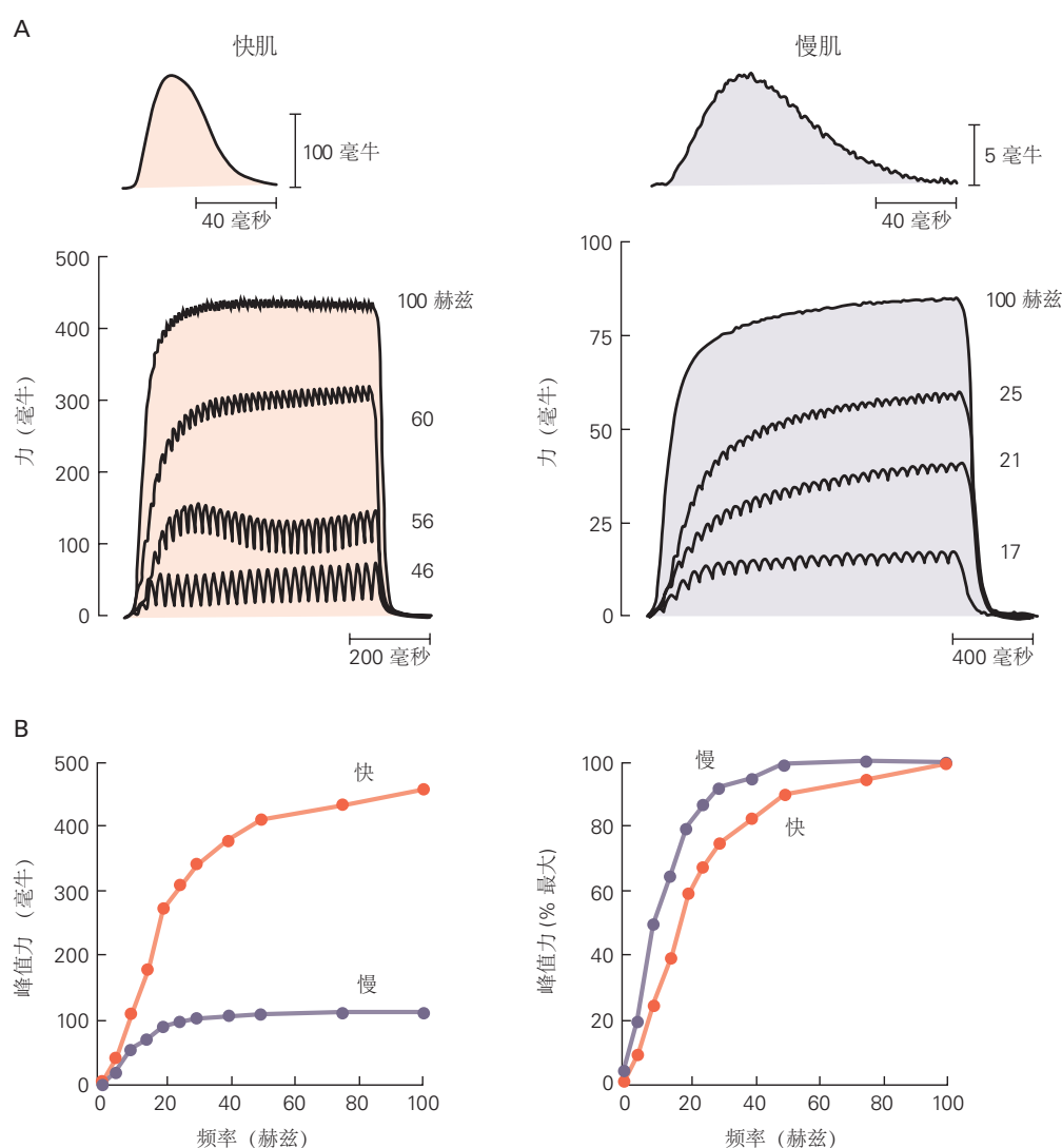
图 31.1.2: 运动单元施加的力随其神经元产生动作电位的速率而变化。A. 轨迹显示快速和慢速收缩运动单元响应单个动作电位（顶部轨迹）和一系列动作电位（下面的 4 个轨迹组）所施加的力。速度更快的单元达到峰值抽搐力或收缩时间的时间更短。用于引起强直性收缩的动作电位的速率范围从慢速收缩单元中的 17 到 100 赫兹到快速收缩单元中的 46 到 100 赫兹。由 100 赫兹刺激引起的强直力峰值对于快速收缩单元来说更大。注意 2 组迹线的不同力标度 [278-280] 。B. 快速收缩和慢速收缩运动单元的峰值力和动作电位之间的关系。在所有频率下，快速收缩的运动单元的绝对力（左图）都更大。在较低的刺激率下（右图），与快速收缩的运动单元（较短的收缩时间）相比，慢速收缩的运动单元（较长的收缩时间）产生的相对力（峰值力的百分比）更大。
