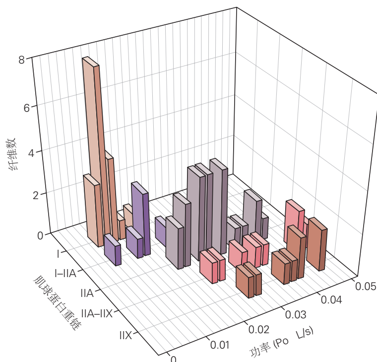
图 31.1.4: 肌纤维类型的收缩特性是连续分布的。具有不同类型肌球蛋白重链亚型的股外侧肌单肌纤维片段产生的峰值功率。2 种类型的混合纤维（I-IIA 和 IIA-IIX）包含 2 种类型的肌球蛋白重链的亚型。功率计算为峰值强直力 ( P_o ) 和最大缩短速度（每秒段长度 [L/s]）的乘积 [282] 。
