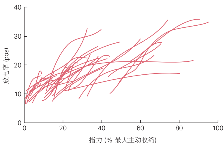
图 31.1.7: 可以通过改变活动运动单元的数量及其放电率来调节肌肉力量。每条线显示手部肌肉中单个运动单元在一系列手指力（最大主动收缩）下的放电率（每秒脉冲数）。手指力是由单手肌肉的作用产生的。每条线最左边的点表示运动单元被募集的阈值力，而最右边的点对应于可以识别运动单元的峰值力。对于募集阈值较低的运动单元，放电率的范围通常较小。手指力的增加是由同时增加的放电率和激活的运动单元的数量产生的 [285] 。
