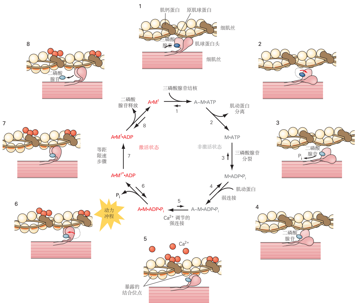
图 31.2.2: 跨桥循环。 几个非激活状态之后是几个由 Ca^{2+} 触发的激活状态。该循环从顶部（步骤 1）开始，三磷酸腺苷与肌球蛋白头部结合。肌球蛋白头与肌动蛋白分离（第 2 步），三磷酸腺苷被切割成磷酸盐 ( P_i ) 和二磷酸腺苷（第 3 步），肌球蛋白与肌动蛋白弱结合（第 4 步）。 Ca^{2+} 与肌钙蛋白的结合导致原肌球蛋白滑过肌动蛋白并使 2 个肌球蛋白头部闭合（第 5 步）。这导致 P_i 的释放和肌球蛋白颈部的延伸，即跨桥循环的动力冲程（步骤 6）。在结构变化（步骤 7）和二磷酸腺苷释放（步骤 8）期间，每个横桥施加大约 2 pN 的力（•，强结合；，弱结合；Mf，肌球蛋白的跨桥力；和 Mf*，肌球蛋白的受力状态） [289] 。
