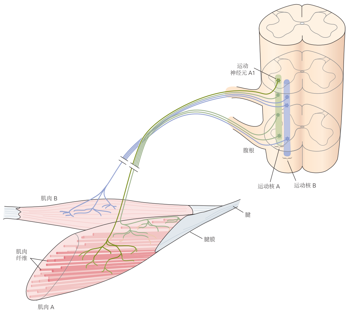
图 31.1.1: 典型的肌肉由数千条并行工作的肌纤维组成，并组织成数量较少的运动单元。一个运动单元包括一个运动神经元和它支配的肌肉纤维，此处用运动神经元 A1 表示。支配一块肌肉的运动神经元通常聚集成一个细长的运动核，该核可能在腹侧脊髓内延伸 1 个到 4 个节段。来自运动核的轴突在几个腹根和周围神经中离开脊髓，但聚集在目标肌肉附近形成一个神经束。在图中，运动核 A 包括所有支配肌肉 A 的运动神经元；同样，运动核 B 包括支配肌肉 B 的所有运动神经元。每个运动神经元的广泛分支树突（图中未显示）倾向于与来自其他核的运动神经元的树突混合。
