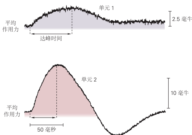
图 31.1.5: 施加较小力量的运动单元先于施加较大力量的运动单元被募集 [283-284] 。A. 当受试者逐渐增加肌肉力量时，用单个肌内电极同时记录 2 个运动单元的动作电位。运动单元 1 在自主收缩开始时开始释放动作电位，并且在收缩期间其放电速率增加。运动单元 2 在收缩接近尾声时开始释放动作电位。B. 在自主收缩期间使用平均程序提取的运动单元 1 和 2 的平均抽搐力。C. 该图显示了一个人的手部肌肉中 64 个运动单元在自主收缩期间被募集的净肌肉力量（募集阈值）相对于各个运动单元的抽搐力。
