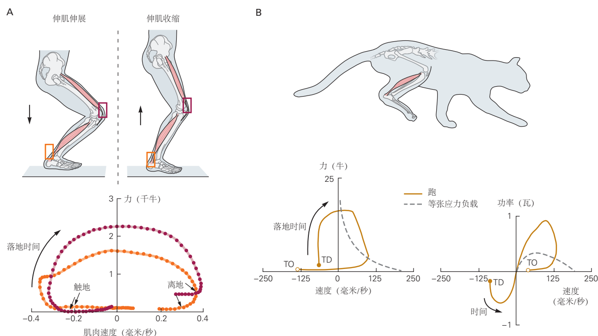
图 31.3.4: 负功的初始阶段会增强肌肉随后执行的正功 [292-293] 。A. 跟腱（橙色）和髌腱（紫色）的力在两足跳跃的触地阶段发生变化。脚在触地时接触地面，在脚趾离地时离开地面。对于运动的大约前半部分，股四头肌和三头肌小腿肌肉拉长，执行负功（负速度）。肌肉在缩短时执行正功（正速度）。力传感器测量的位置由矩形表示。B. 以中速奔跑的猫比目鱼肌施加的力从爪子触地到离地的瞬间发生变化。肌肉在缩短收缩（正速度）期间施加的力大于肌肉在各种恒定负荷（等张负荷）下最大程度收缩时测得的峰值力。负速度反映了比目鱼肌的收缩延长。猫的比目鱼肌在跑步过程中产生的力量大于孤立肌肉实验（虚线）中产生的力量。当肌肉执行负功时，负功率阶段对应于爪子触地后的延长收缩。
