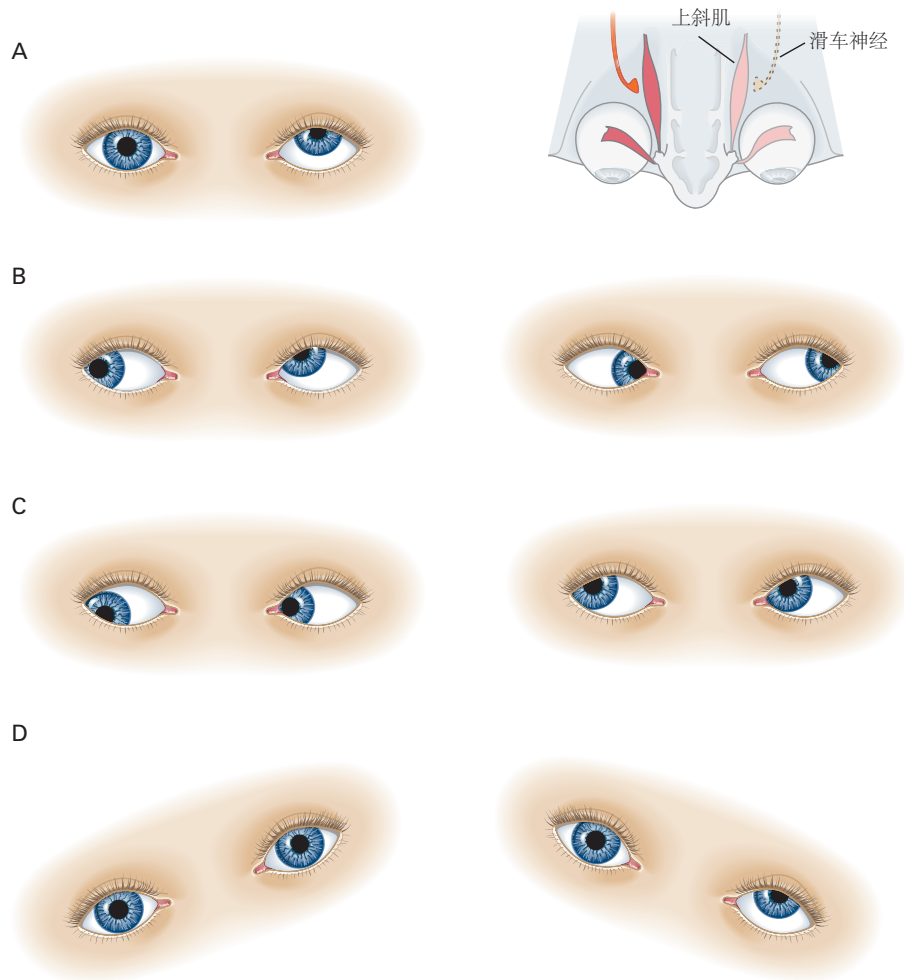
图 35.1.4: 左滑车神经麻痹的疗效。滑车神经支配上斜肌，上斜肌插入眼球赤道后方。当它内收时，它会压低眼睛，当它外转时，它就会内旋眼睛。 A. 斜视是一种眼睛的永久性向上偏斜，当患者直视前方时可以看到。右眼位于眼眶中心，但受影响的左眼略高于右眼。 B. 当眼睛内收时，由于无干扰的下斜肌将眼睛推高（左），因此斜视更严重。当眼睛被诱拐（右）时，情况会得到改善，因为上斜肌对凹陷的贡献小于对内翻的贡献。 C. 当患者向右看时，斜视向下看（左）比向上看（右）更严重。 D. 头向右（左）倾斜可改善高渗，向左（右）倾斜可恶化。眼球反滚动反射引起左眼向左倾斜时的内斜视和眼睛向右倾斜时的外斜视（第 27 章）。头向左倾斜时，内翻需要增加上直肌的活动，上直肌的提升活动不受弱上斜肌的影响，从而导致高斜视增加。随着头部向右倾斜和左眼外展，无对手的上直肌活动减少，斜视减少。
