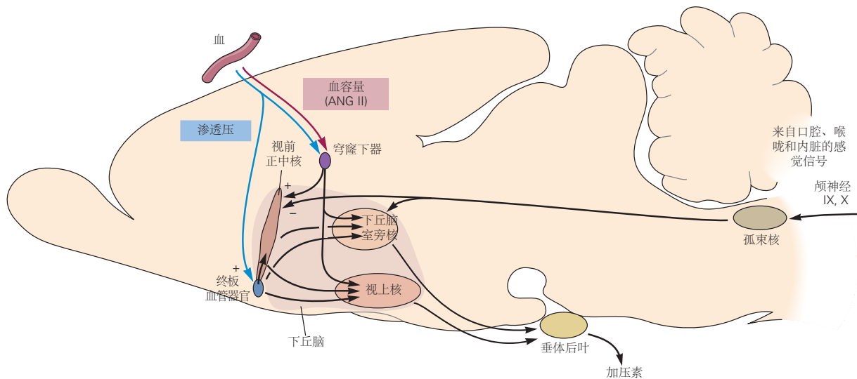
图 41.7.1: 神经和内分泌成分结合起来调节体液平衡。回路显示在大鼠大脑的矢状截面中。来自循环系统中的压力受体和口腔、喉咙和内脏中的感觉受体的信息通过舌咽（IX）和迷走神经（X）神经传递到孤束核和脑干部部的邻近结构。激素血管紧张素 II 为大脑提供有关低血容量的额外信号。循环血管紧张素 II 被穹窿下器中的受体感知；穹窿下器神经元投射到视前正中核、下丘脑室旁核、视上核和终板血管器官。血液的渗透压由投射到视前正中核、下丘脑室旁核和视上核的终板血管器官内和附近的受体感知。下丘脑室旁核和视上核细胞核中的神经分泌细胞触发垂体后叶释放加压素，从而减少肾脏的水排泄 [394] 。
