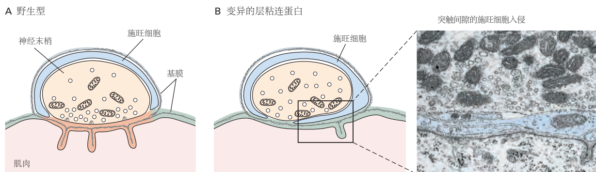
图 48.2.4: 不同的层粘连蛋白亚型位于基底层突触和突触外区域。A. 在基底层的突触（棕色）和突触外（绿色）区域发现了不同的层粘连蛋白亚型。含有 \beta 2 链的异构体集中在突触区域。B. 在缺乏 \beta 2 层粘连蛋白的小鼠中，神经肌肉接头的成熟受损。这些突变体几乎没有活性区，突触间隙被施旺细胞突起（蓝色）侵入 [437] 。
