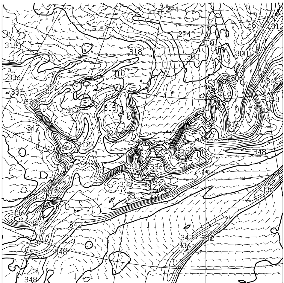
T=48 850hPa: E.P.TEMP(K),WIND(KNOTS) VALID 221200UTC
