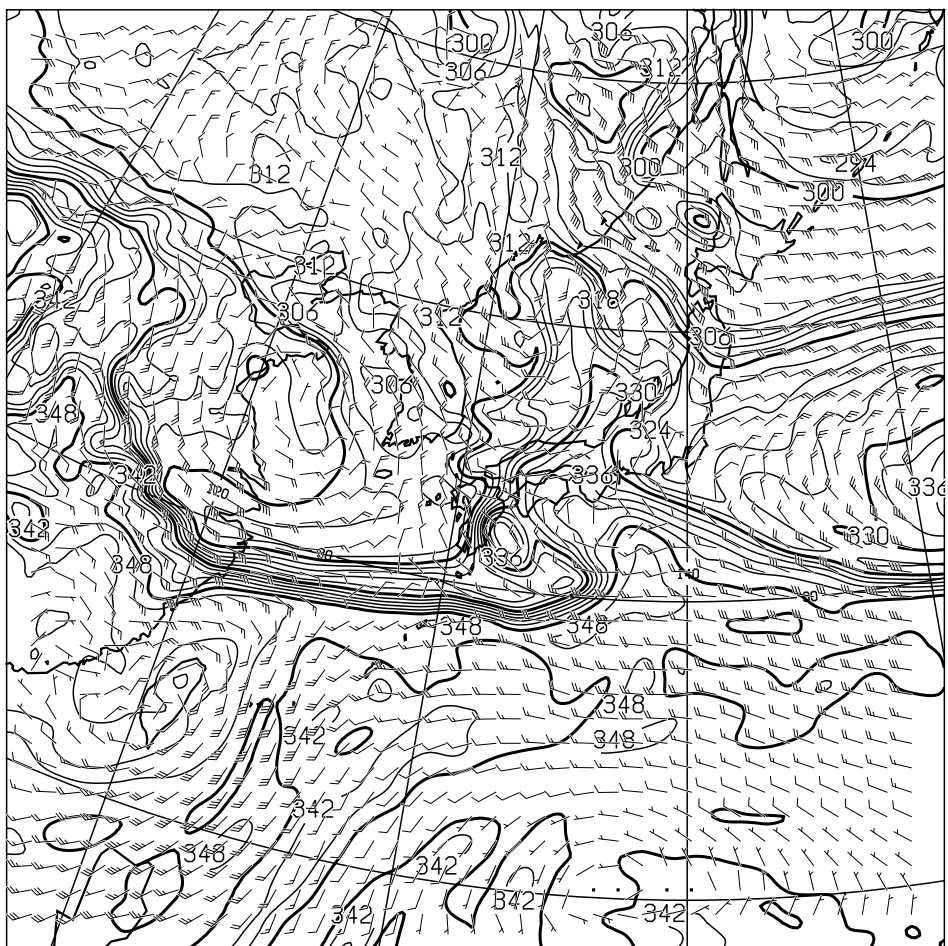
T=48 850hPa: E.P.TEMP(K),WIND(KNOTS) VALID 051200UTC
