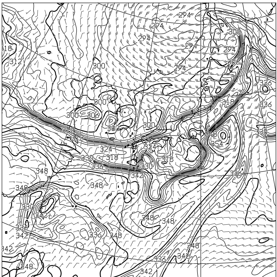
T=48 850hPa: E.P.TEMP(K),WIND(KNOTS) VALID 011200UTC
