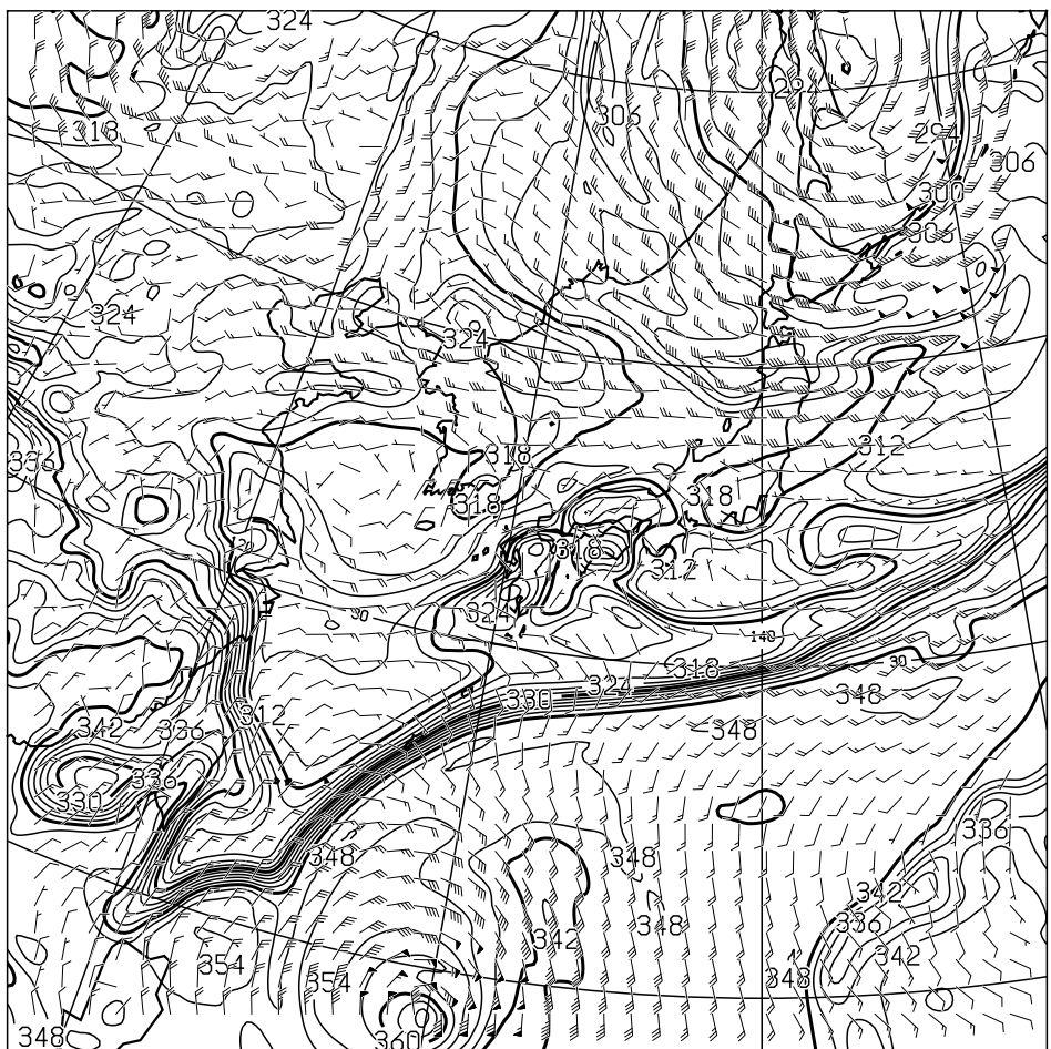
T=48 850hPa: E.P.TEMP(K),WIND(KNOTS) VALID 301200UTC
