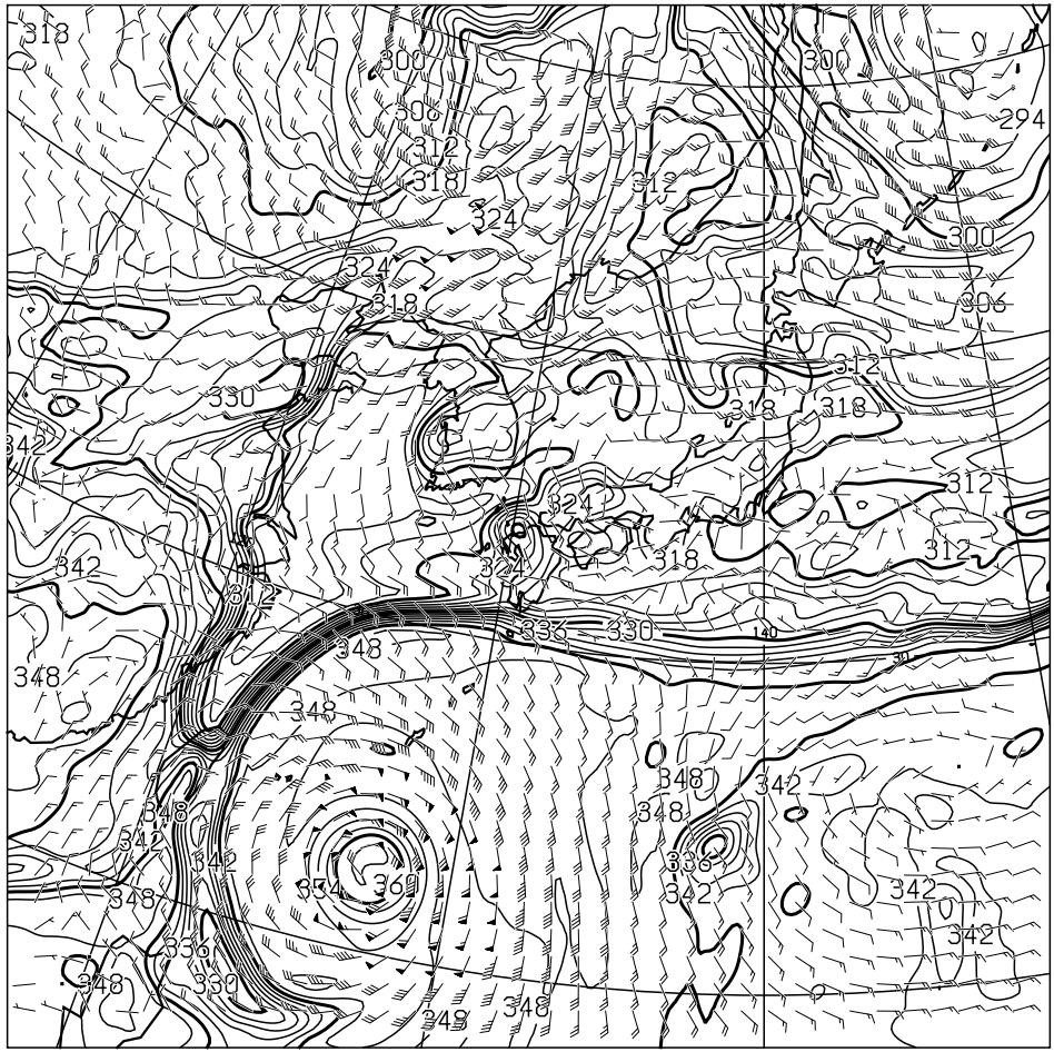
T=24 850hPa: E.P.TEMP(K),WIND(KNOTS) VALID 311200UTC
