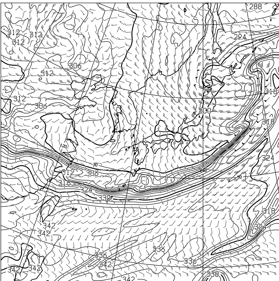
T=36 850hPa: E.P.TEMP(K),WIND(KNOTS) VALID 090000UTC
