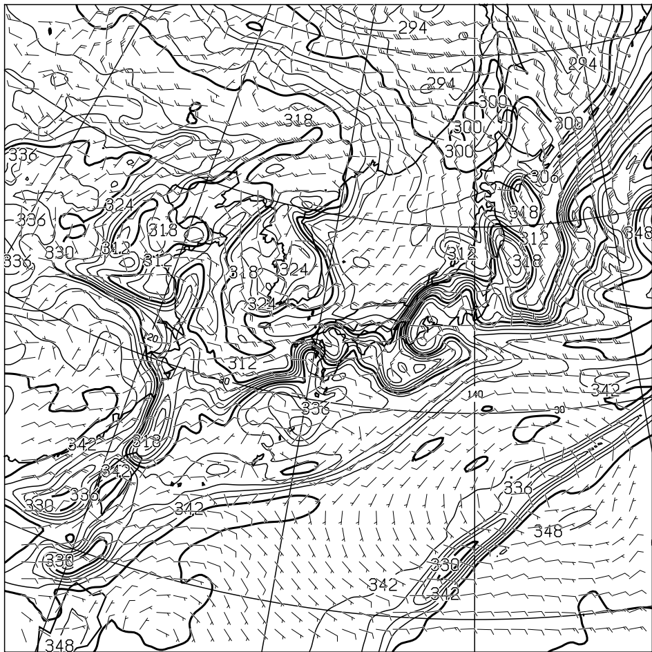
T=24 850hPa: E.P.TEMP(K),WIND(KNOTS) VALID 221200UTC
