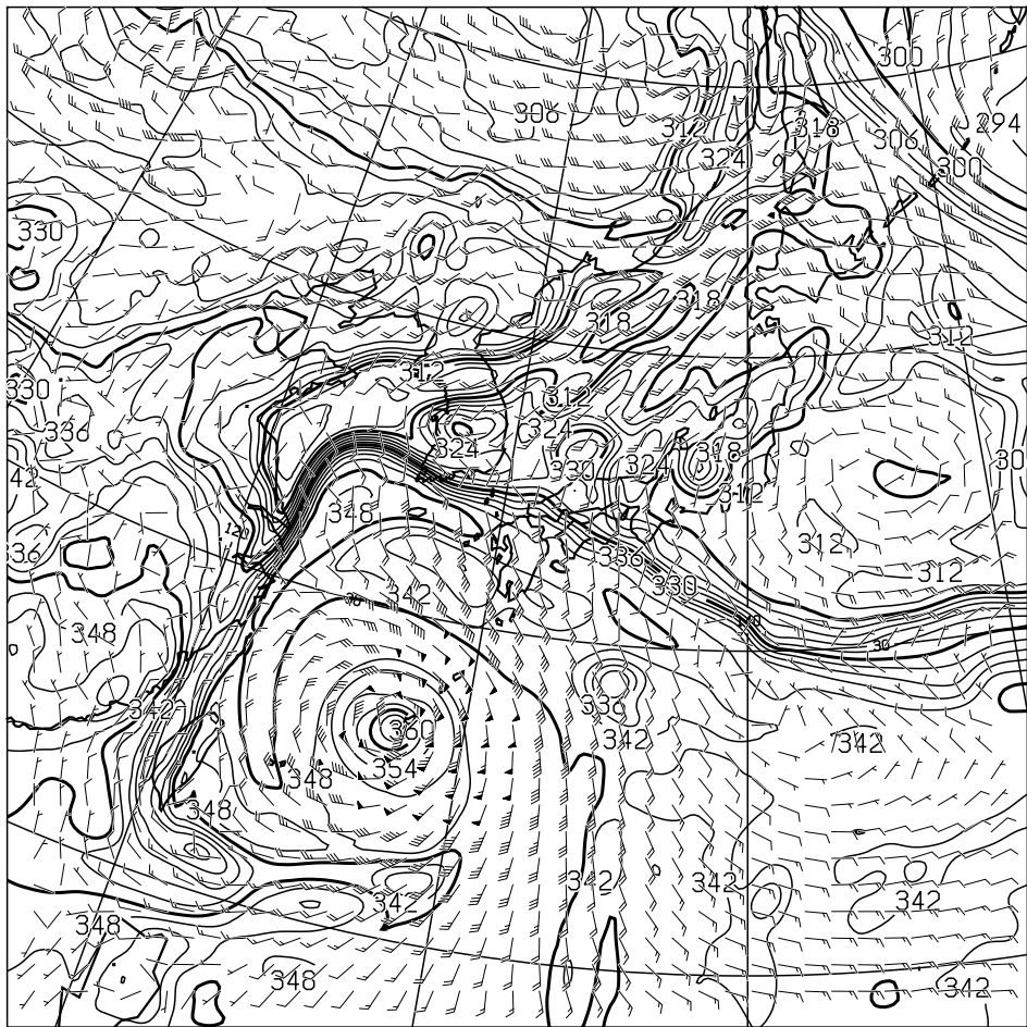
T=24 850hPa: E.P.TEMP(K),WIND(KNOTS) VALID 011200UTC
