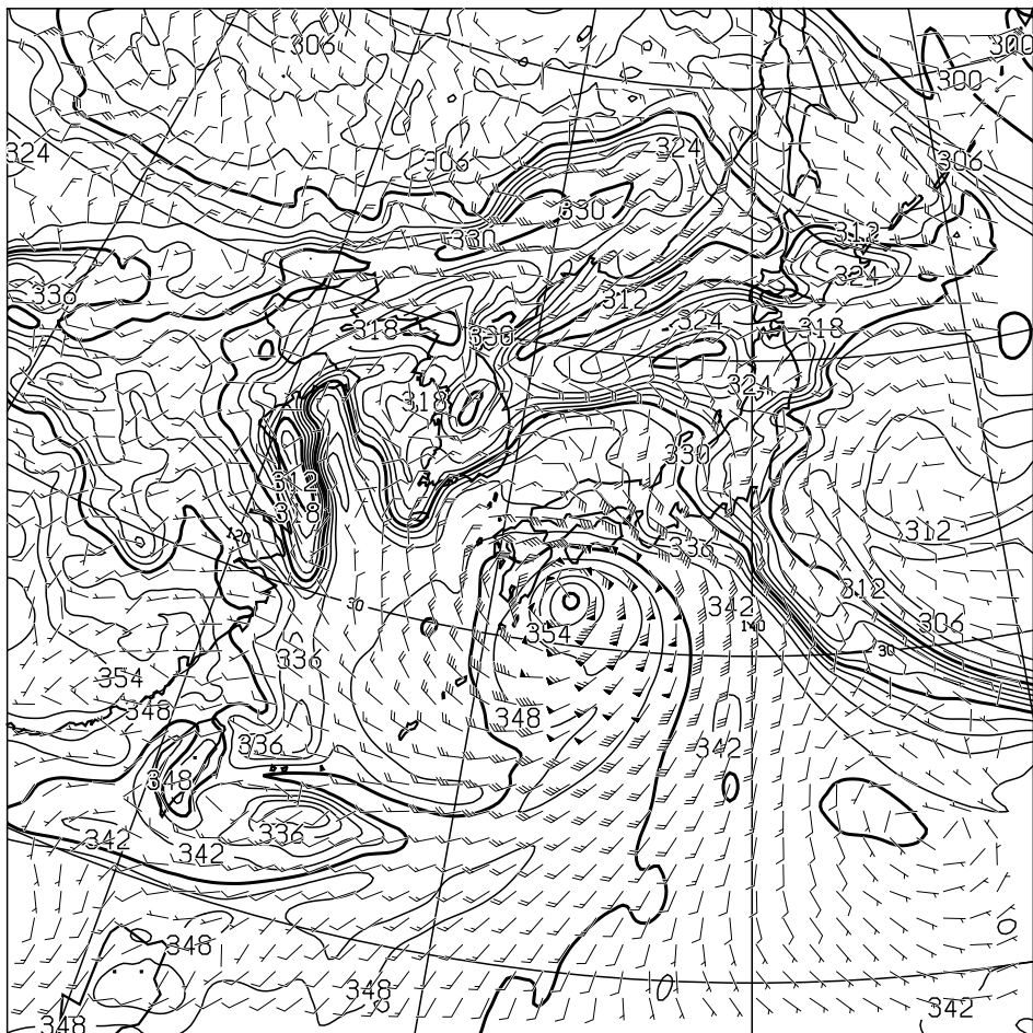
T=48 850hPa: E.P.TEMP(K),WIND(KNOTS) VALID 021200UTC
