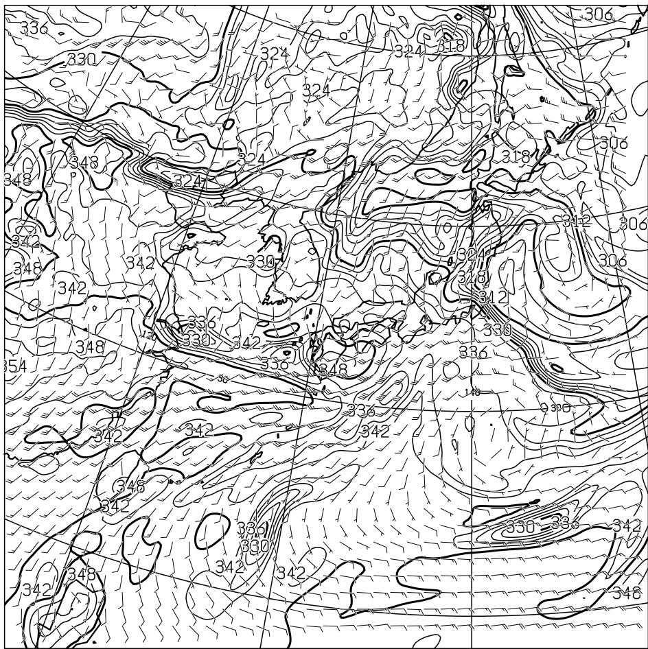
T=48 850hPa: E.P.TEMP(K),WIND(KNOTS) VALID 171200UTC
