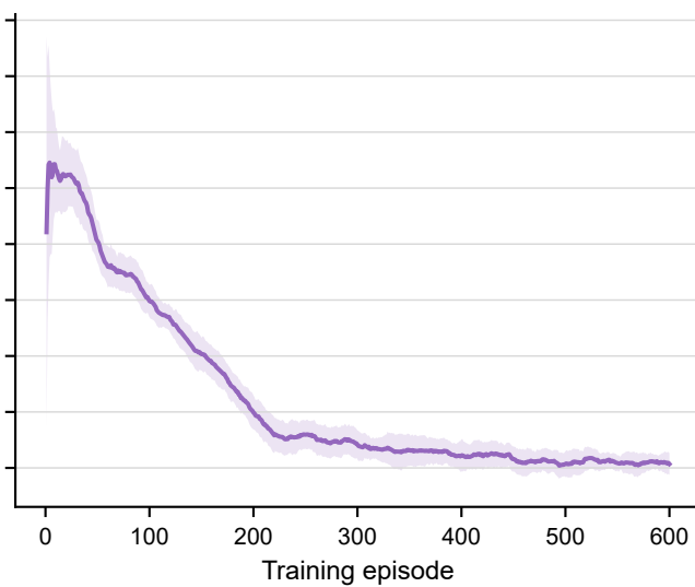
Double DQN
