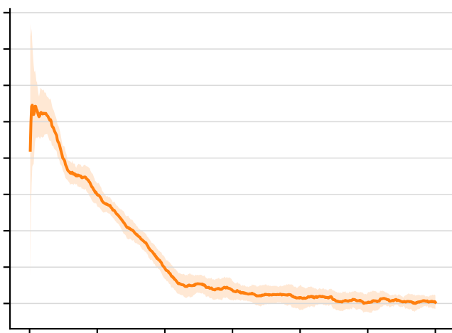
Double DQN
