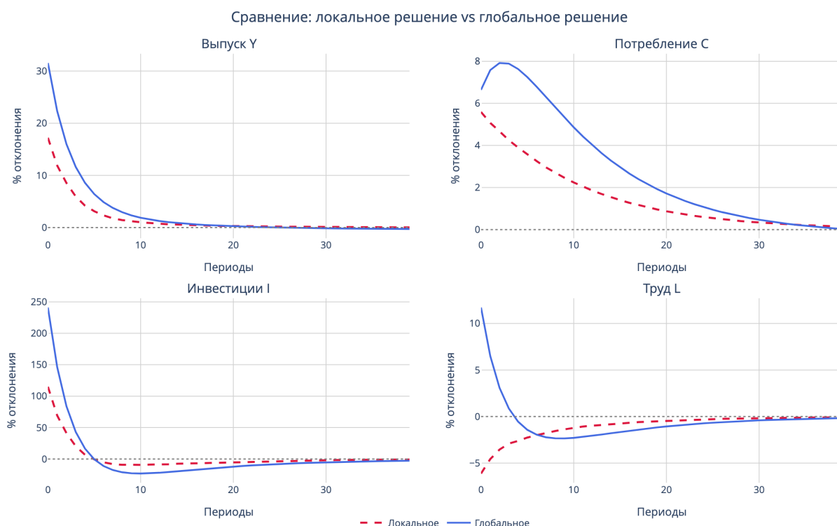
Рис. 5. Сравнение локального (Dynare, линейаризация 1-го порядка) и глобального (коллокация Чебышёва) решений: импульсные функции отклика выпуска Y , потребления C , инвестиций I и труда L на шок совокупной факторной производительности с \sigma_{tfp} = 0,2 .
