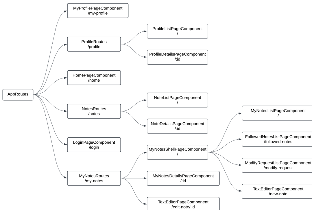
6.7. ábra: Routing fa
