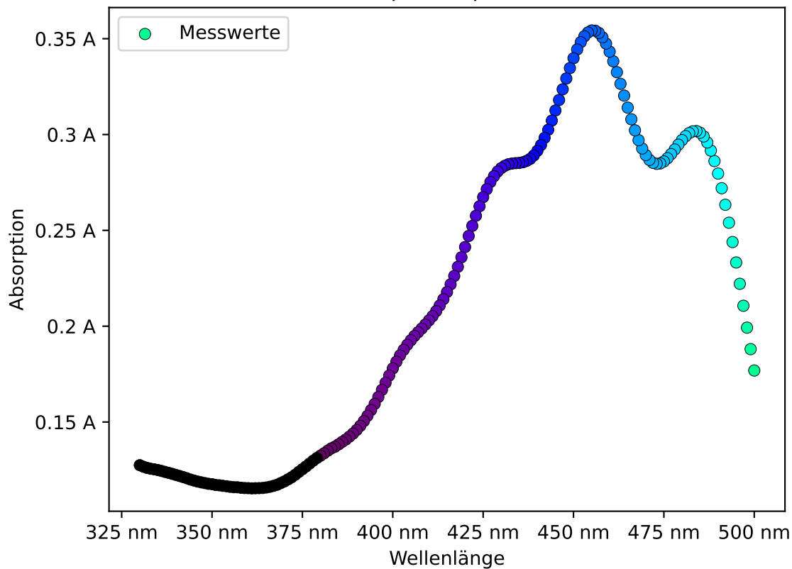
Absorptionsspektrum
