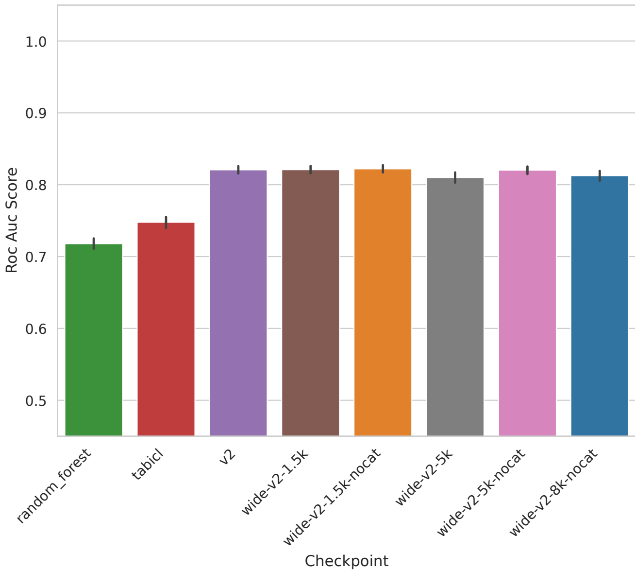
Task 363671 - Roc Auc Score
