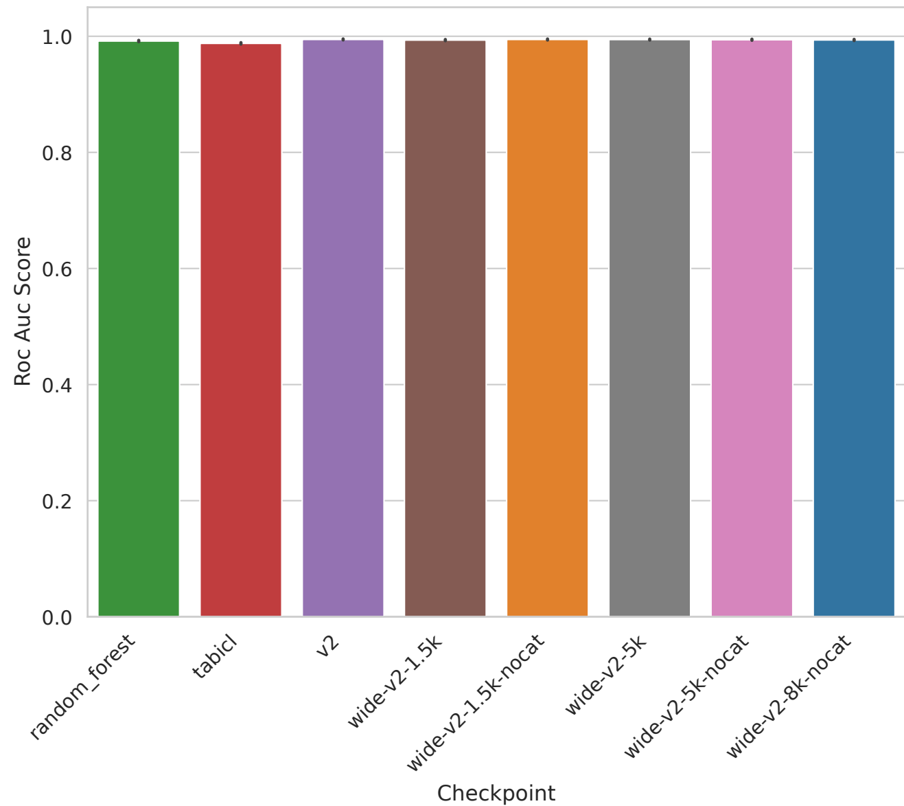
Task 363702 - Roc Auc Score
