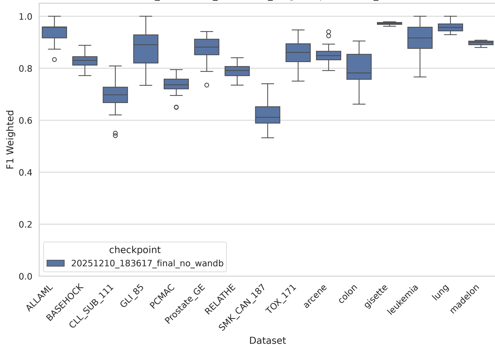
hdlss_benchmark_results - f1_weighted per dataset_name
