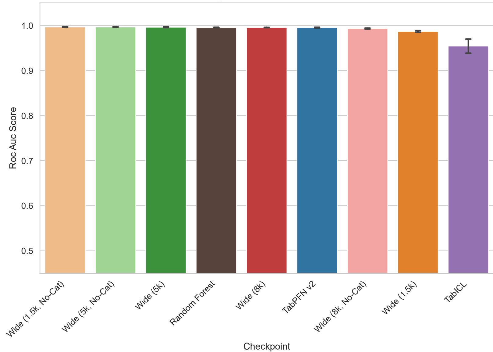
gisette - Roc Auc Score
