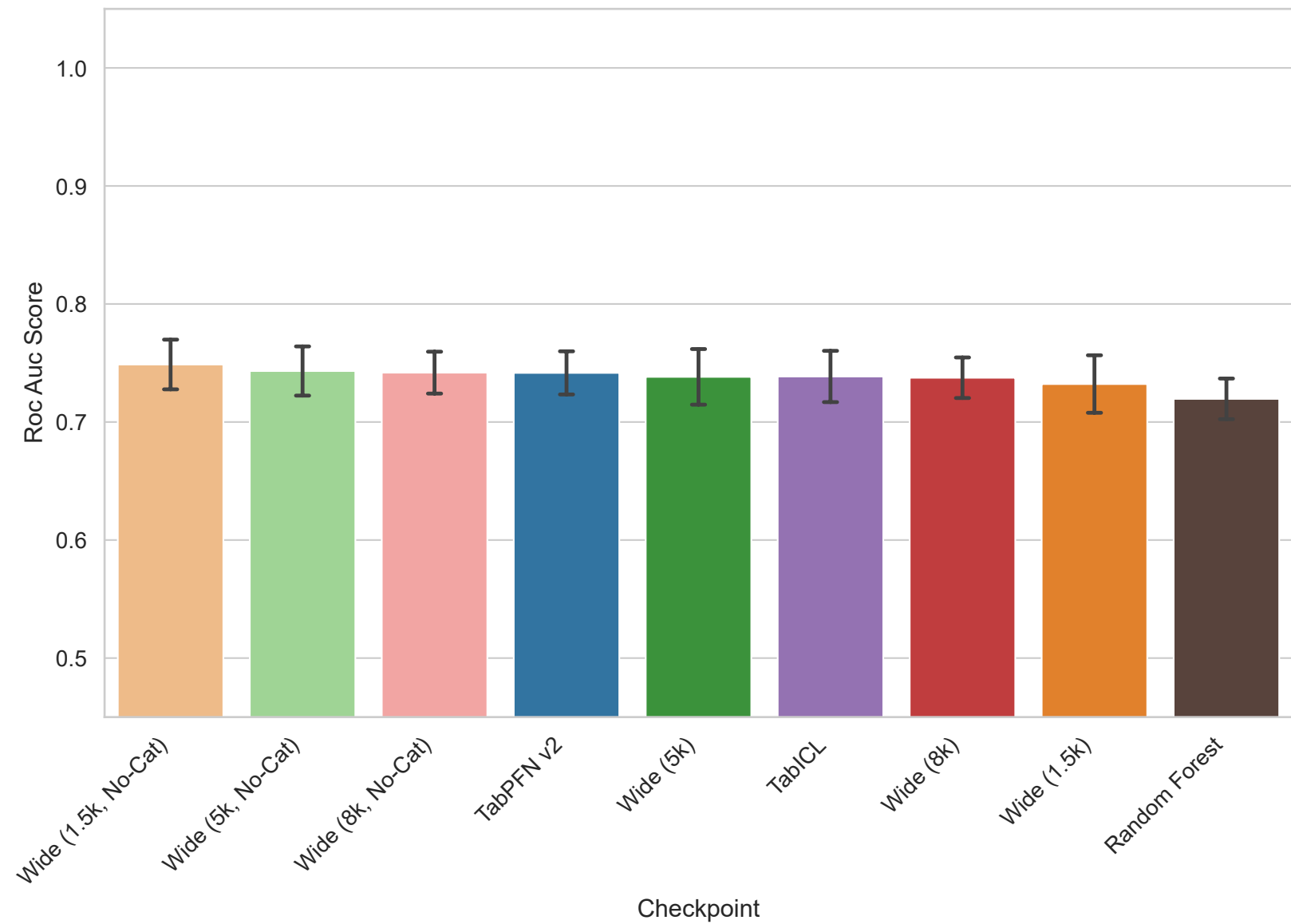
Task 363682 - Roc Auc Score
