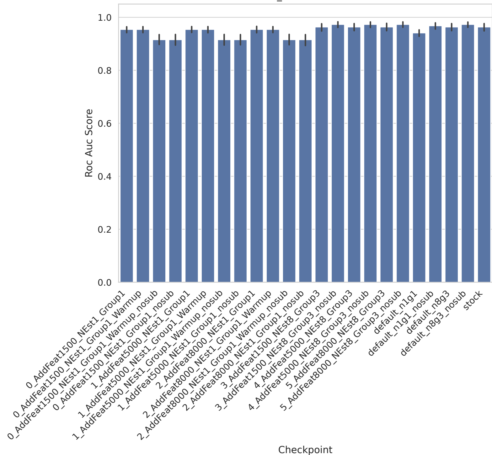
Prostate_GE - Roc Auc Score
