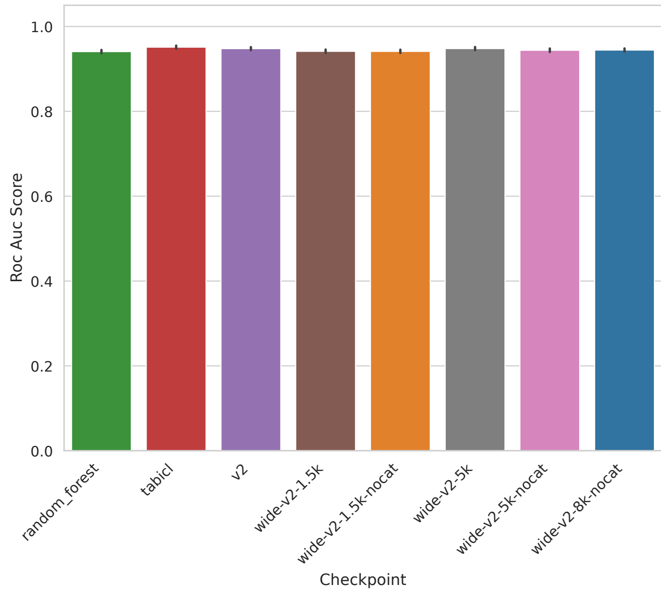
Task 363685 - Roc Auc Score
