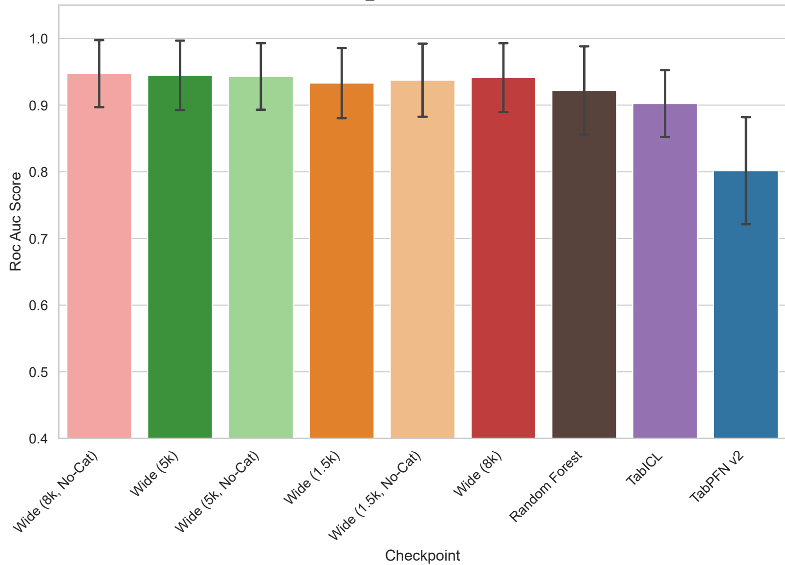
GLI_85 - Roc Auc Score
