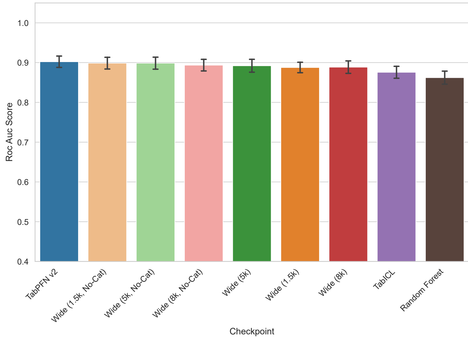
Task 363684 - Roc Auc Score
