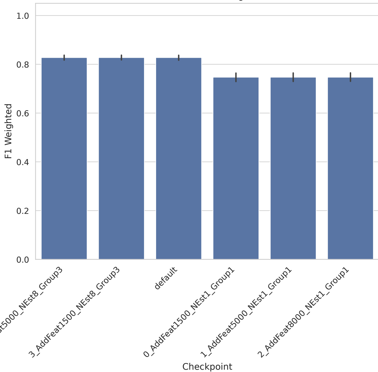
BASEHOCK - F1 Weighted
