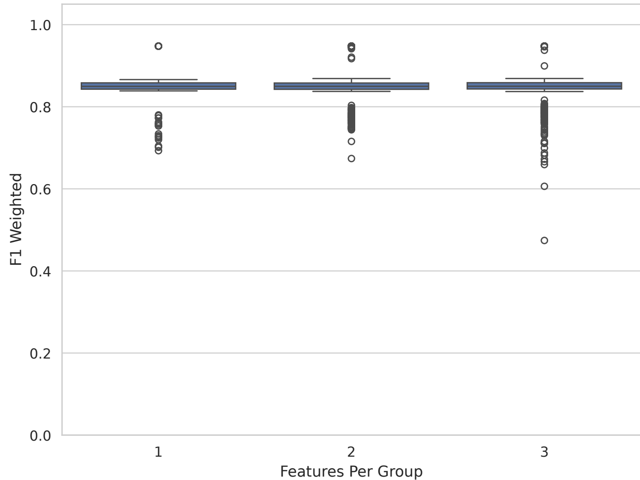
Impact of Grouping on F1 Weighted
