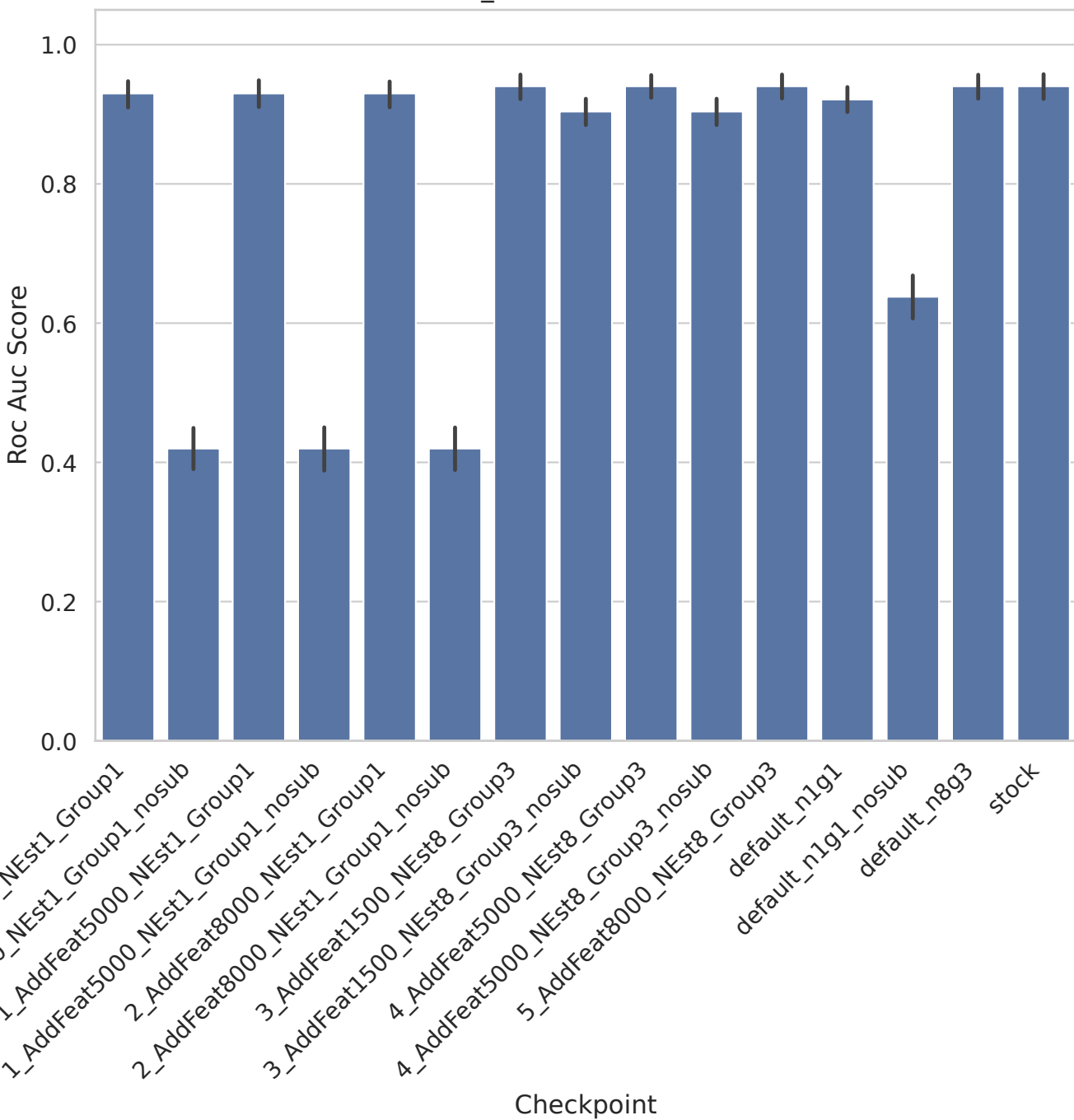
GLI_85 - Roc Auc Score
