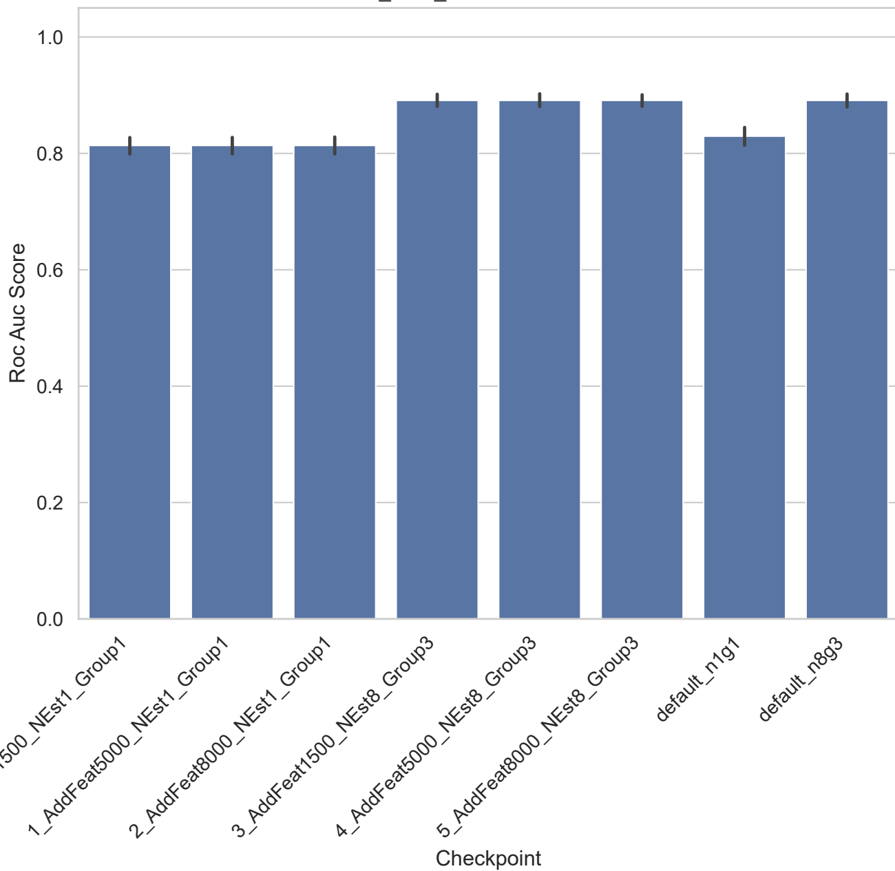
CLL_SUB_111 - Roc Auc Score
