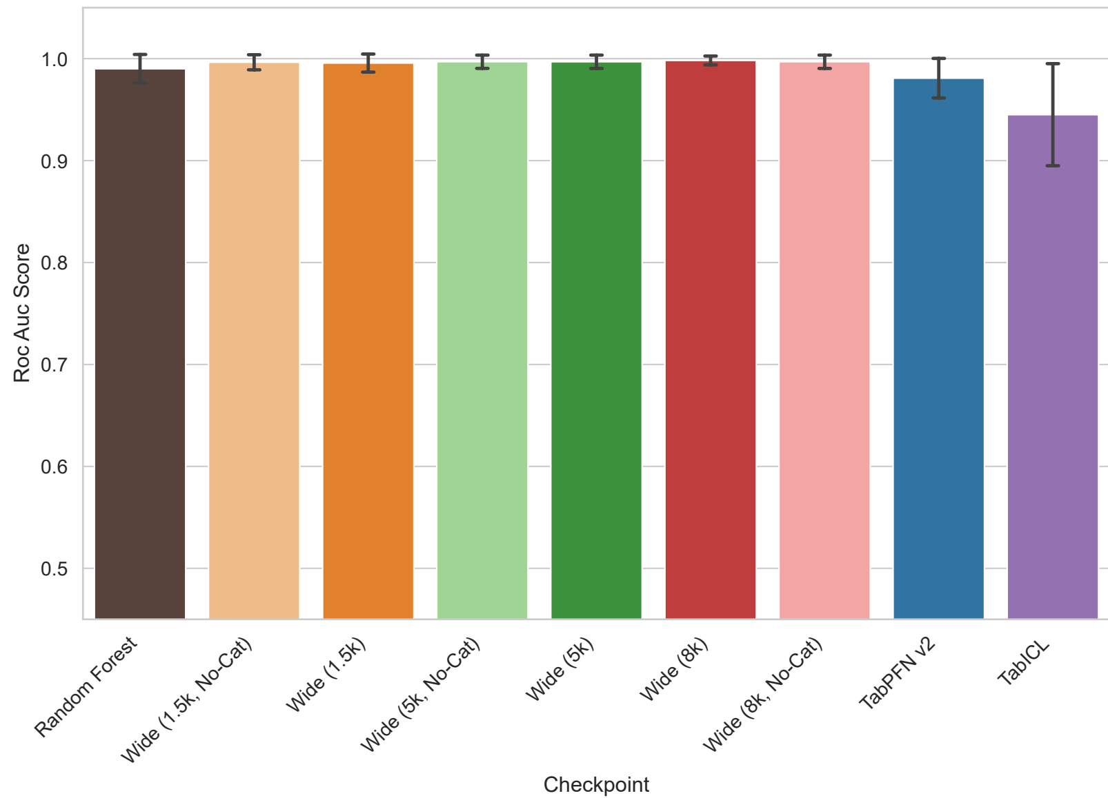
leukemia - Roc Auc Score
