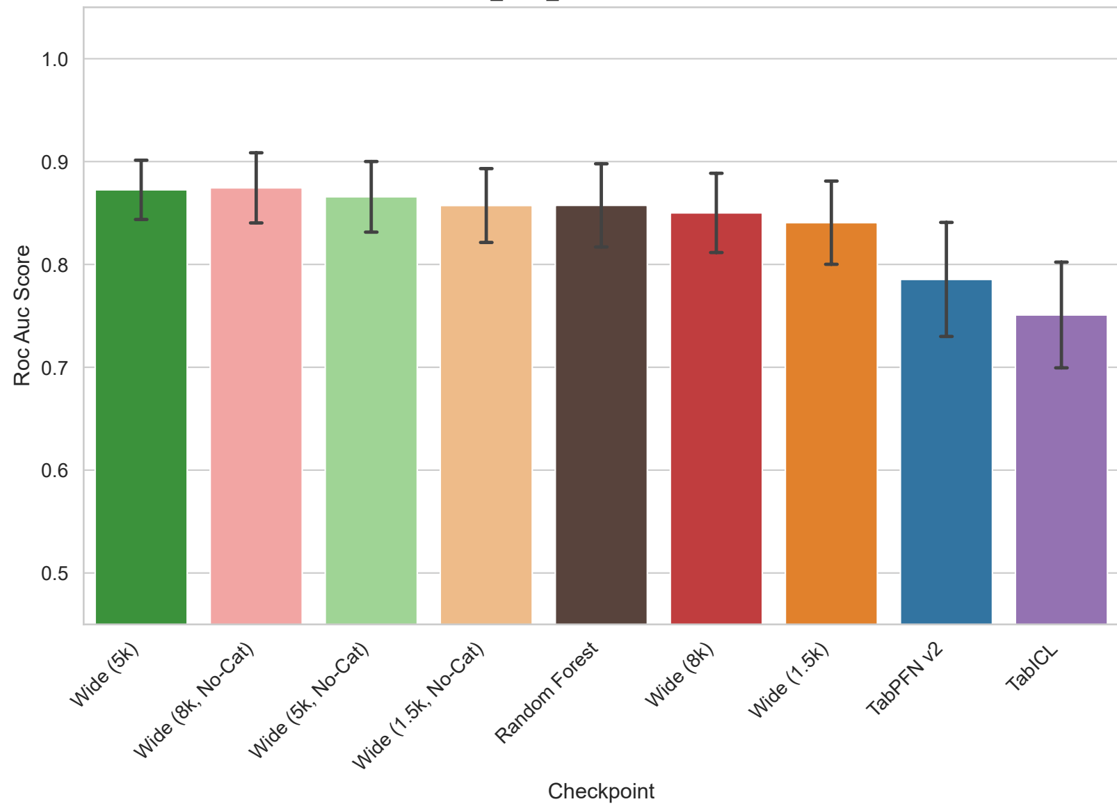
CLL_SUB_111 - Roc Auc Score
