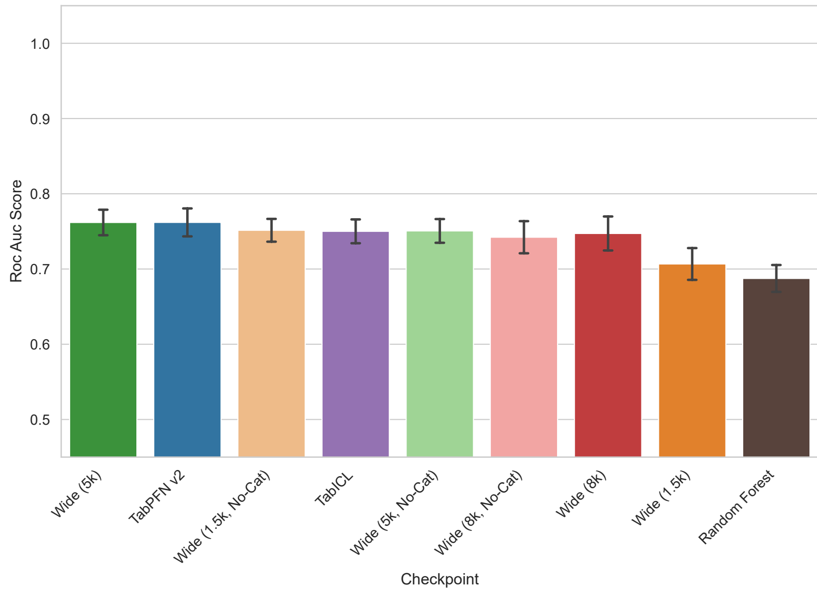
Task 363624 - Roc Auc Score
