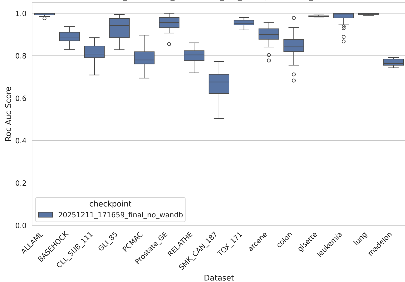
hdls_benchmark_results - roc_auc_score per dataset_name
