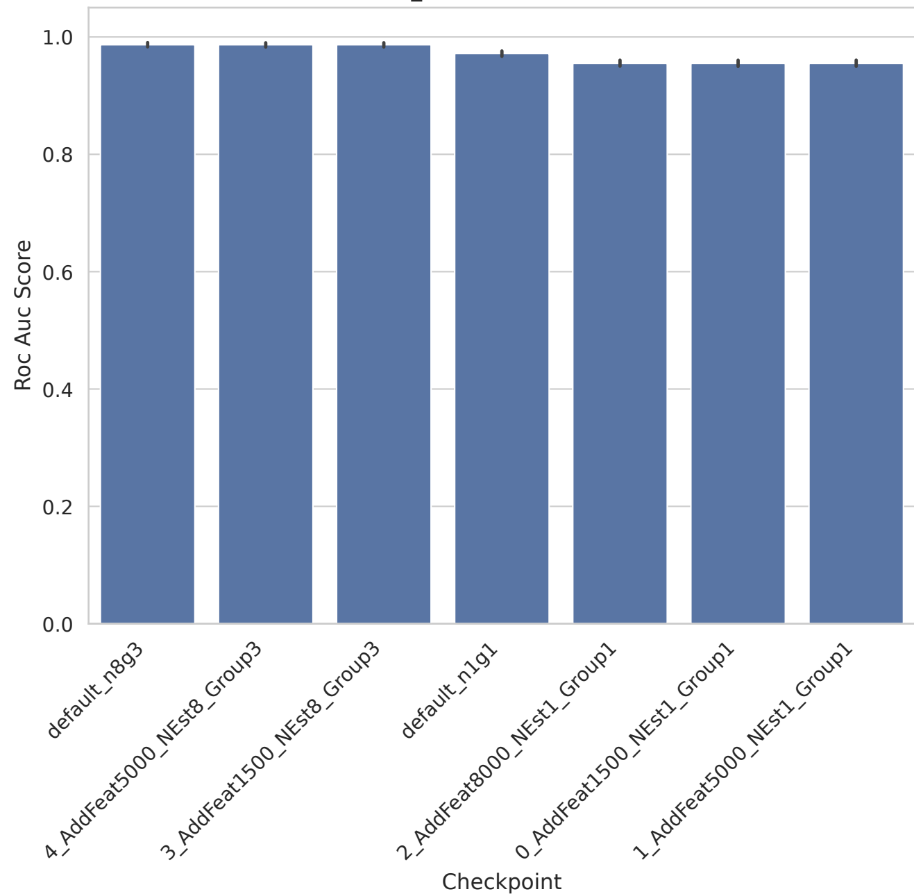
TOX_171 - Roc Auc Score
