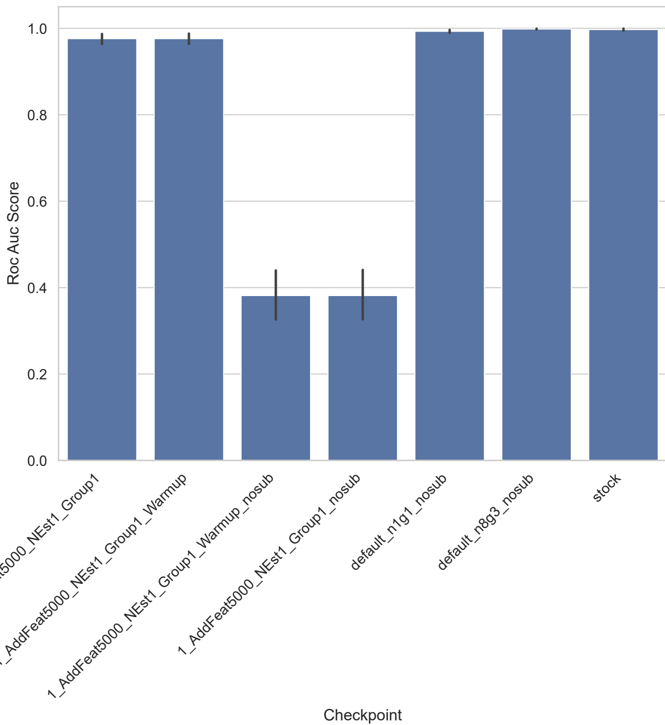
leukemia - Roc Auc Score
