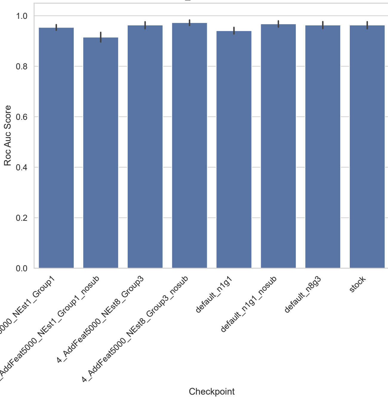
Prostate_GE - Roc Auc Score
