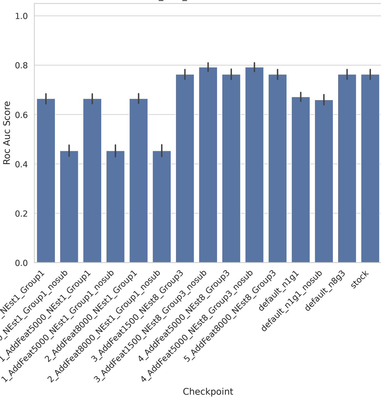
SMK_CAN_187 - Roc Auc Score
