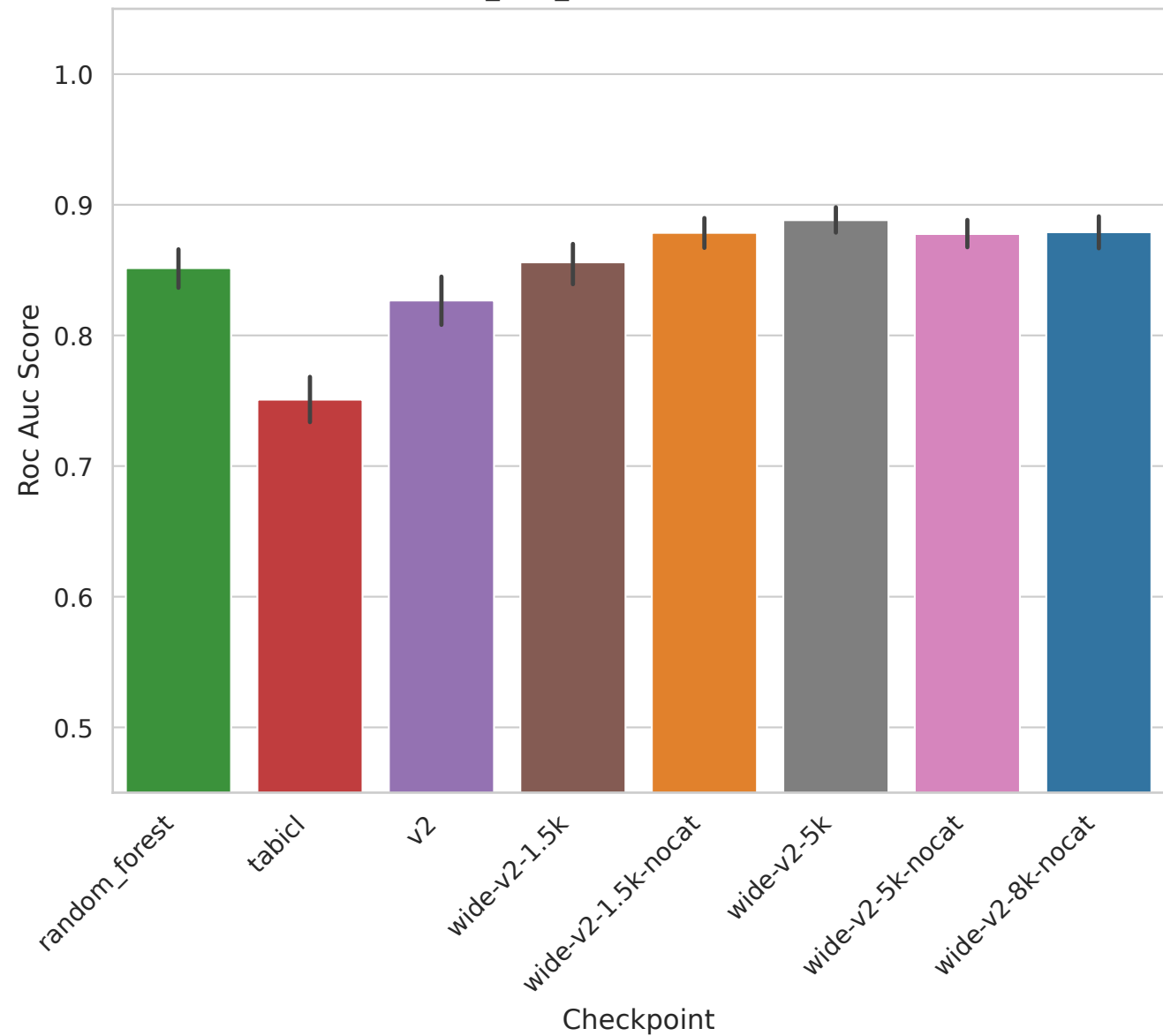
CLL_SUB_111 - Roc Auc Score
