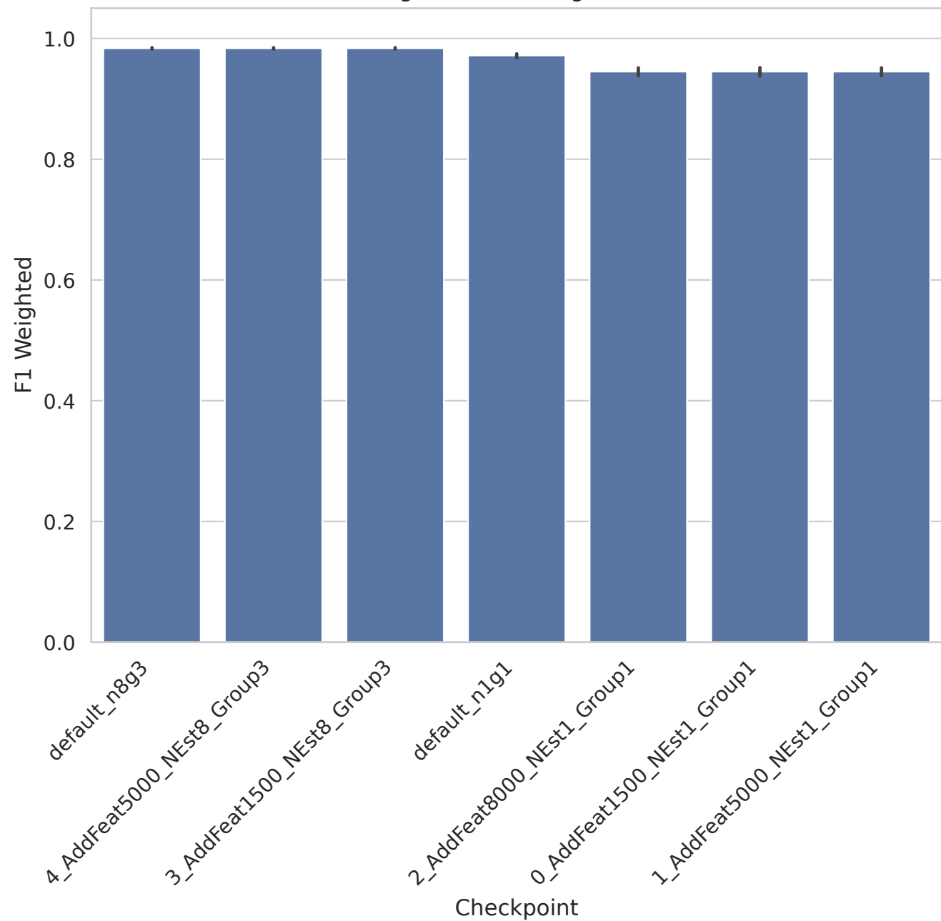
gisette - F1 Weighted
