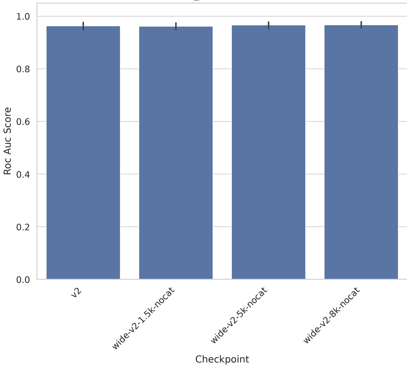
Prostate_GE - Roc Auc Score
