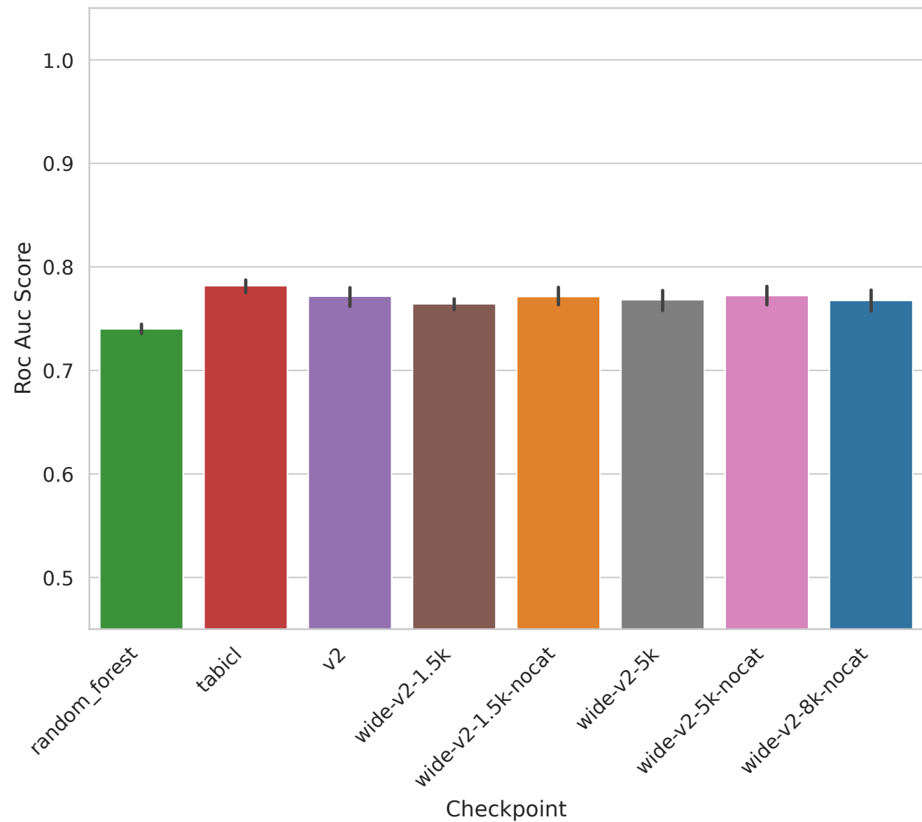
Task 363700 - Roc Auc Score
