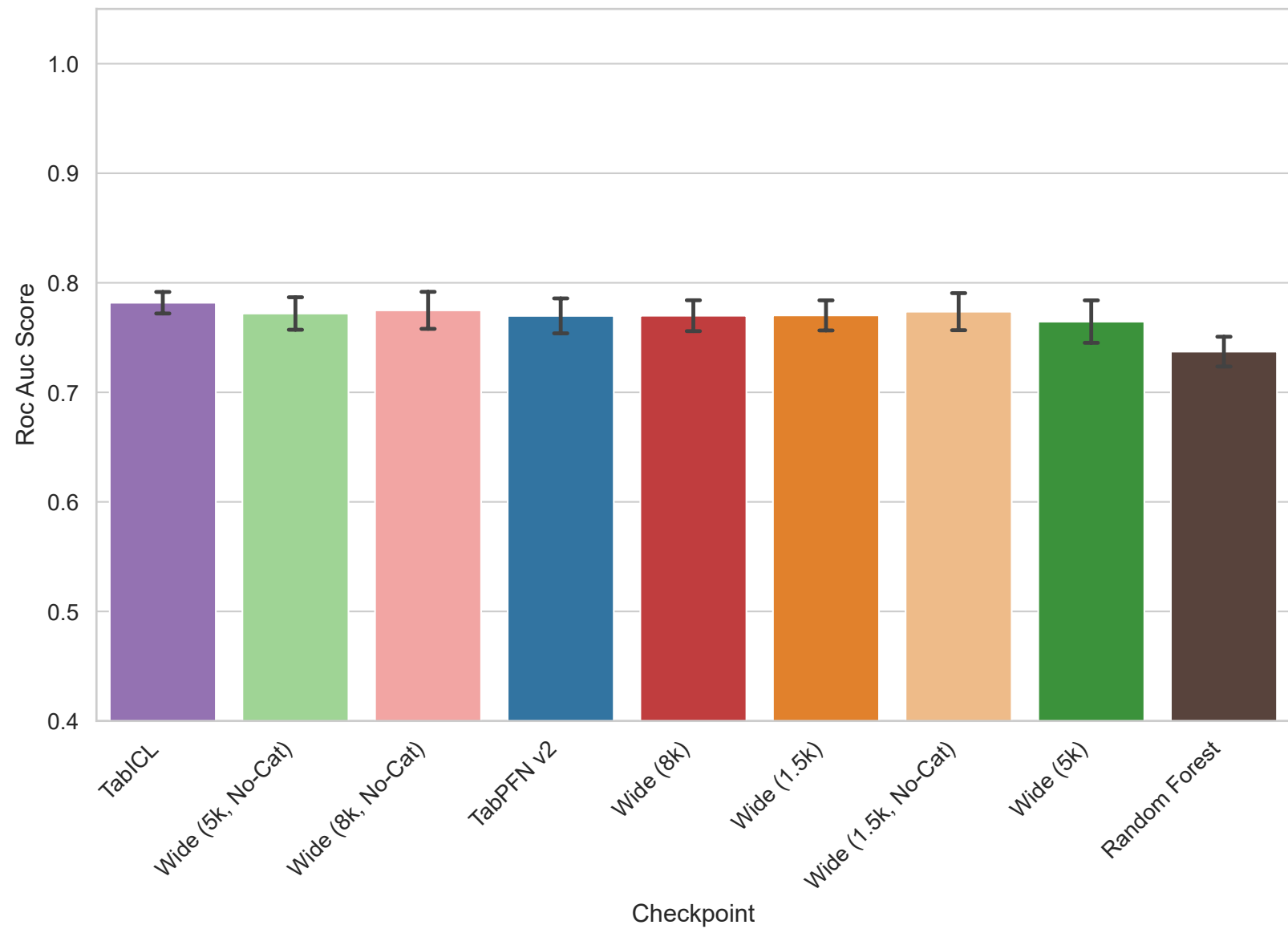
Task 363700 - Roc Auc Score
