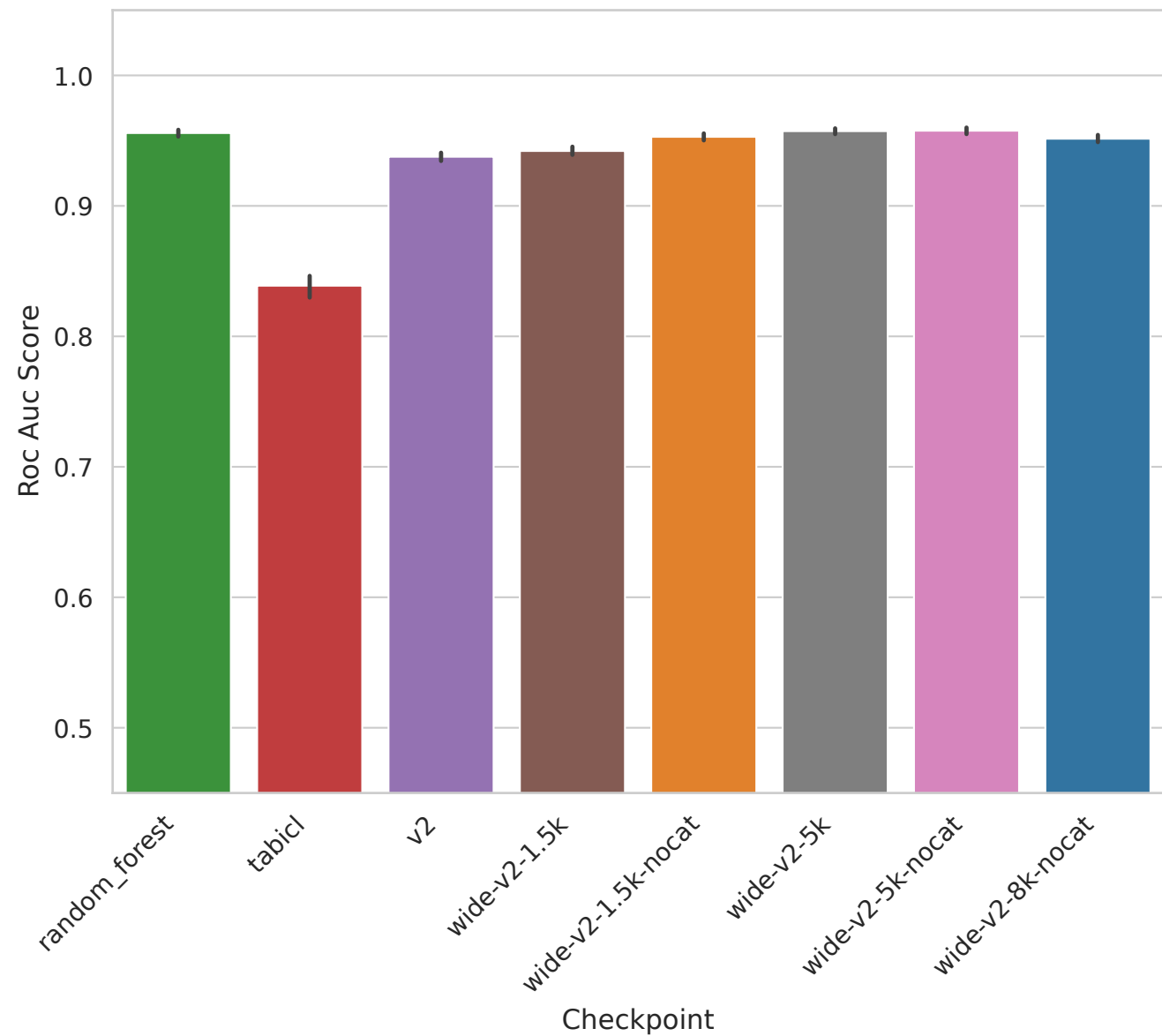
RELATHE - Roc Auc Score
