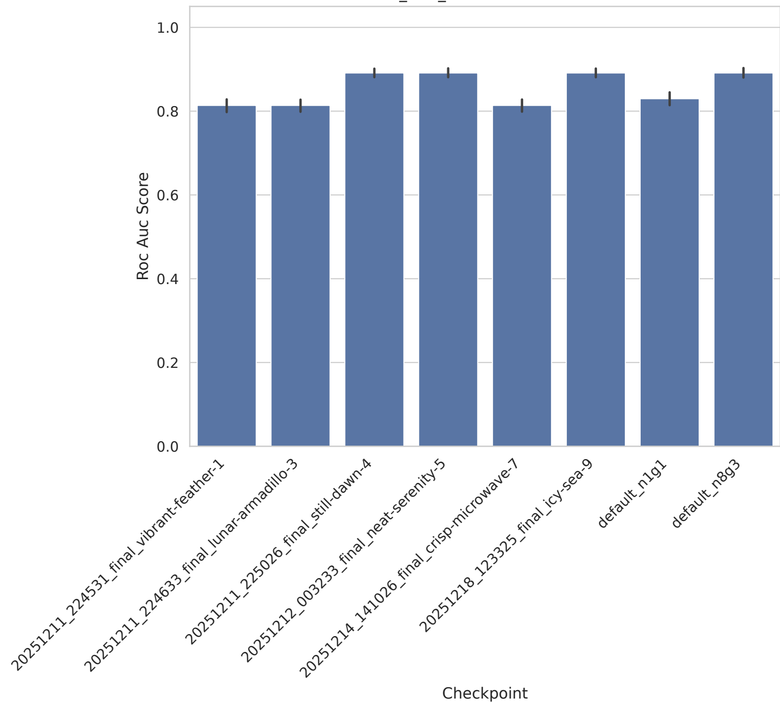
CLL_SUB_111 - Roc Auc Score
