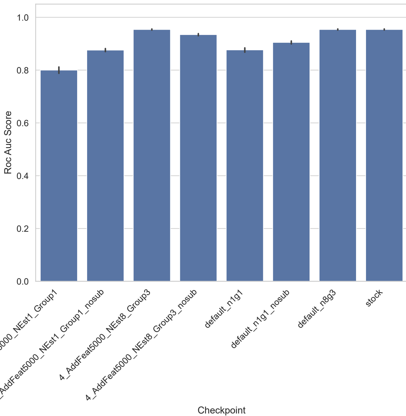
RELATHE - Roc Auc Score
