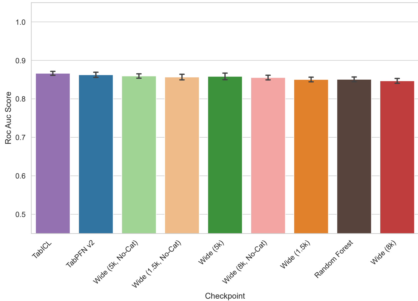
Task 363619 - Roc Auc Score
