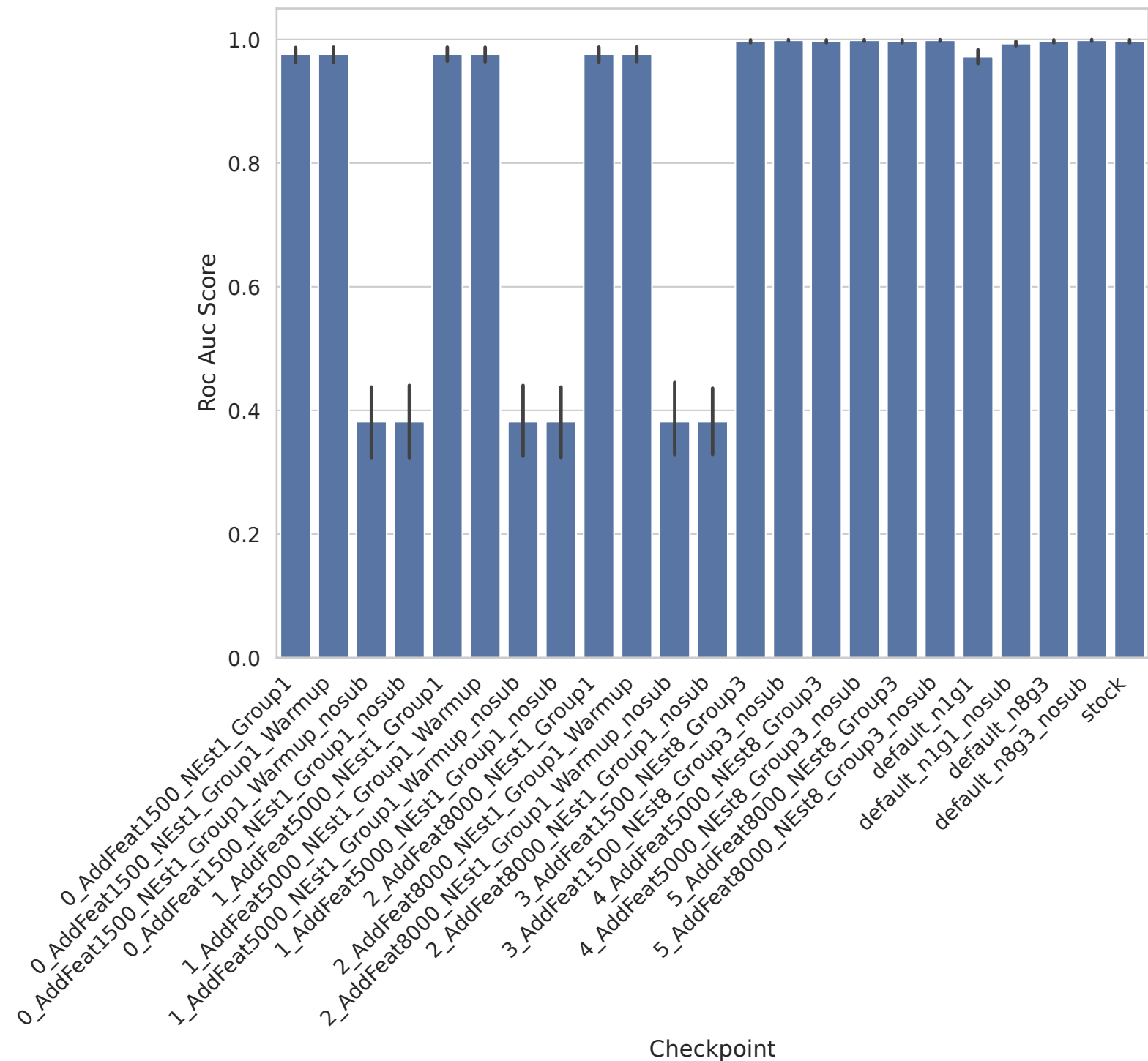
leukemia - Roc Auc Score
