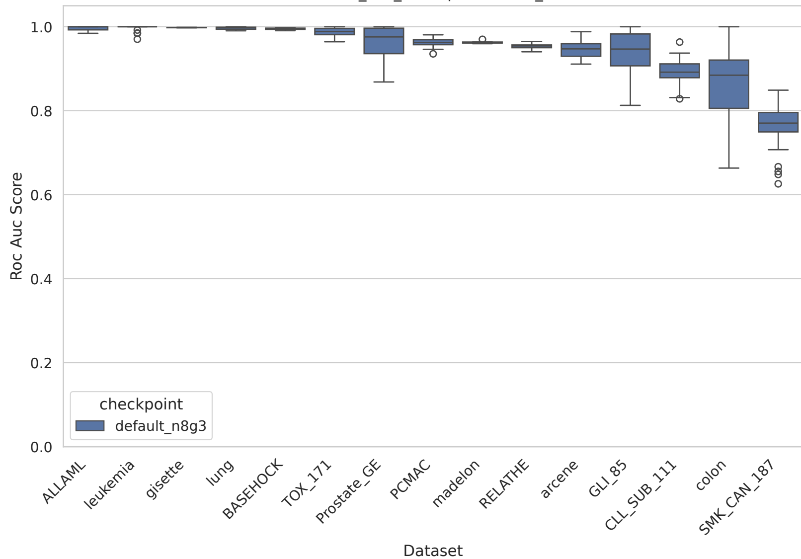
hdls - roc_auc_score per dataset_name
