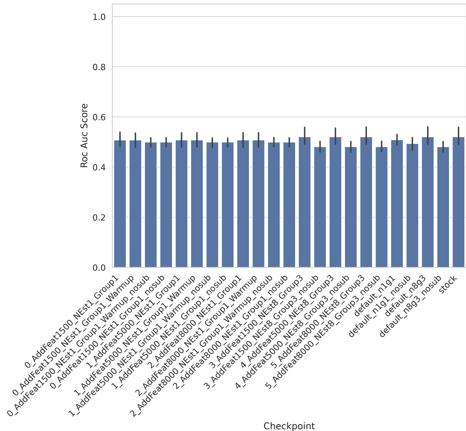
Task 363677 - Roc Auc Score
