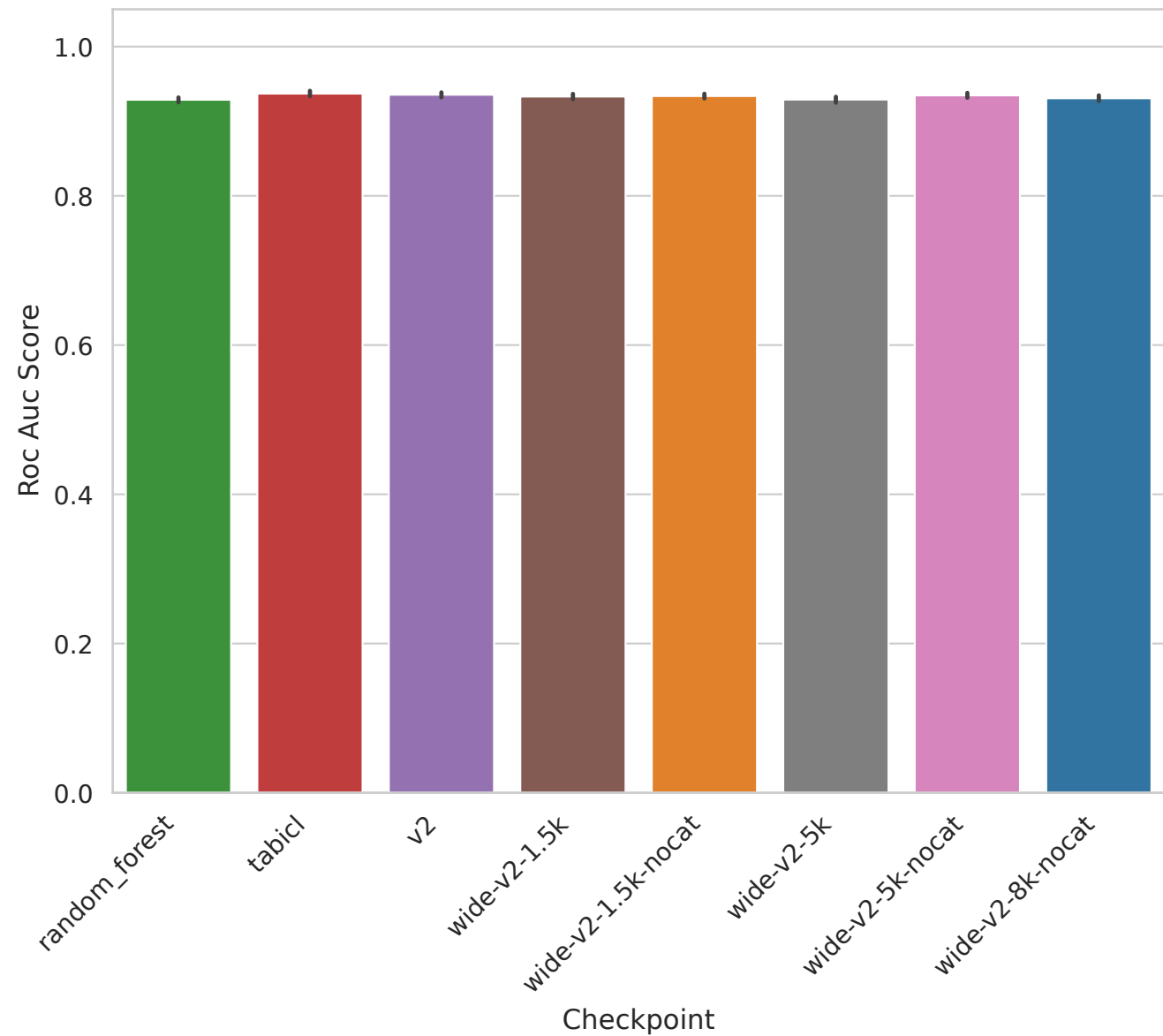
Task 363696 - Roc Auc Score
