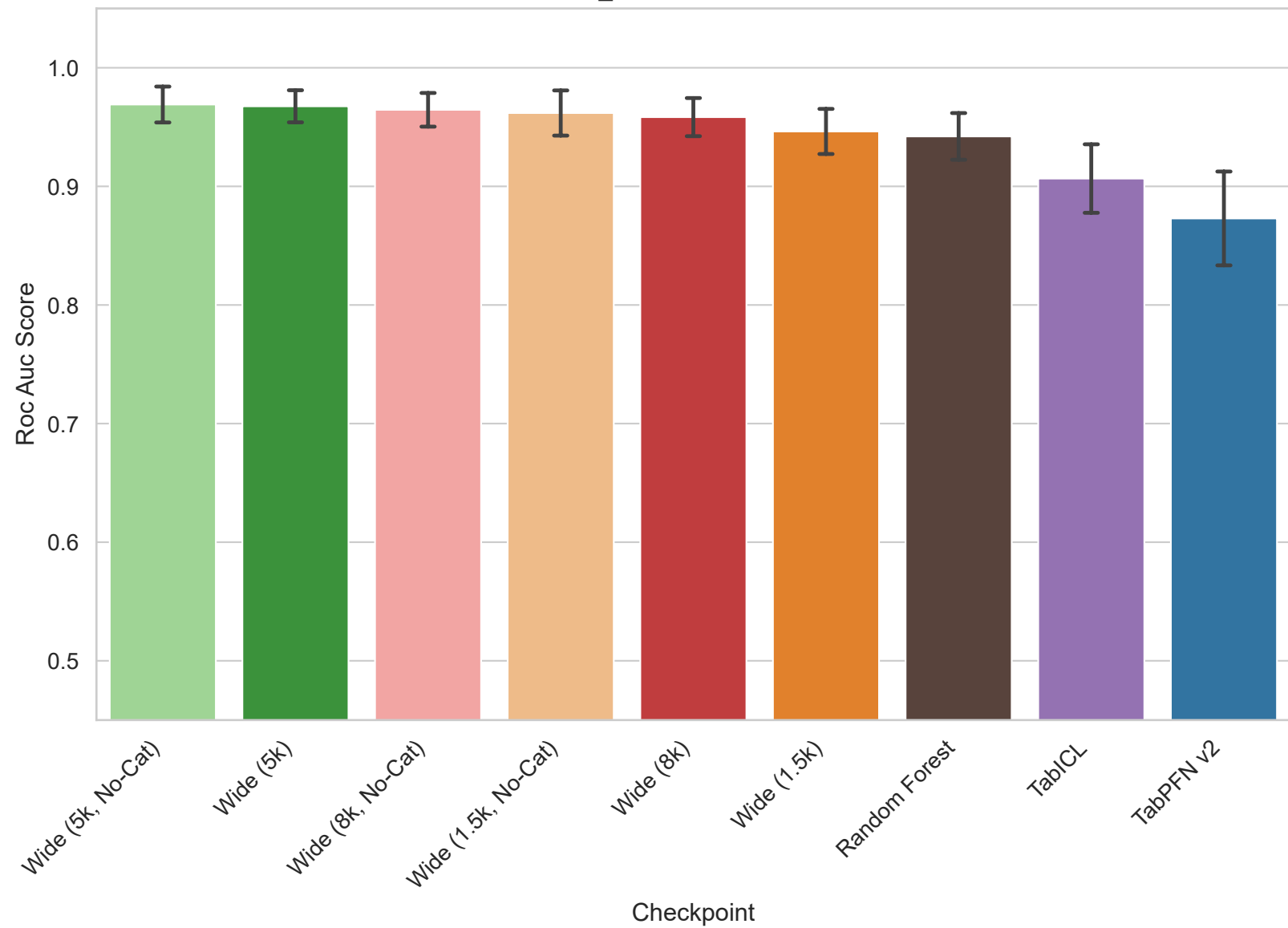
TOX_171 - Roc Auc Score
