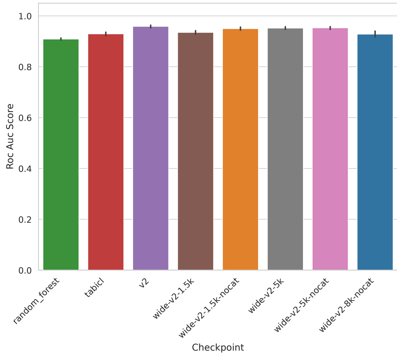
Task 363694 - Roc Auc Score
