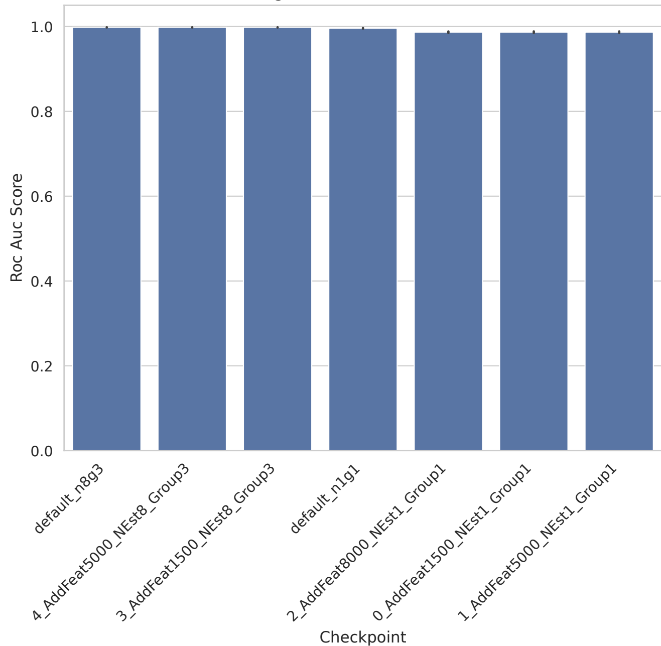
gisette - Roc Auc Score
