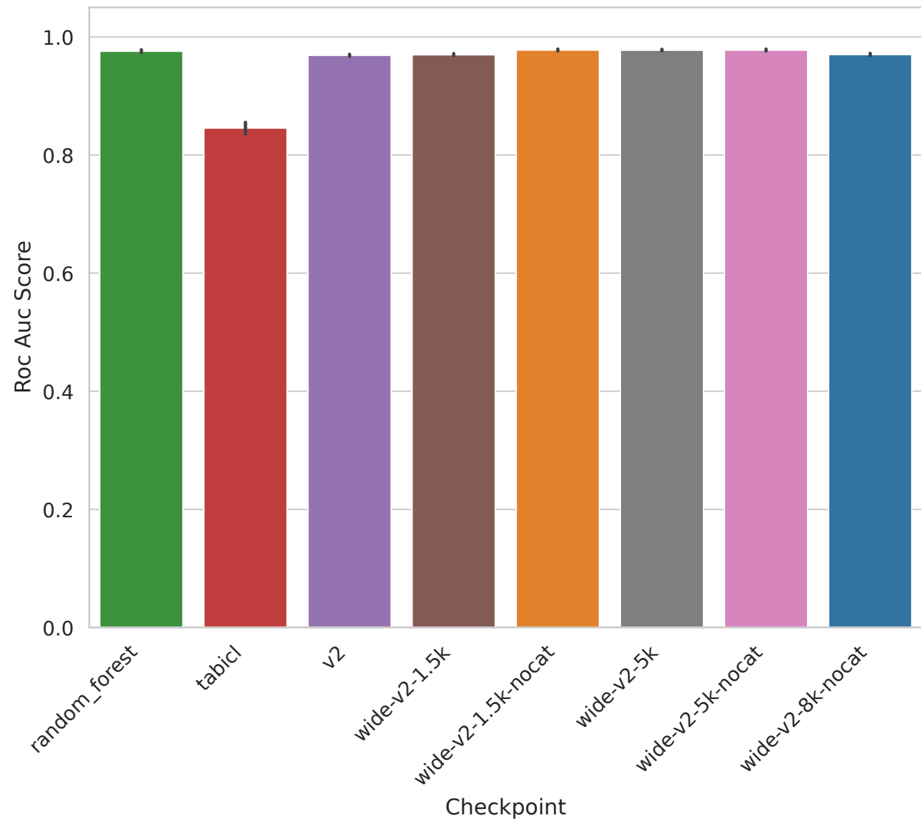
PCMAC - Roc Auc Score
