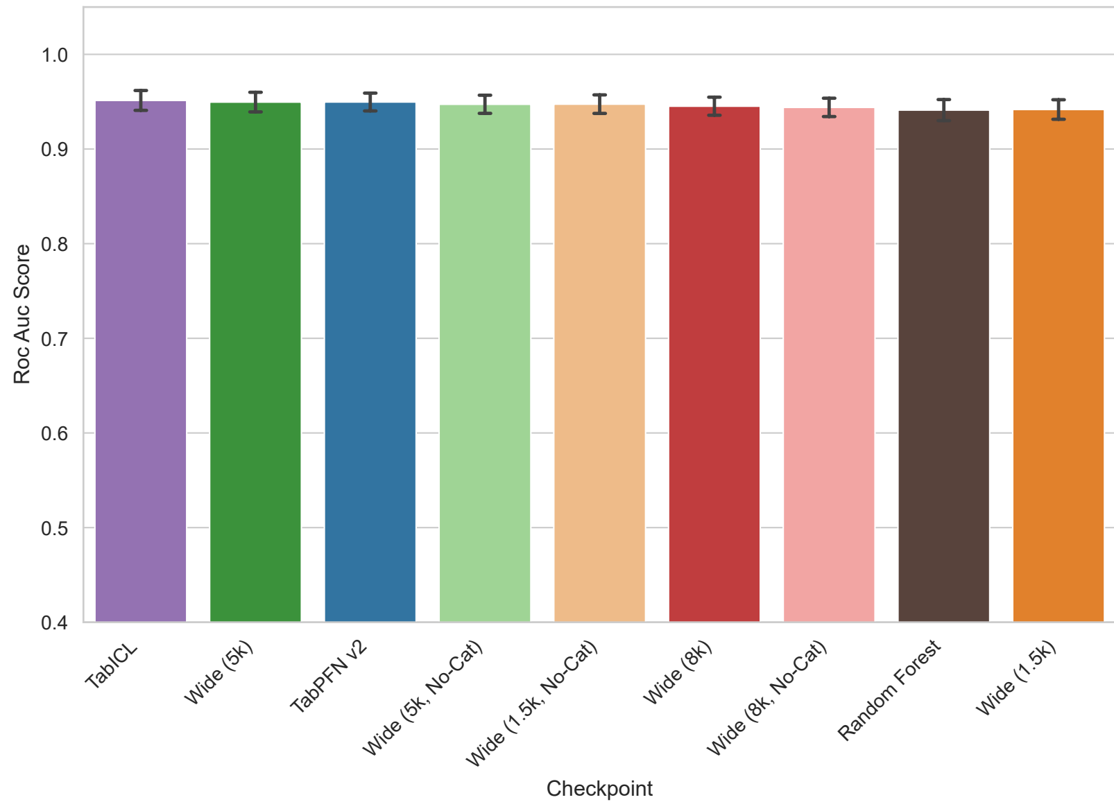
Task 363685 - Roc Auc Score
