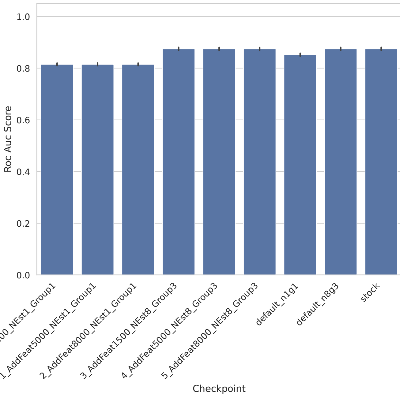
Task 363620 - Roc Auc Score
