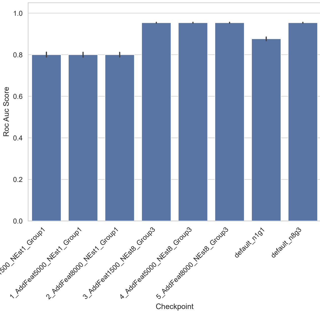
RELATHE - Roc Auc Score
