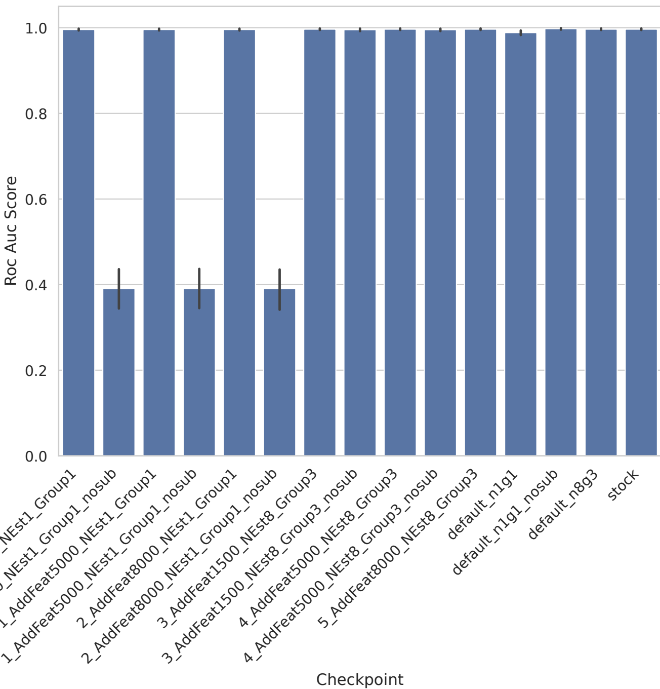
ALLAML - Roc Auc Score
