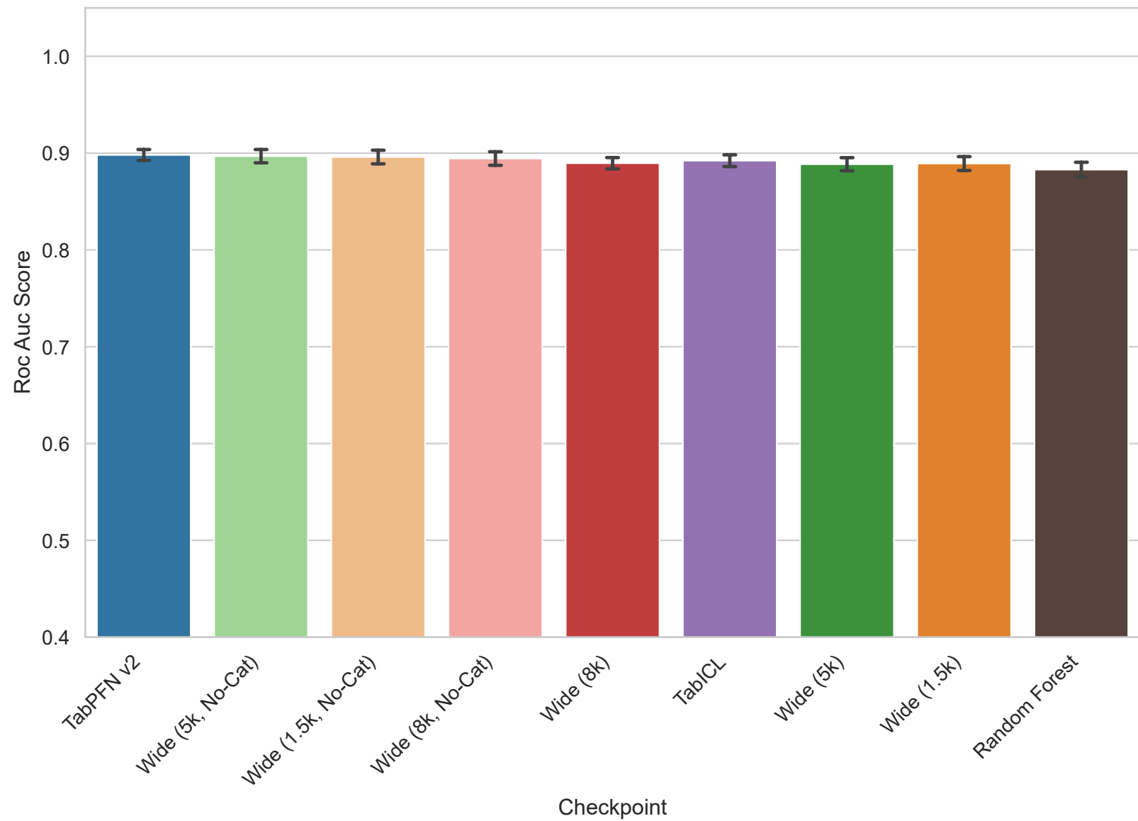
Task 363704 - Roc Auc Score
