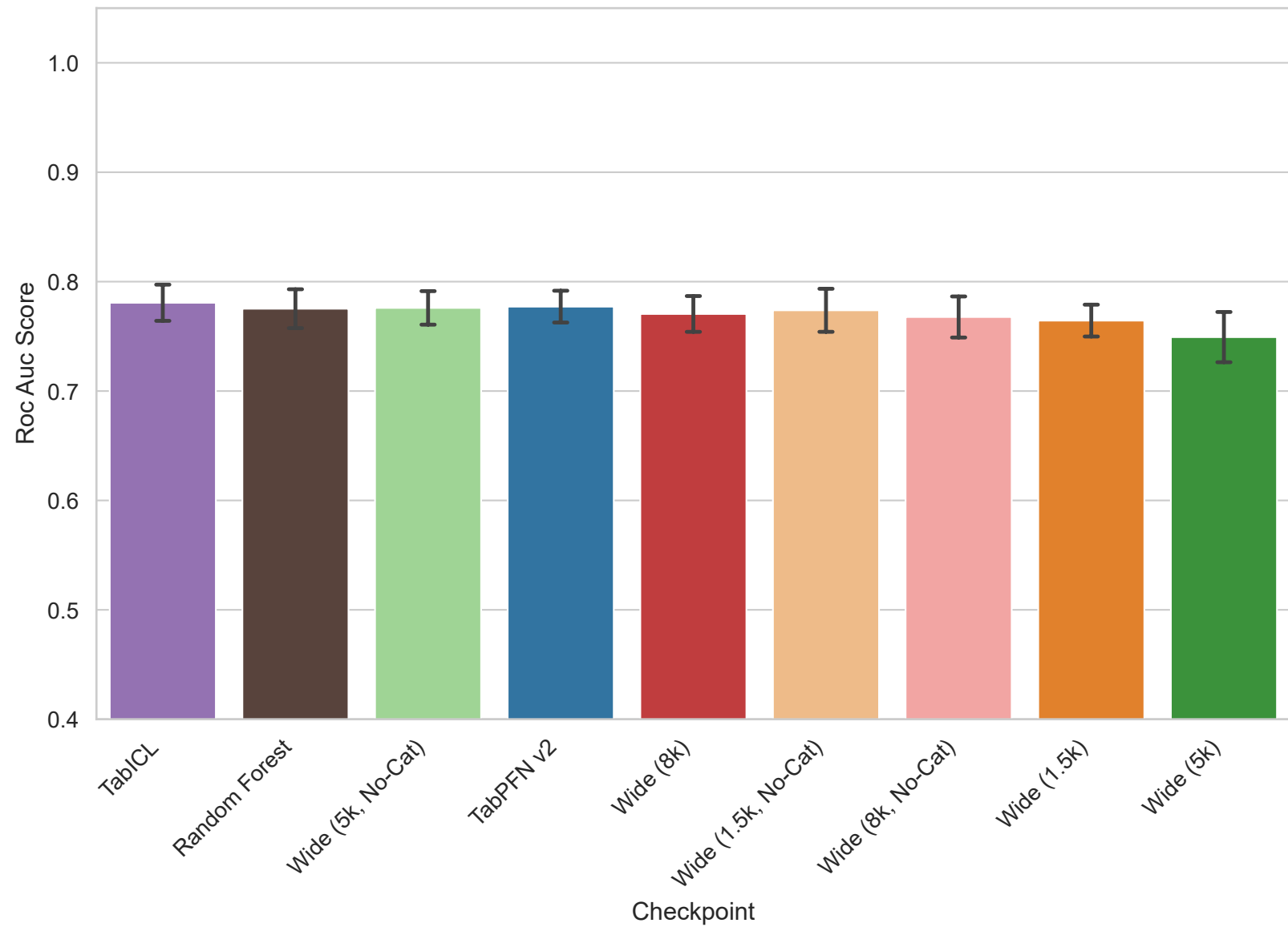
Task 363626 - Roc Auc Score
