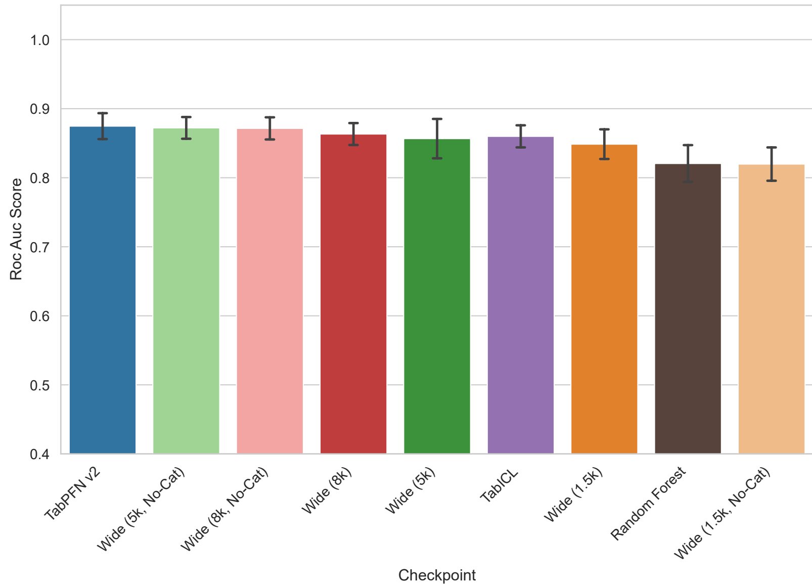
Task 363711 - Roc Auc Score
