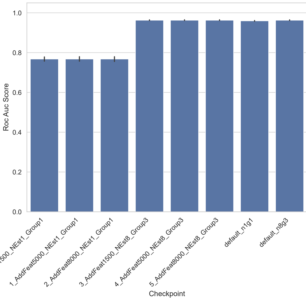
madelon - Roc Auc Score
