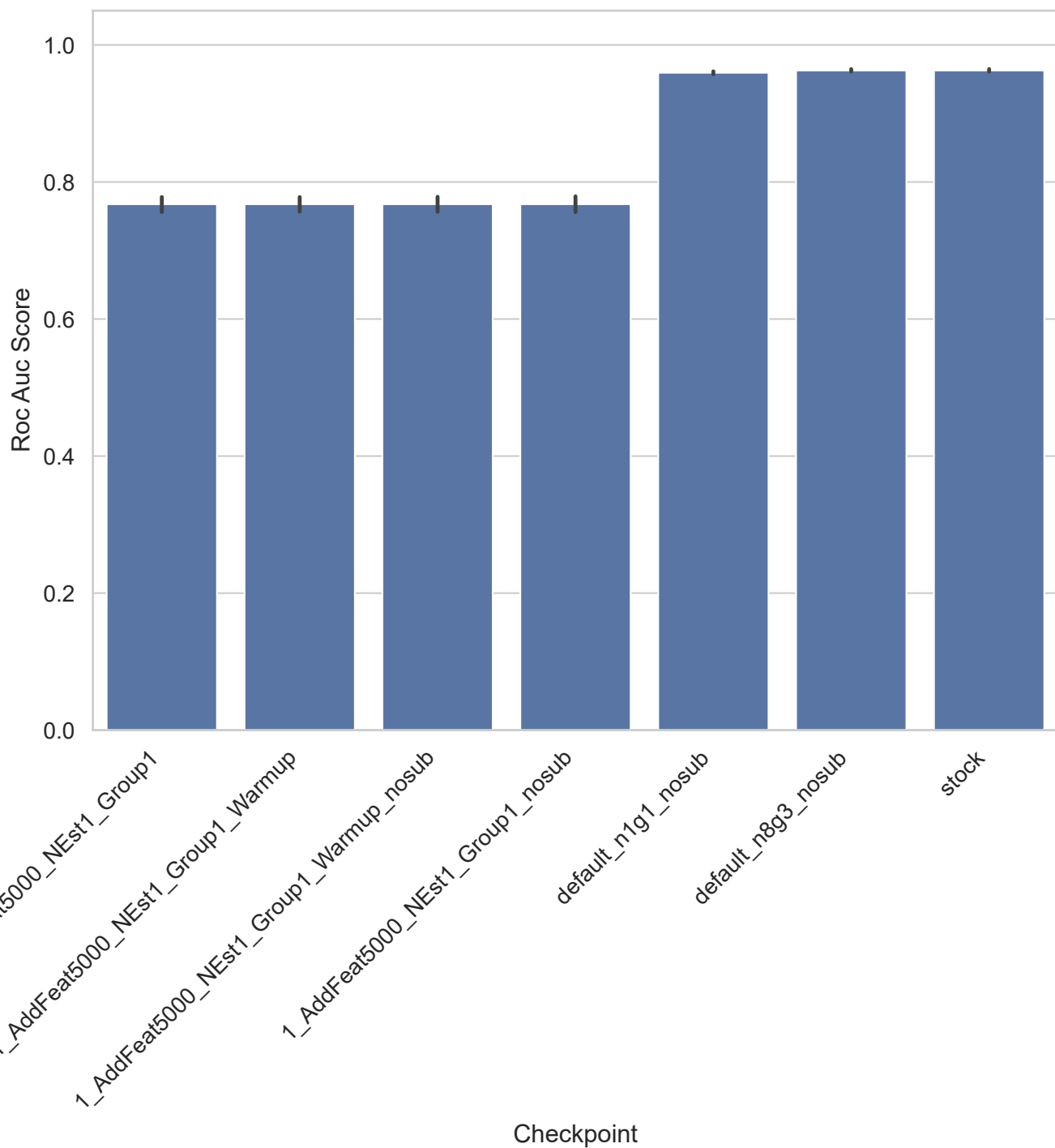
madelon - Roc Auc Score
