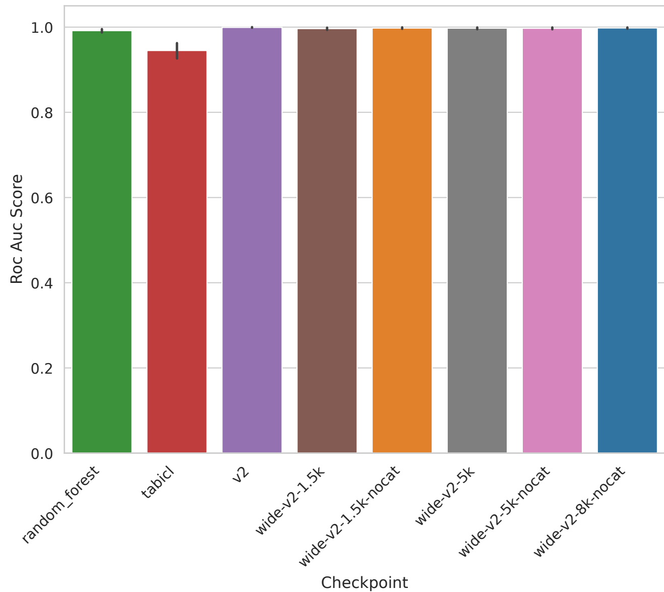
leukemia - Roc Auc Score
