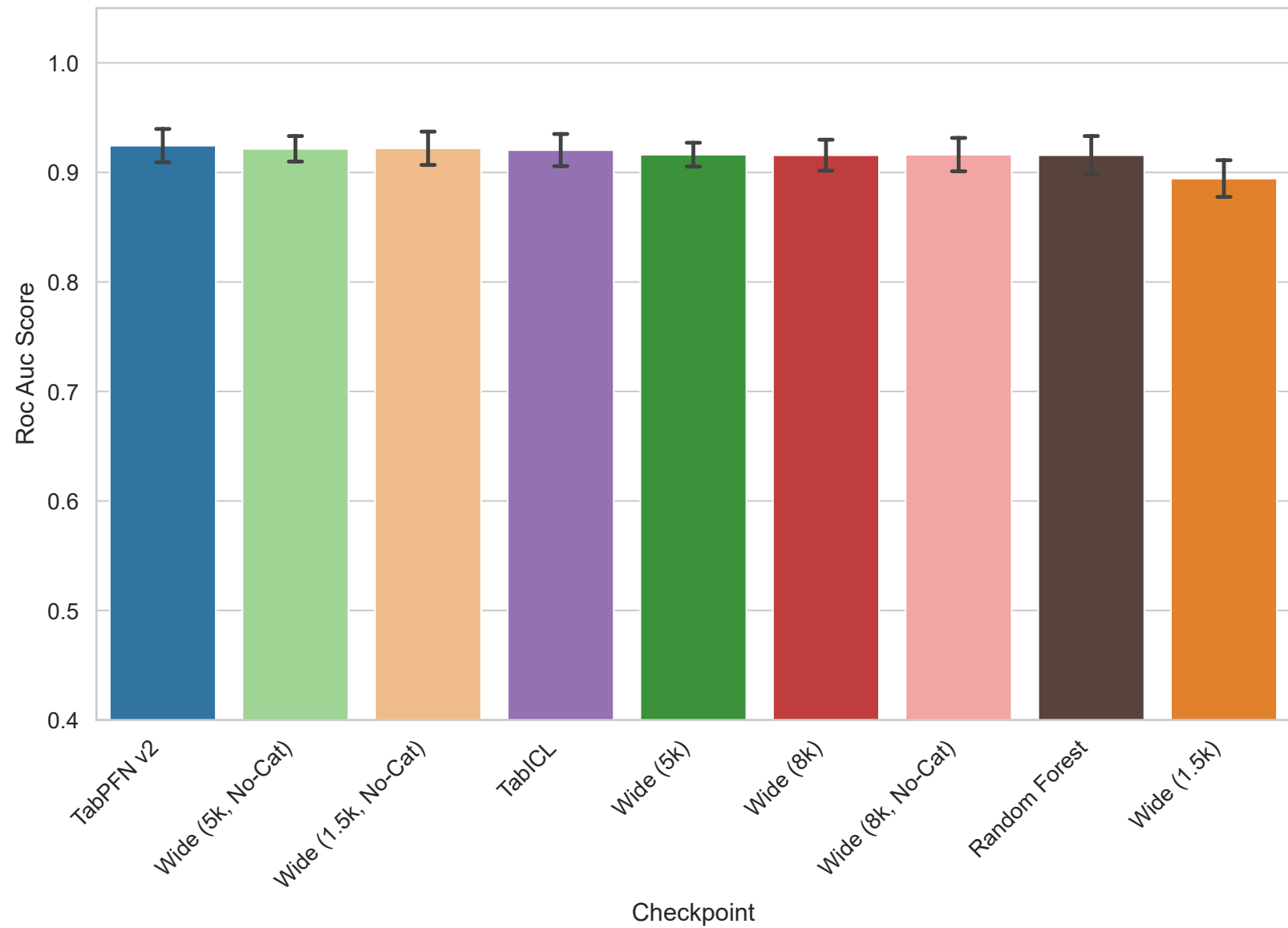
Task 363623 - Roc Auc Score
