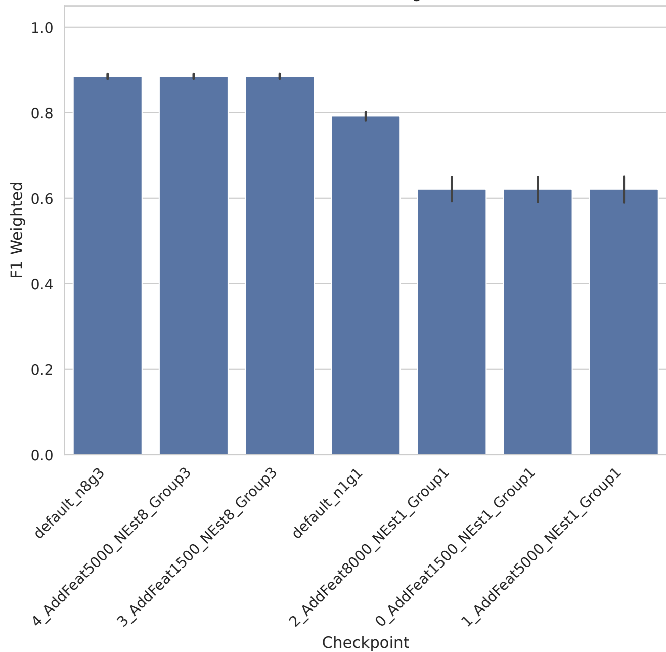
RELATHE - F1 Weighted
