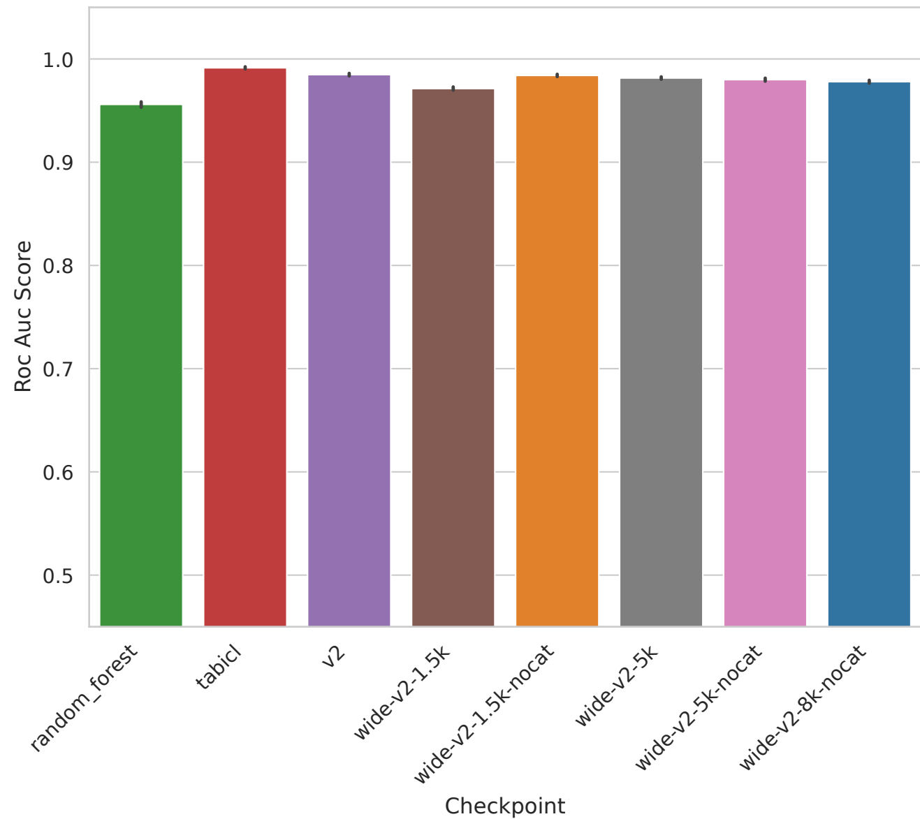
Task 363674 - Roc Auc Score
