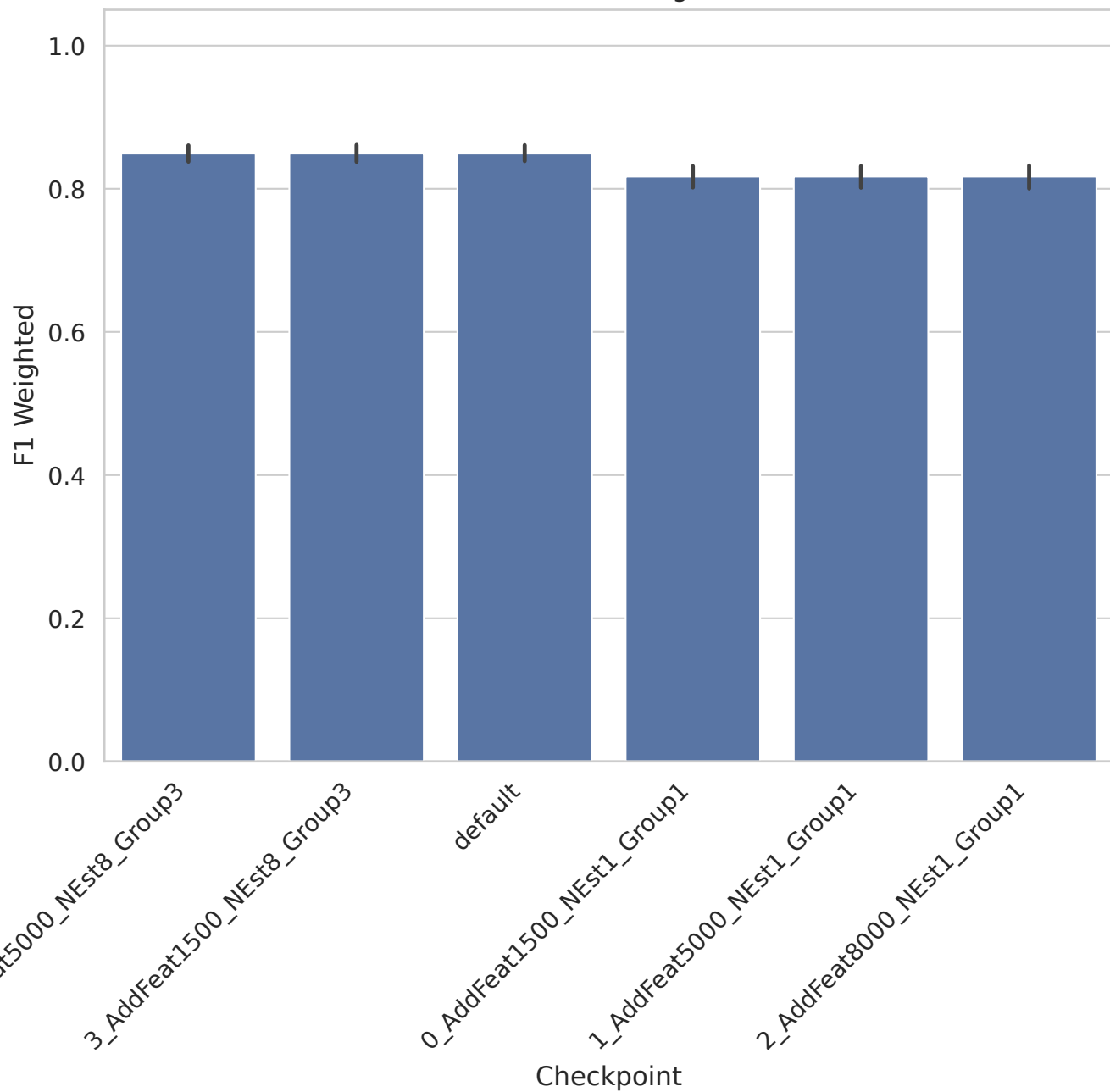
arcene - F1 Weighted
