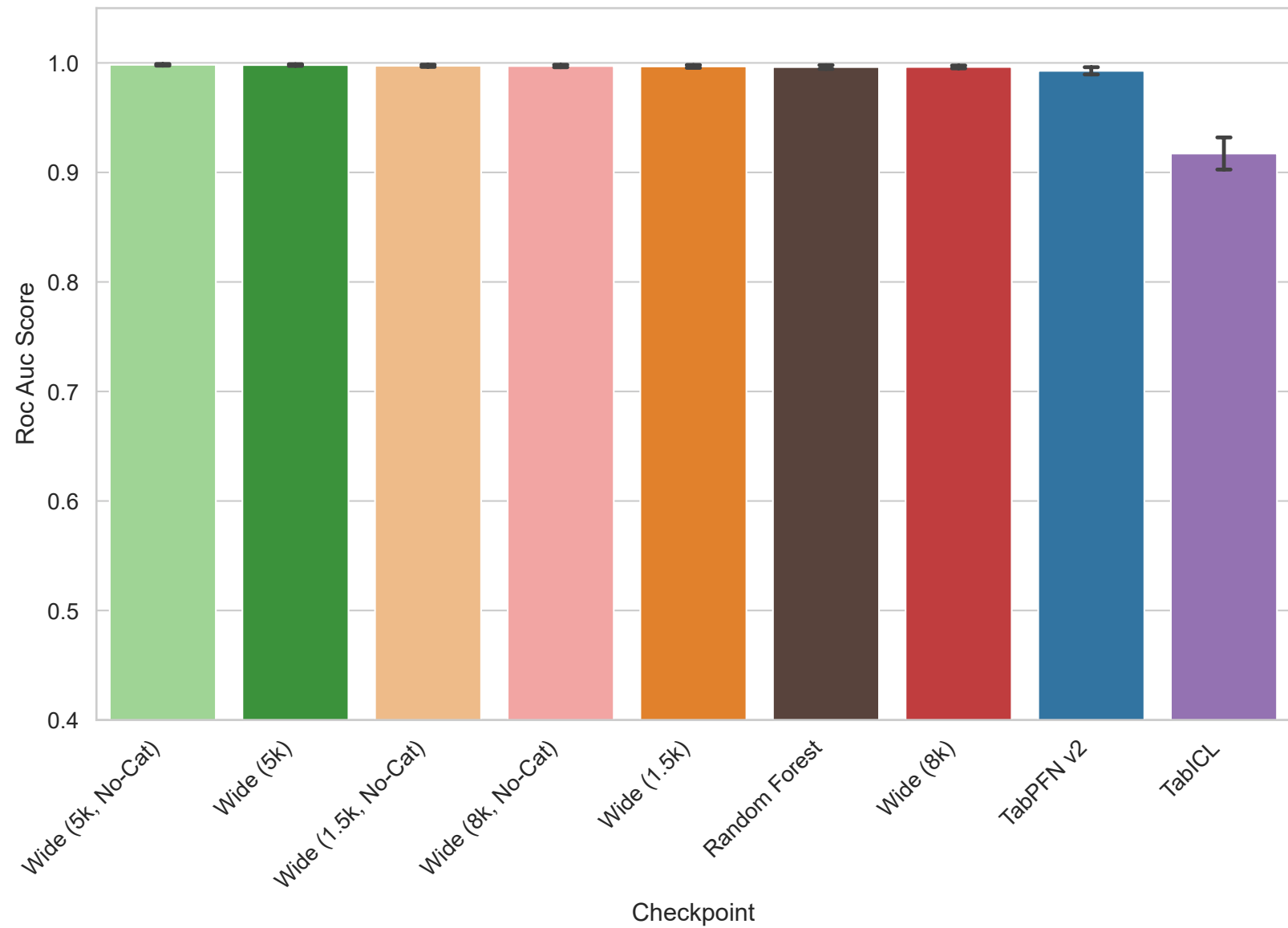
BASEHOCK - Roc Auc Score
