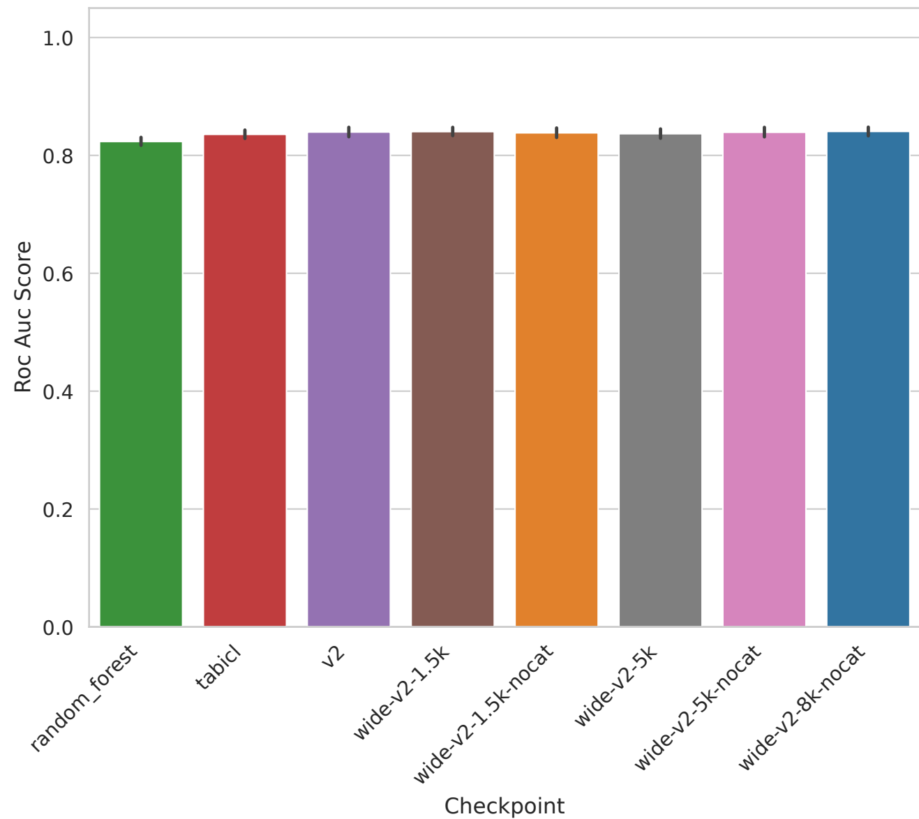
Task 363629 - Roc Auc Score
