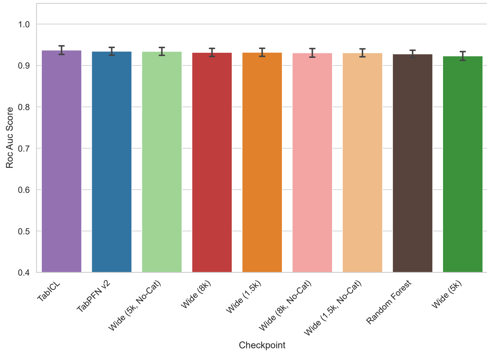
Task 363696 - Roc Auc Score
