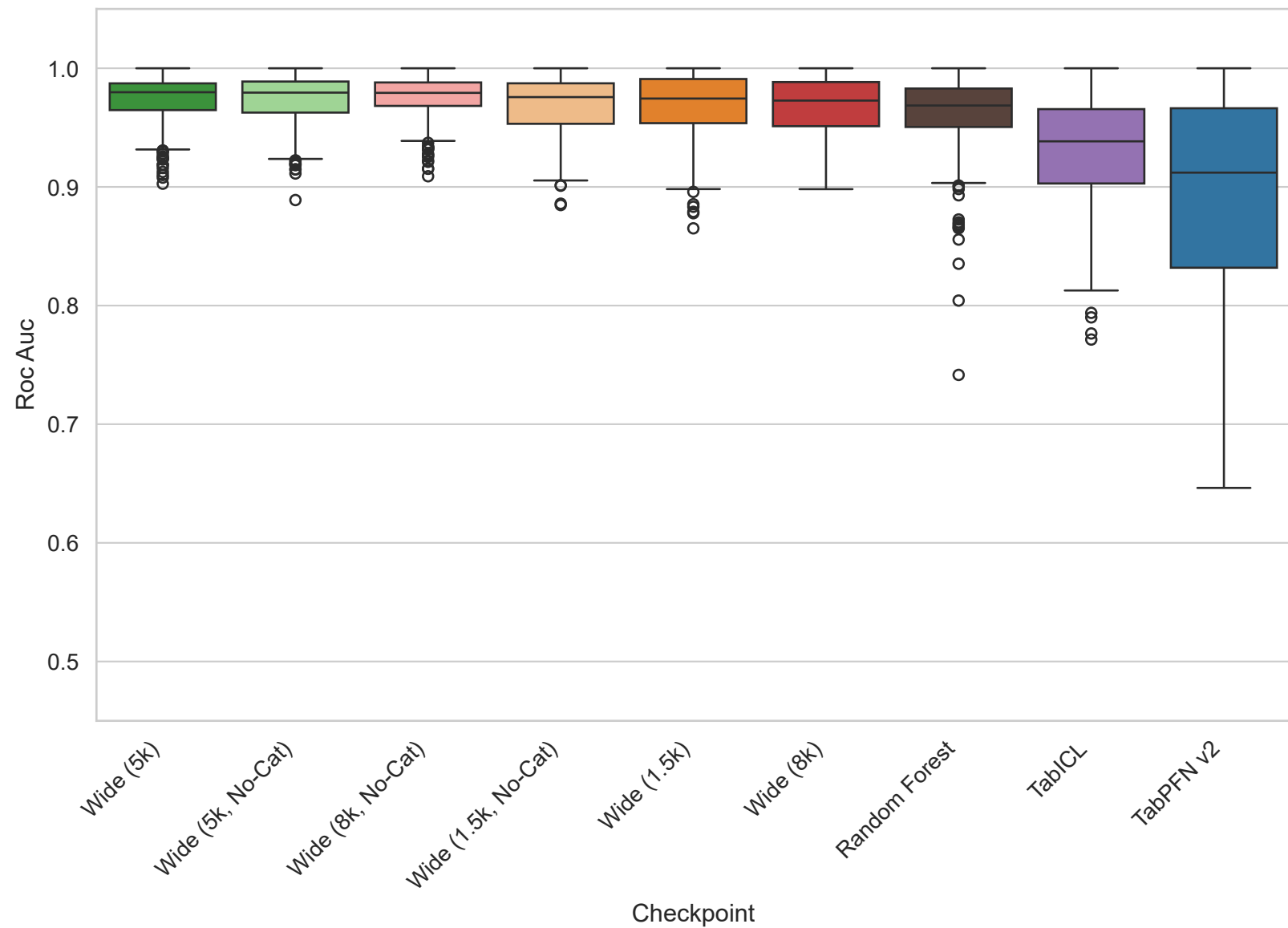
Multiomics Overview - Roc Auc Distribution
