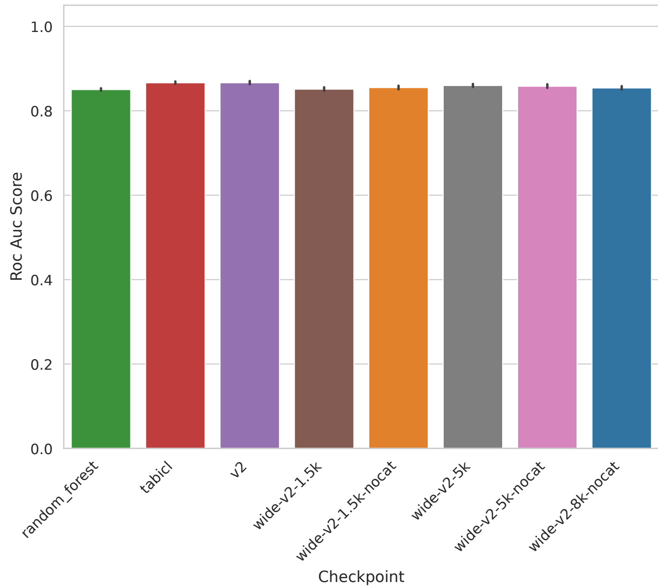
Task 363619 - Roc Auc Score
