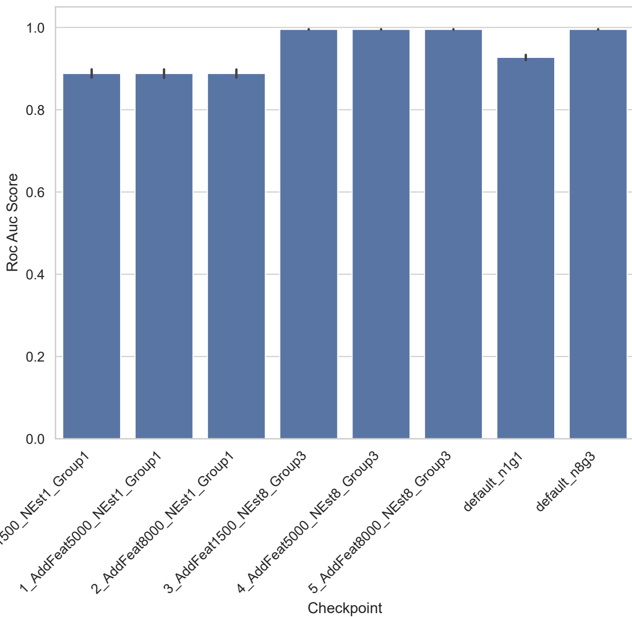
BASEHOCK - Roc Auc Score
