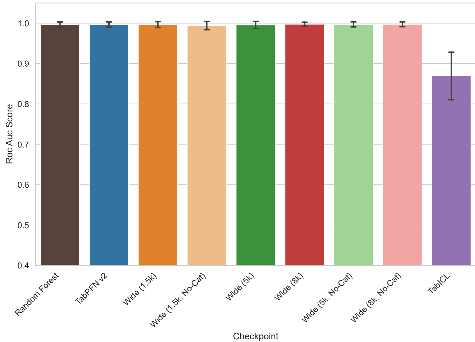
ALLAML - Roc Auc Score
