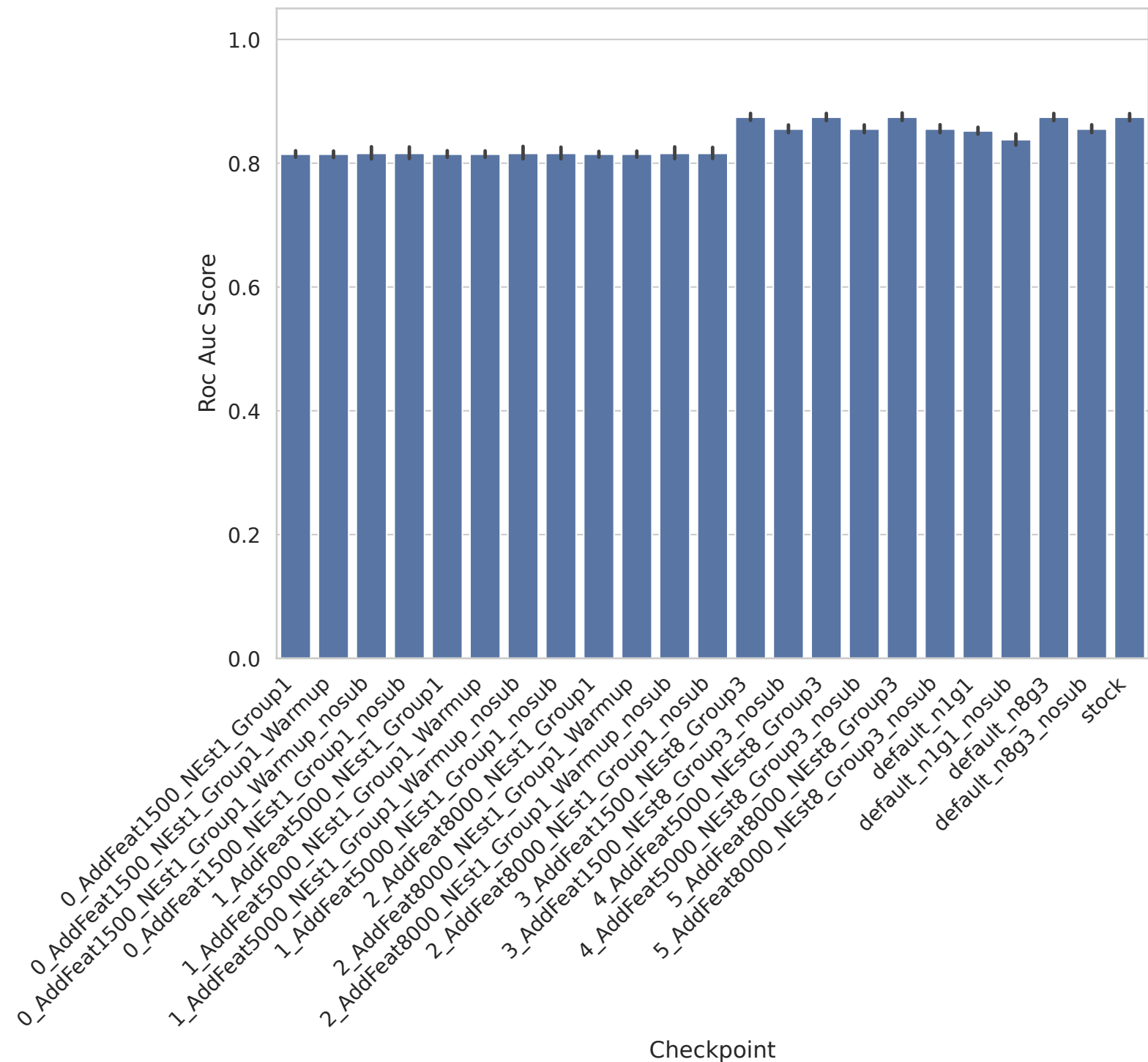
Task 363620 - Roc Auc Score
