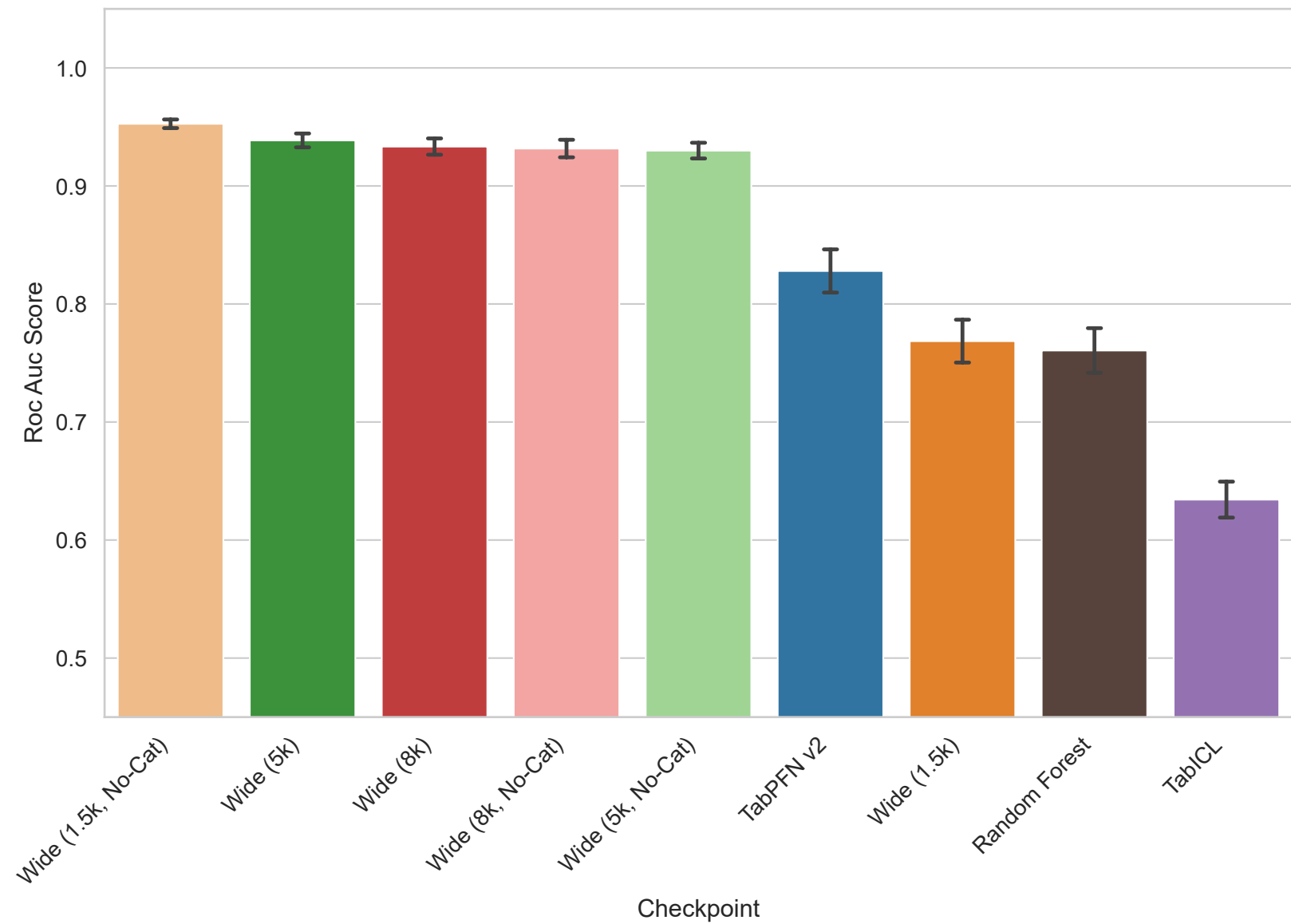
madelon - Roc Auc Score
