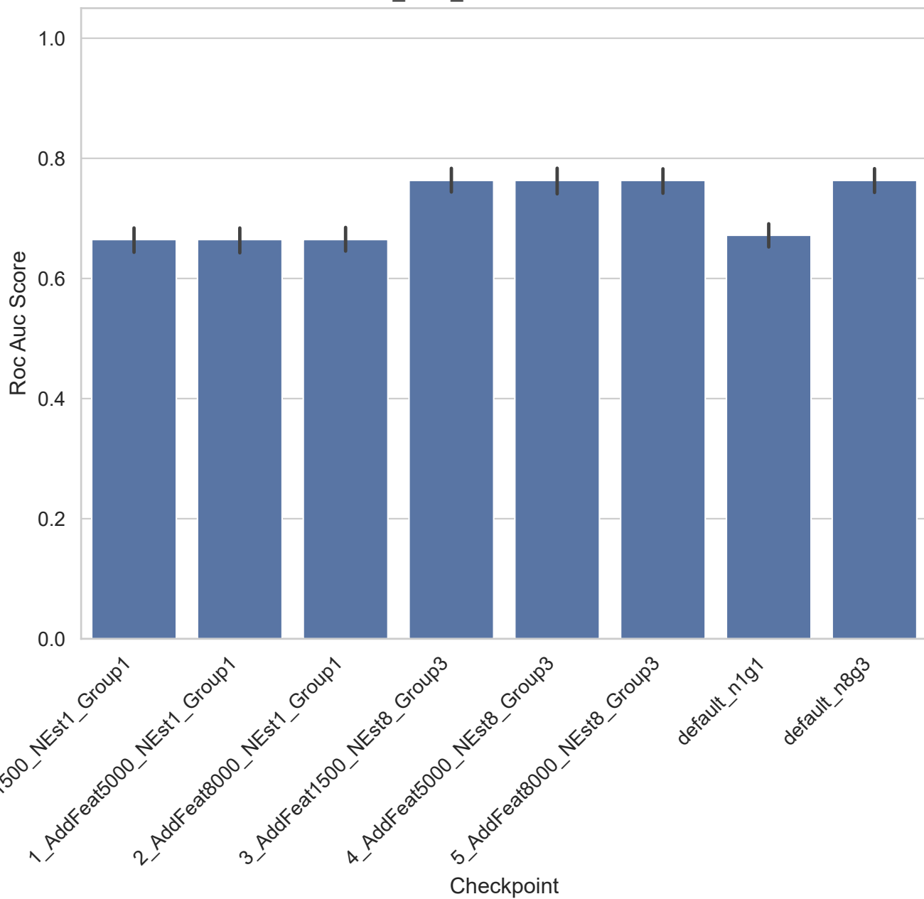
SMK_CAN_187 - Roc Auc Score
