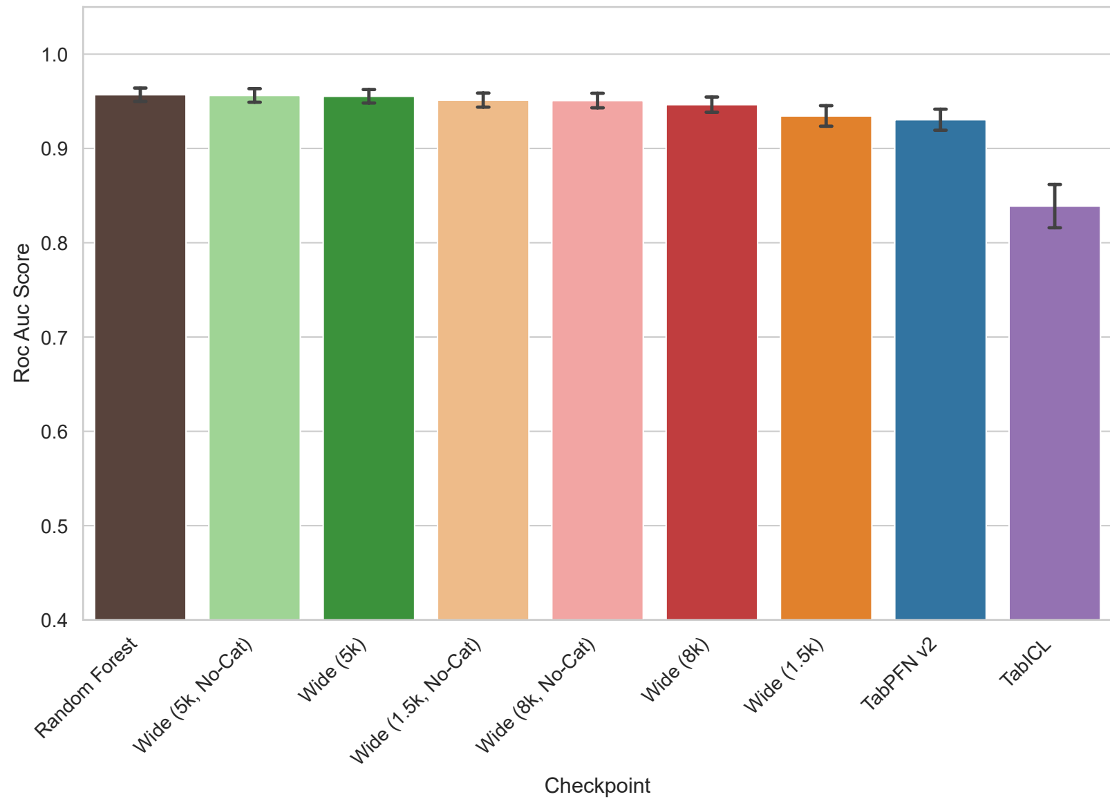
RELATHE - Roc Auc Score
