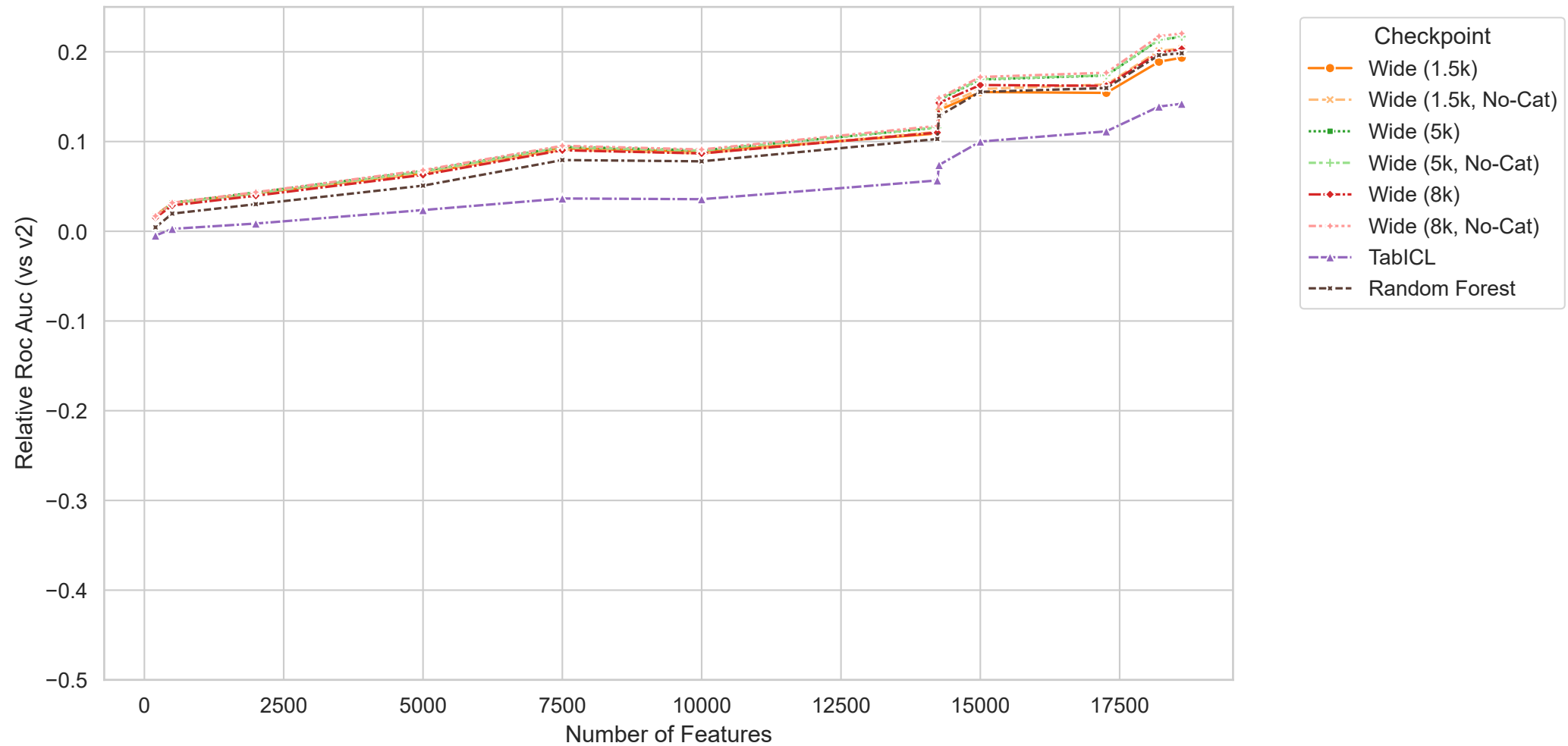
Multiomics Overview - Relative Roc Auc
