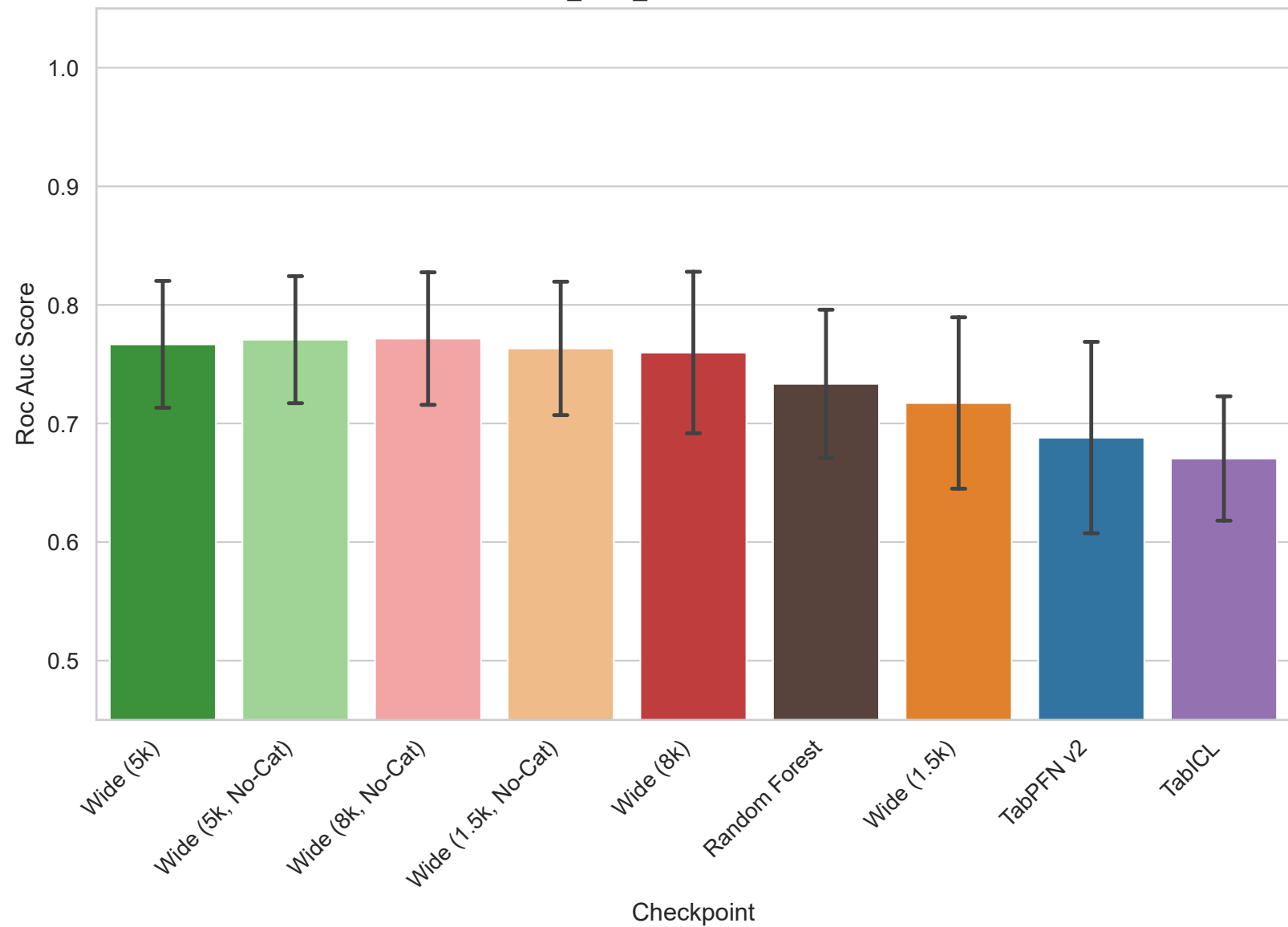
SMK_CAN_187 - Roc Auc Score
