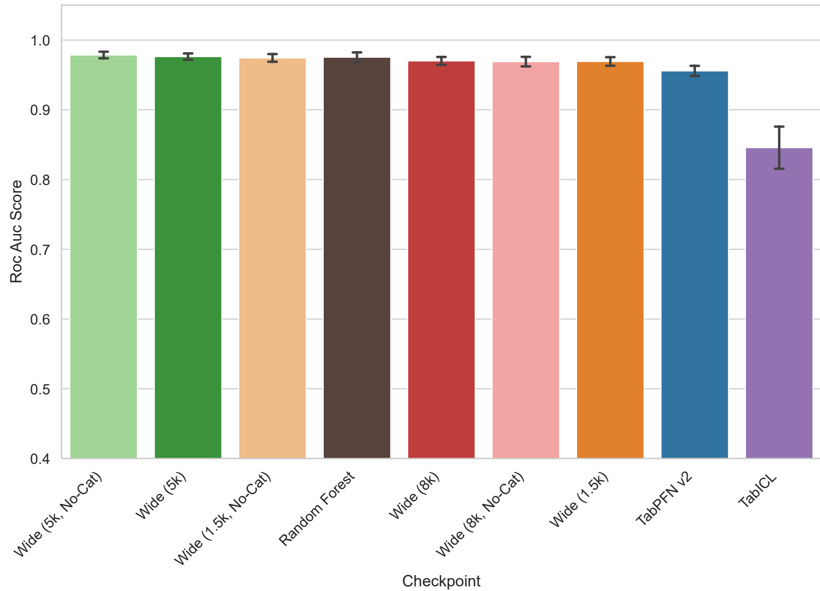
PCMAC - Roc Auc Score
