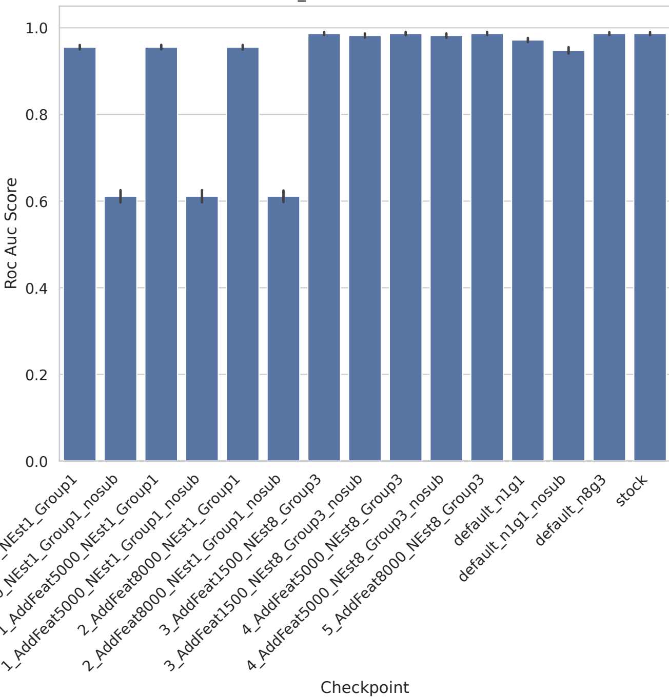
TOX_171 - Roc Auc Score
