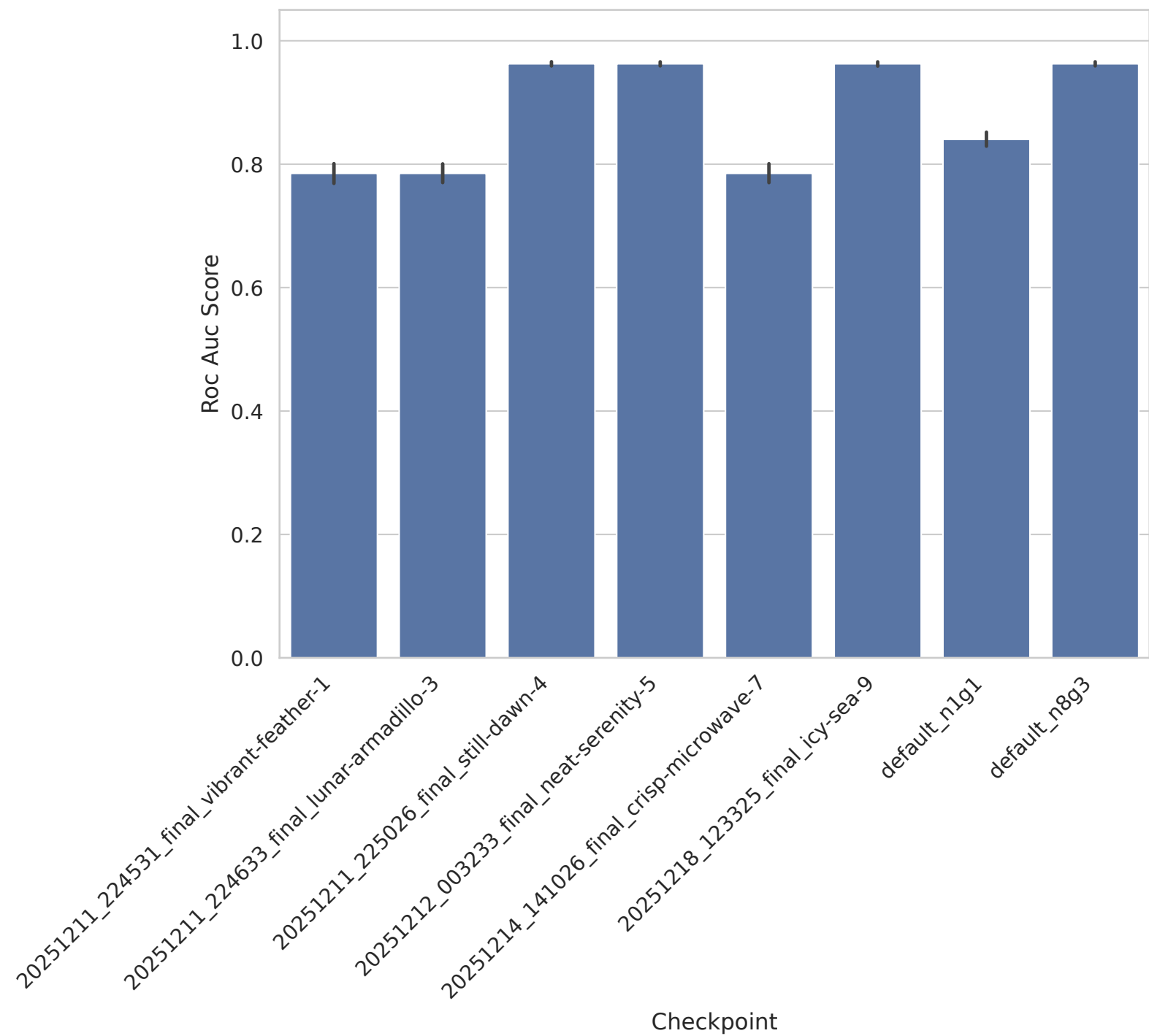
PCMAC - Roc Auc Score
