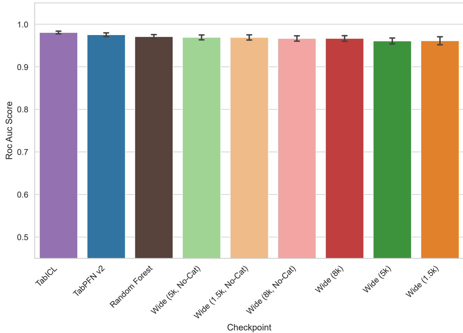
Task 363707 - Roc Auc Score
