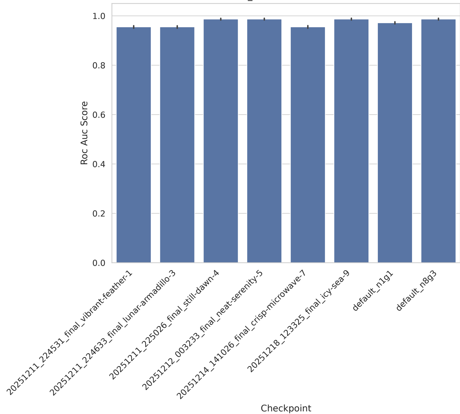
TOX_171 - Roc Auc Score
