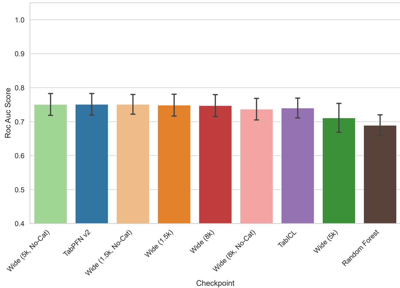
Task 363621 - Roc Auc Score
