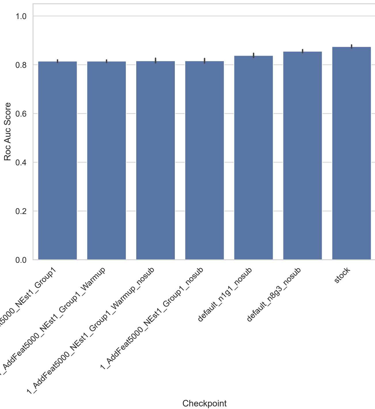
Task 363620 - Roc Auc Score
