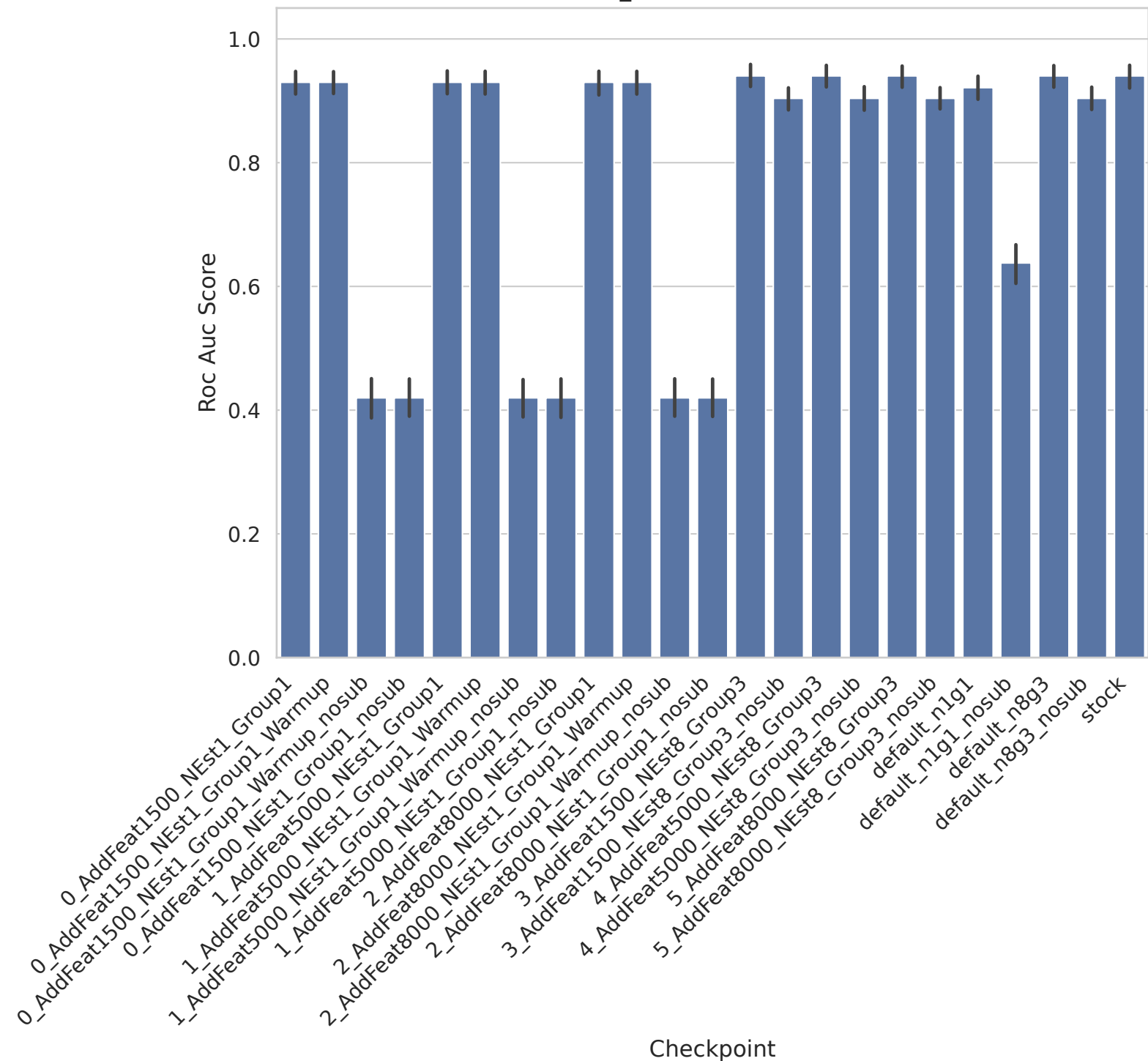
GLI_85 - Roc Auc Score
