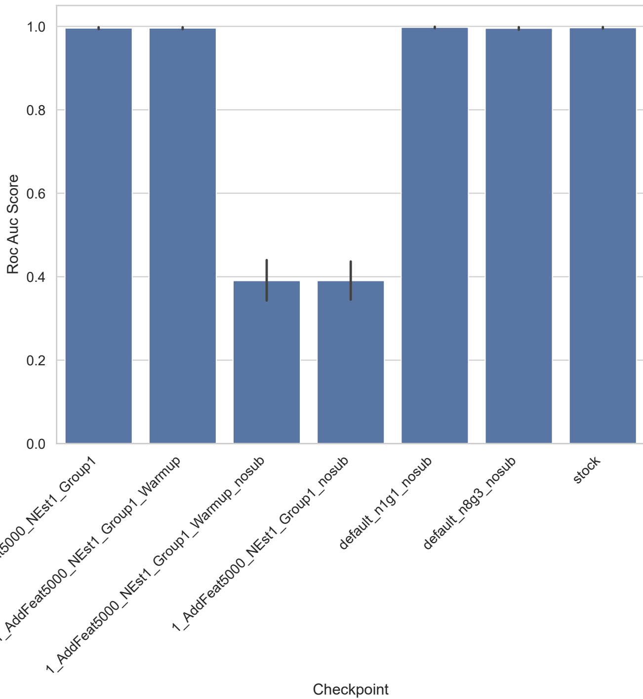
ALLAML - Roc Auc Score
