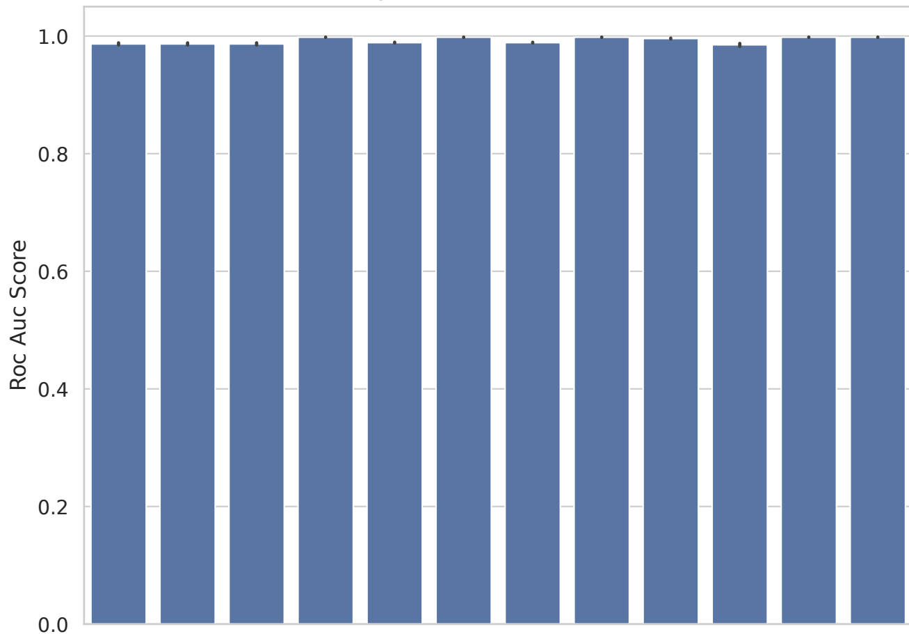
gisette - Roc Auc Score
