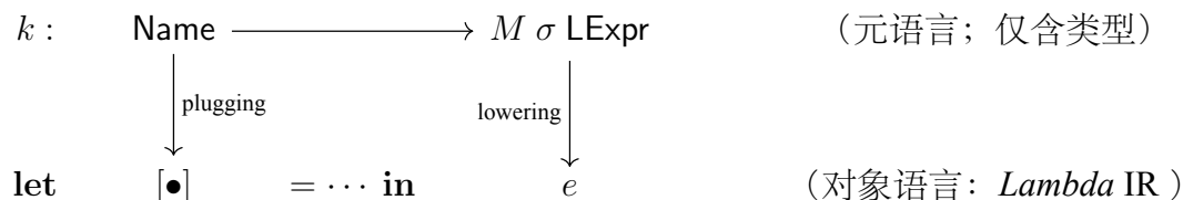
图 4.3 CPS 化在元语言与对象语言间的同态
