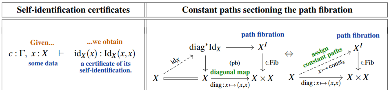
图 6.1 恒等类型的引入规则（introduction rule）在范畴论上的意义 [51]
