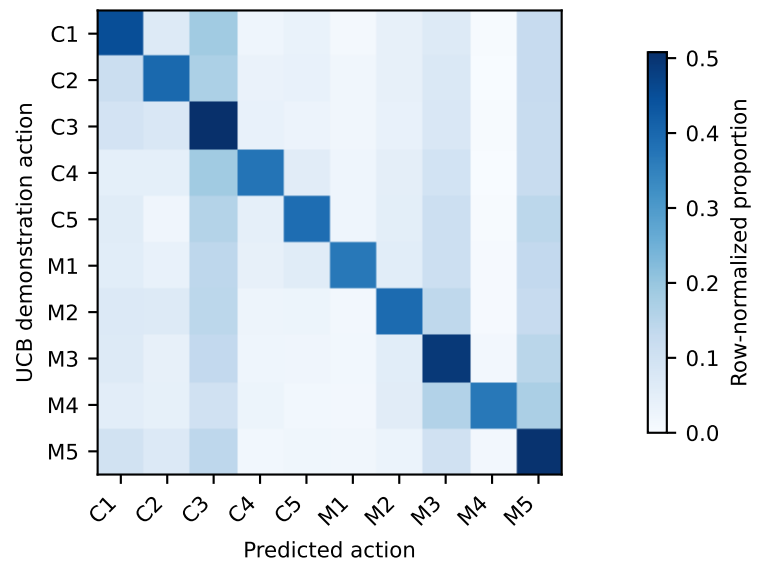
(d) Enhanced-state confusion
