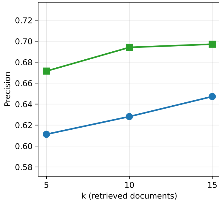
Precision
