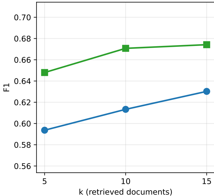
F1
