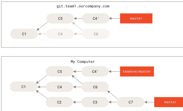
شكل ٤٦. شخص يدفع إيداعات معاد تأسيسها، هاجراً بذلك الإيداعات التي بنيت عليها عملك
