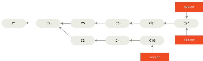
شكل ٤١. تسريع الفرع الرئيس لضم تعديلات فرع client
