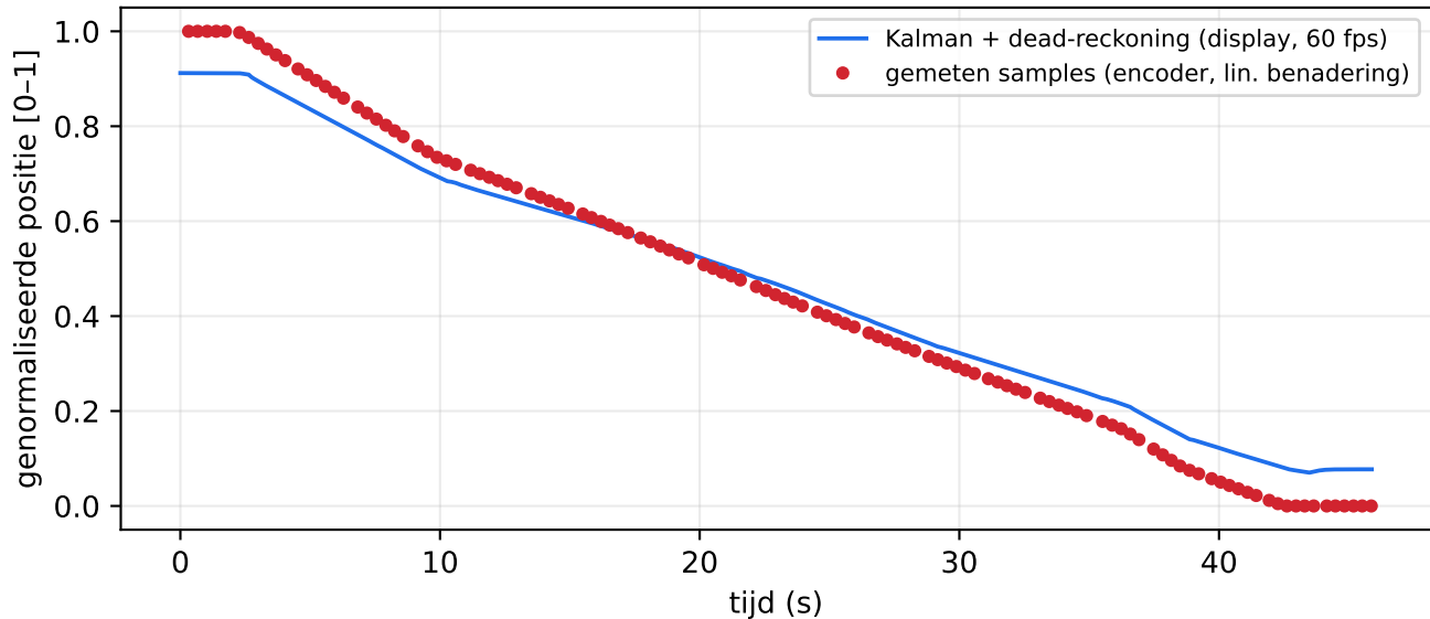
Positie over tijd: gemeten samples vs. Kalman/dead-reckoning
