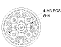
밑면 · 고정부
