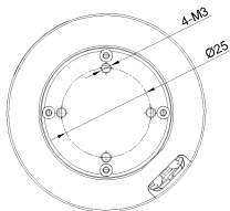
윗면 · 프로펠러 쪽
