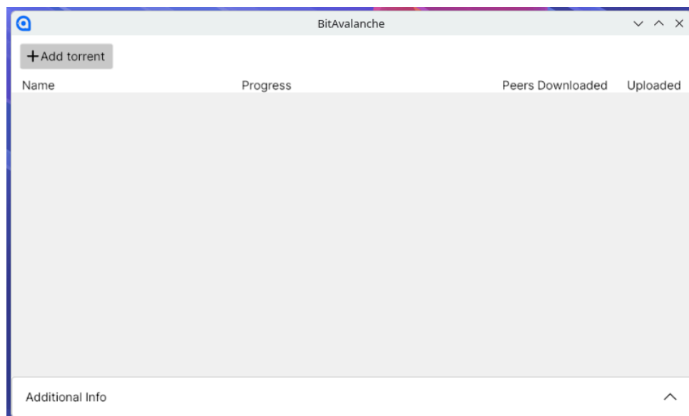
Figura 1: Spuštěný program
