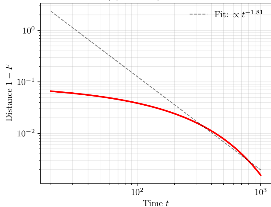
(d) Convergence Rate
