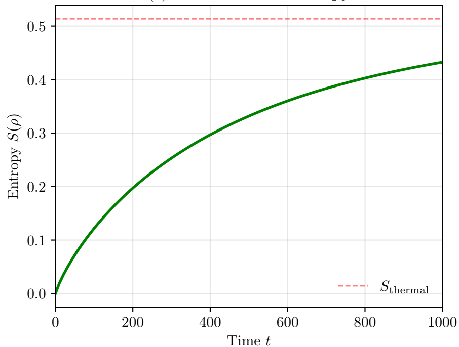
(c) Von Neumann Entropy
