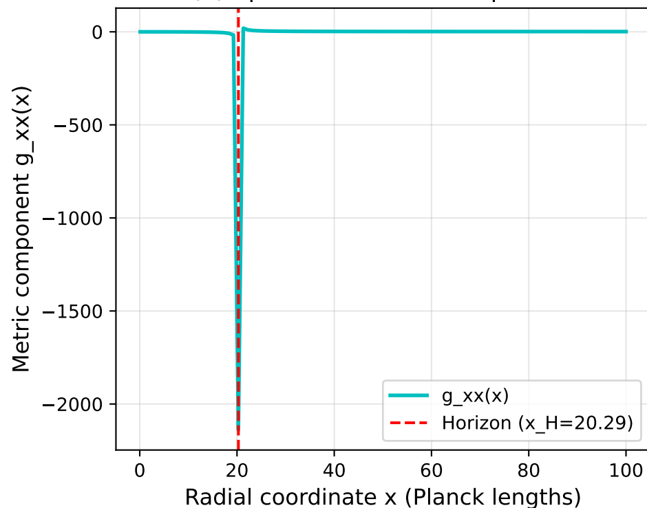
(d) Spacelike Metric Component
