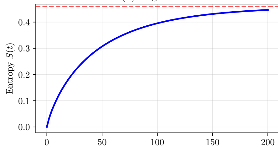
(d) Detailed Balance
