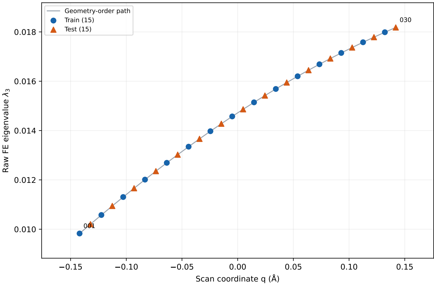
BeH2 · column 3 · active FE vs geometry
