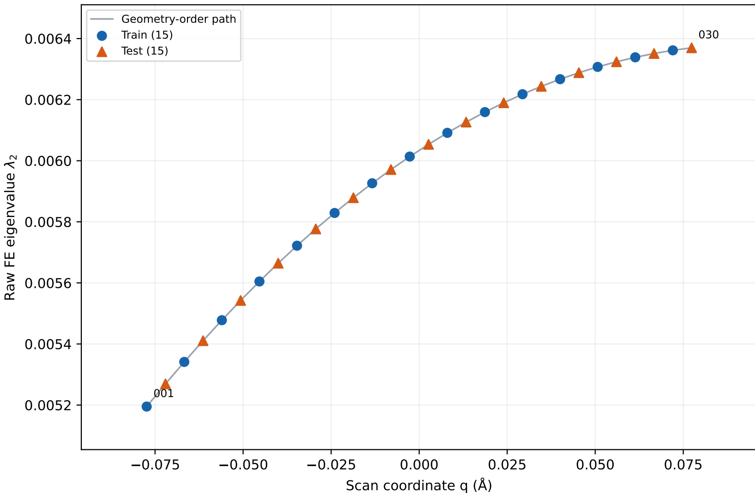
CO · column 2 · active FE vs geometry
