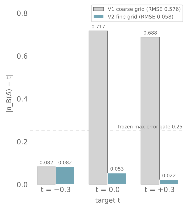
(c) per-target error: V1 vs V2
