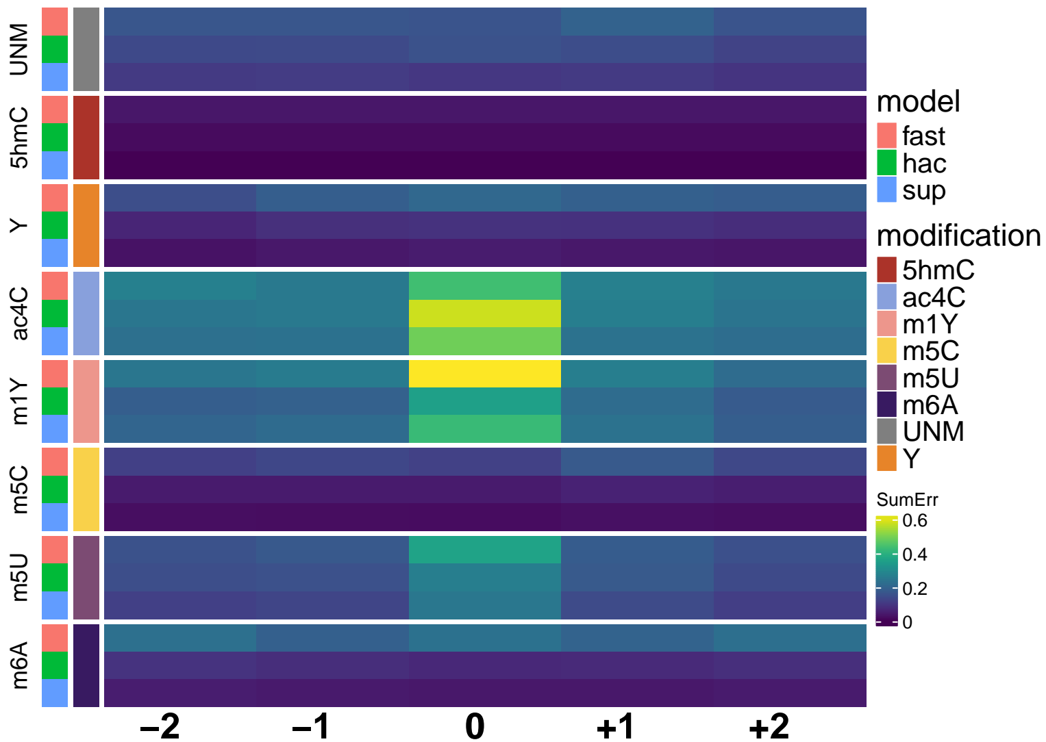
SumErr
