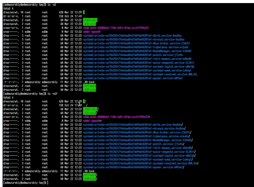
Рис. 4.2: Использование команды ls
