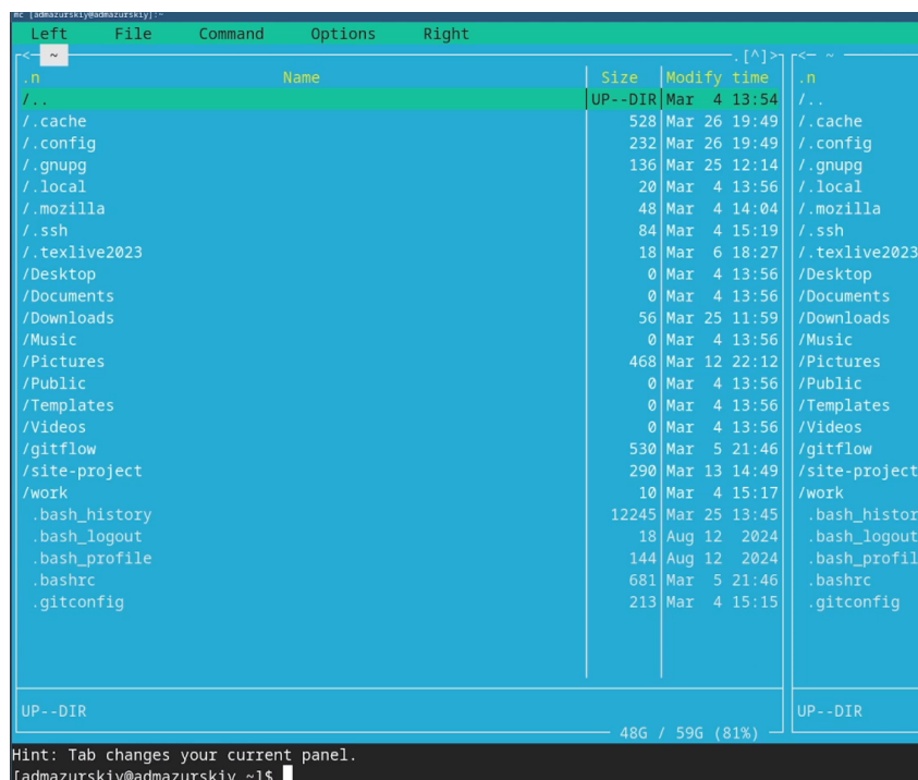
Рис. 4.2: Интерфейс mc
