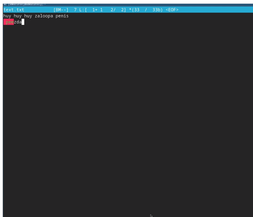
Рис. 4.3: Редактор mc
