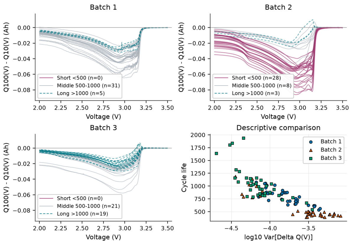
그림 3. Delta Q(V)는 같은 전압에서 100사이클 용량에서 10사이클 용량을 뺀 값입니다. 곡선은 수명 그룹별로, 산점도는 배치별로 색과 모양을 구분했습니다.
