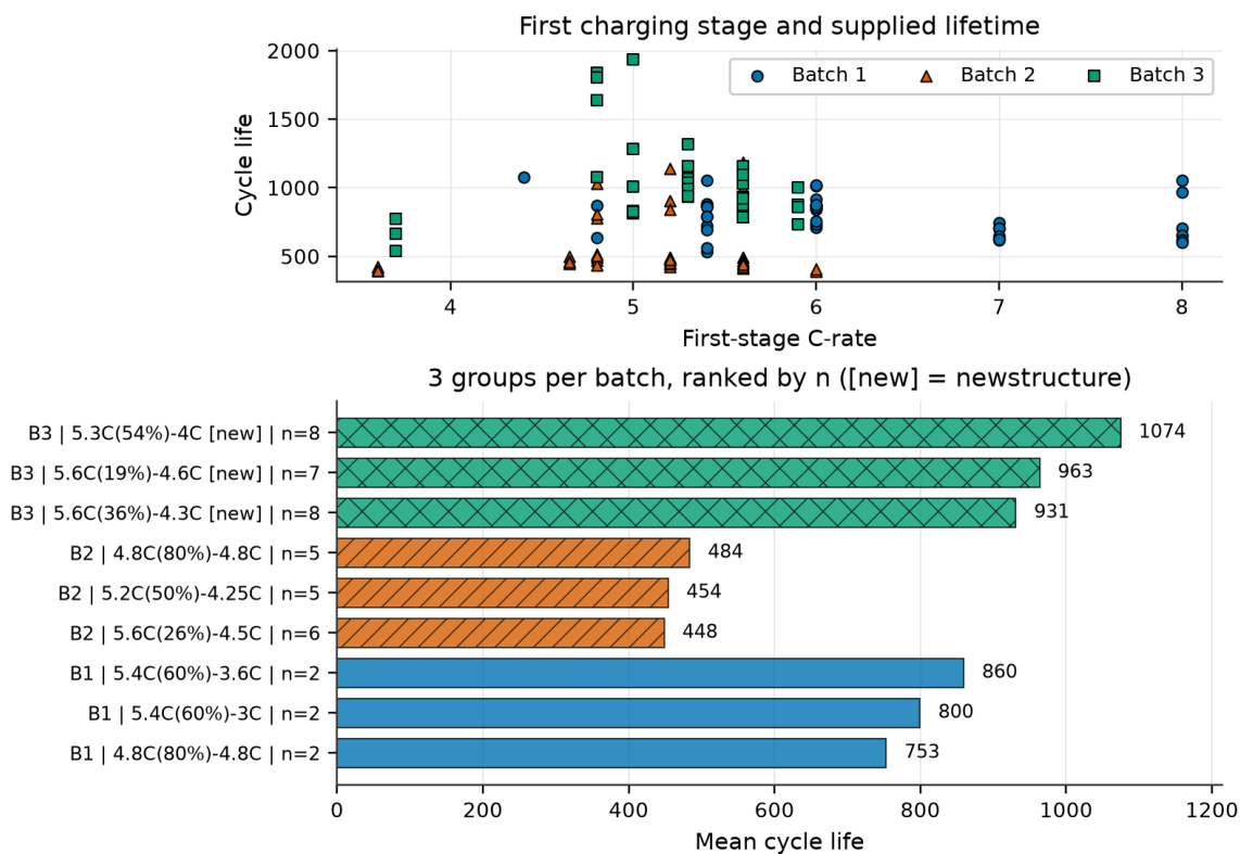
그림 4. 첫 충전 단계의 C-rate와 수명, 배치별 주요 충전 방식의 평균 수명을 비교했습니다. 셀 개수가 많은 방식 3개씩을 골랐고, 개수가 같으면 이름순으로 정렬했습니다(n은 셀 개수입니다).
