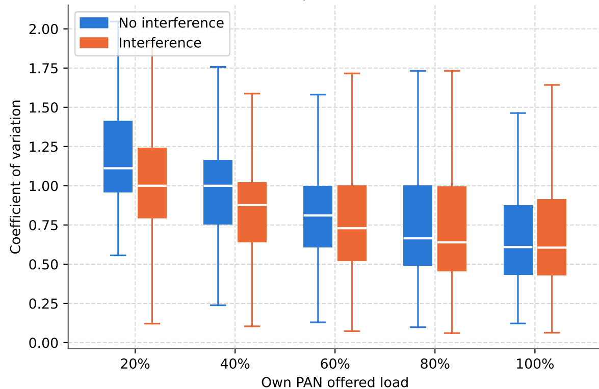
Uplink (UL)
