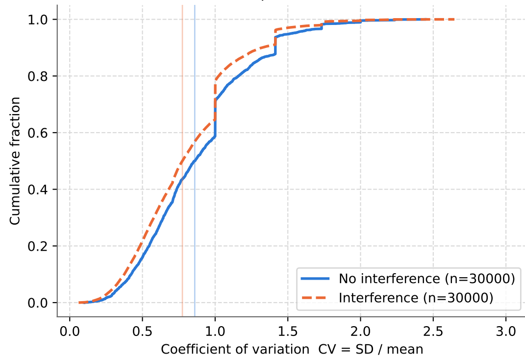
Uplink (UL)
