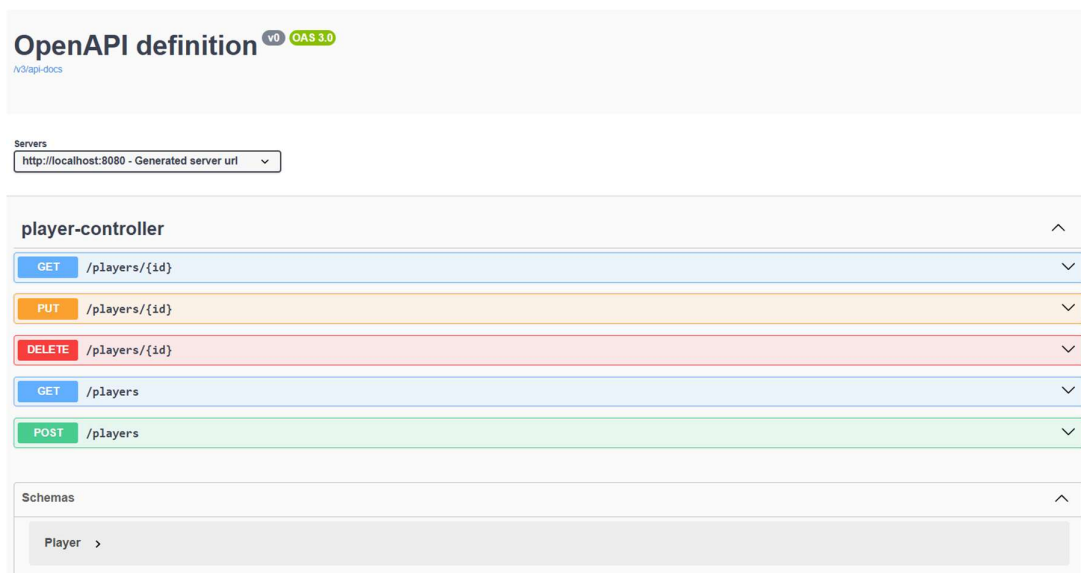
Hình Liệt kê danh sách các RESTful API có trong ứng dụng sử dụng Swagger-UI
