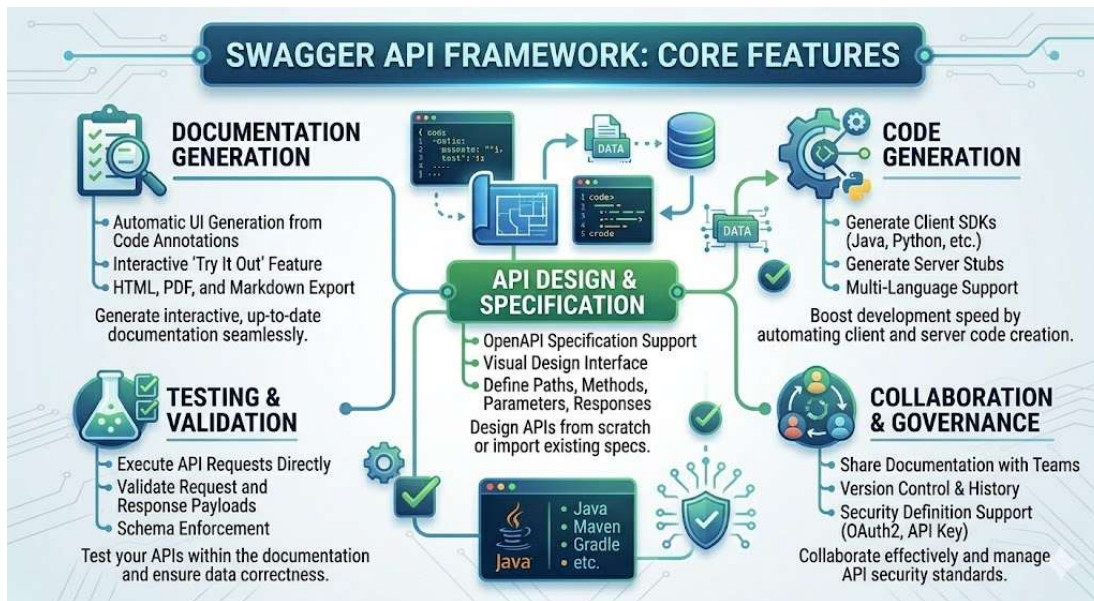
Hình Các tính năng quan trọng của SWAGGER
