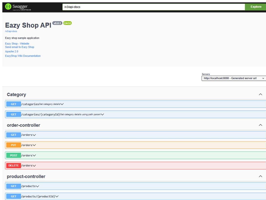
Hình Liệt kê danh sách các Endpoint có trong ứng dụng bằng Swagger UI
