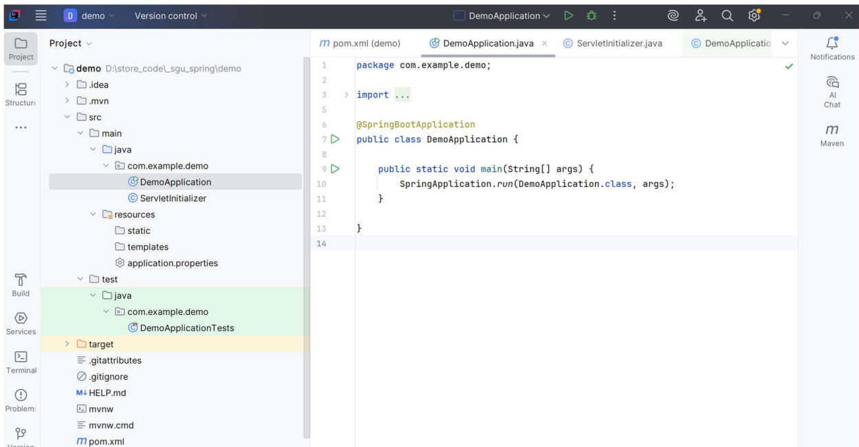
Hình Dự án Spring boot khi được mở bằng ứng dụng IntelliJ Community
