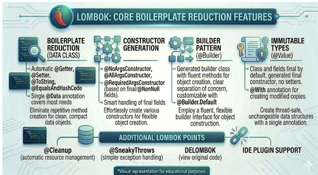
Hình Tổng quan các tính năng của Lombok
