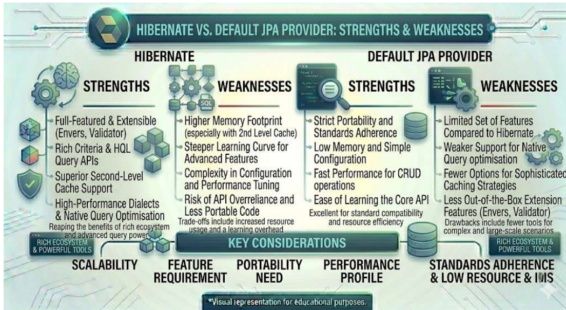
Hình So sánh giữa Hibernate và cài đặt JPA mặc định
