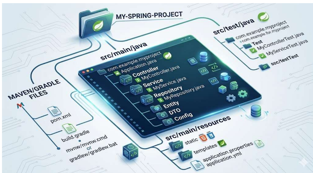
Hình Cấu trúc dự án Spring Project với Spring Boot
