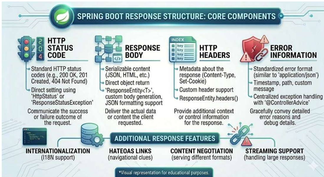
Hình Hỗ trợ các Response có trong Spring Boot
