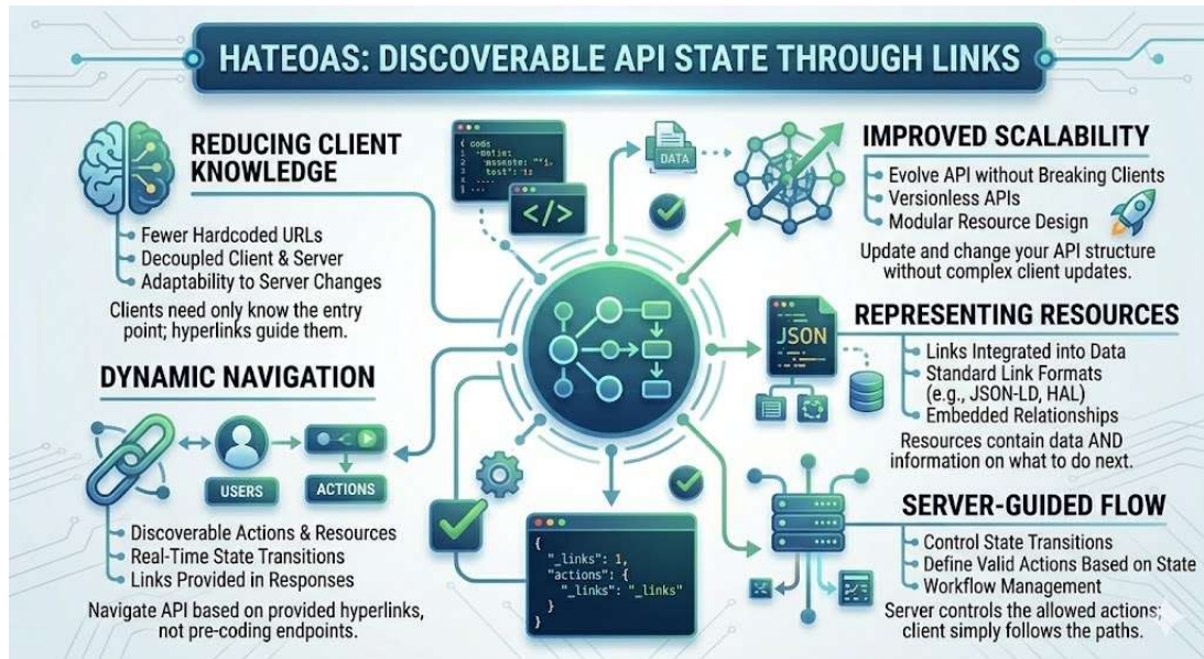
Hình Các tính năng chính HATEOAS
