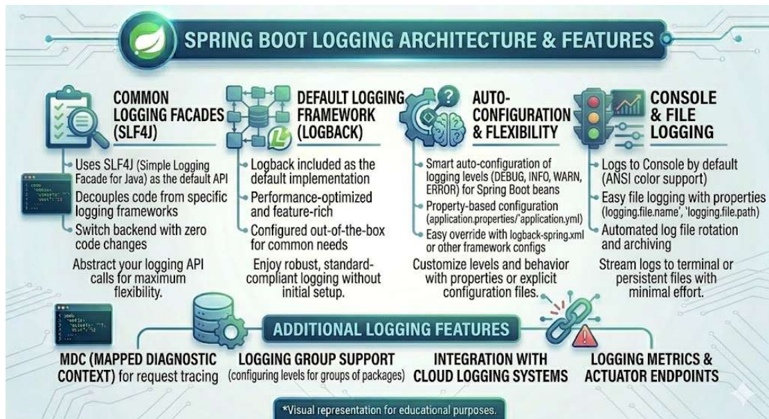
Hình Tổng quan xử lý Logging mà Spring hỗ trợ
