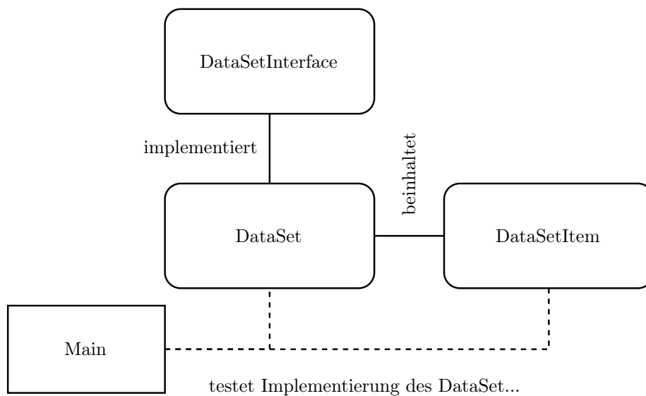
Figure 1: Abbildung 1: Darstellung der Klassenbeziehungen.
