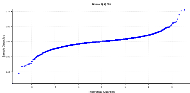
Fig. 21.3: Quantile-Quantile plot.
