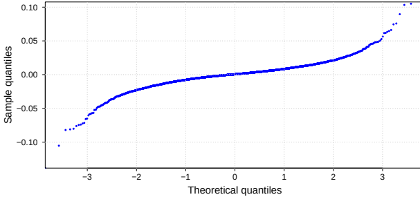
Fig. 1.19: Quantile-Quantile plot.
