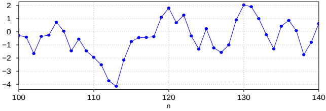
Fig. 2.2: AR(2) Samples.
