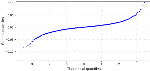
Fig. 1.19: Quantile-Quantile plot.
