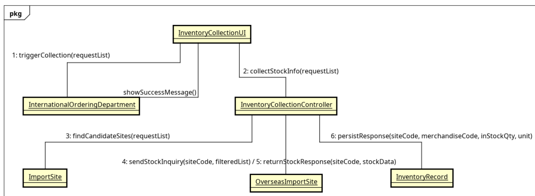
Figure 3.2: Communication diagram mức phân tích UC003 - CollectInventoryData
