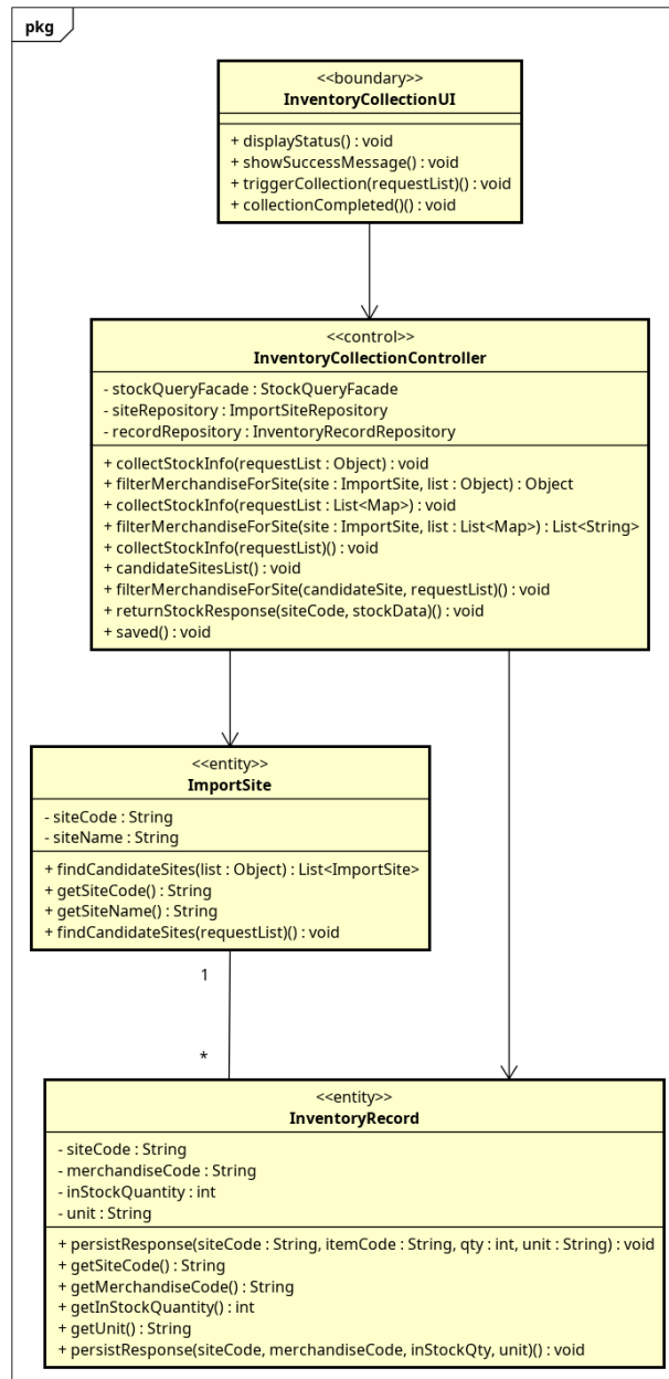
Figure 3.10: Class diagram mức phân tích UC03 - CollectInventoryData
