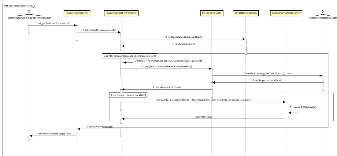
Figure 3.1: Sequence diagram mức thiết kế UC003 - CollectInventory-Data
