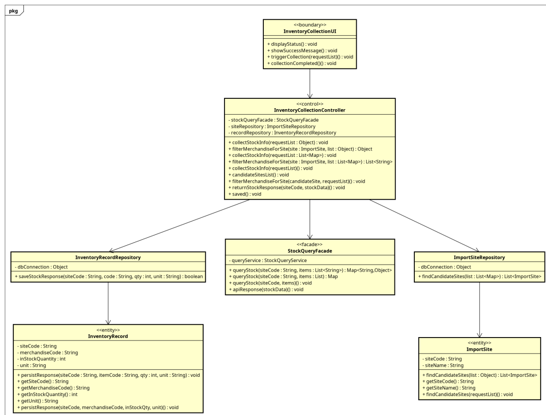
Figure 3.1: Class diagram mức thiết kế UC003 - CollectInventoryData
